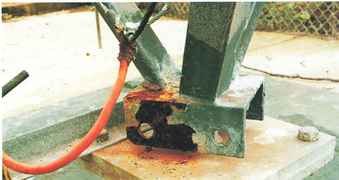
Mast base corrosion 8GO Nhulunbuy.
