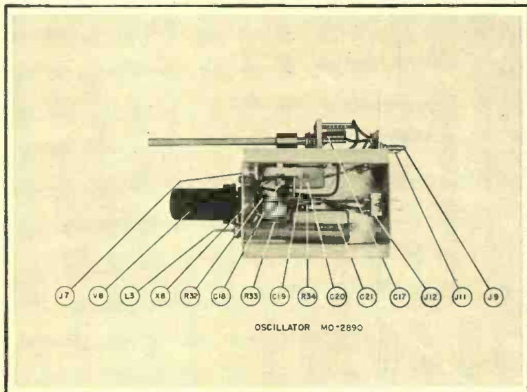
Fig. 5 - Oscillator MO2890
