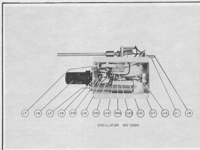
Fig. 5 - Oscillator MO2890
