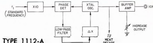
TYPE 1112-A 1, 10, 100 Mc
