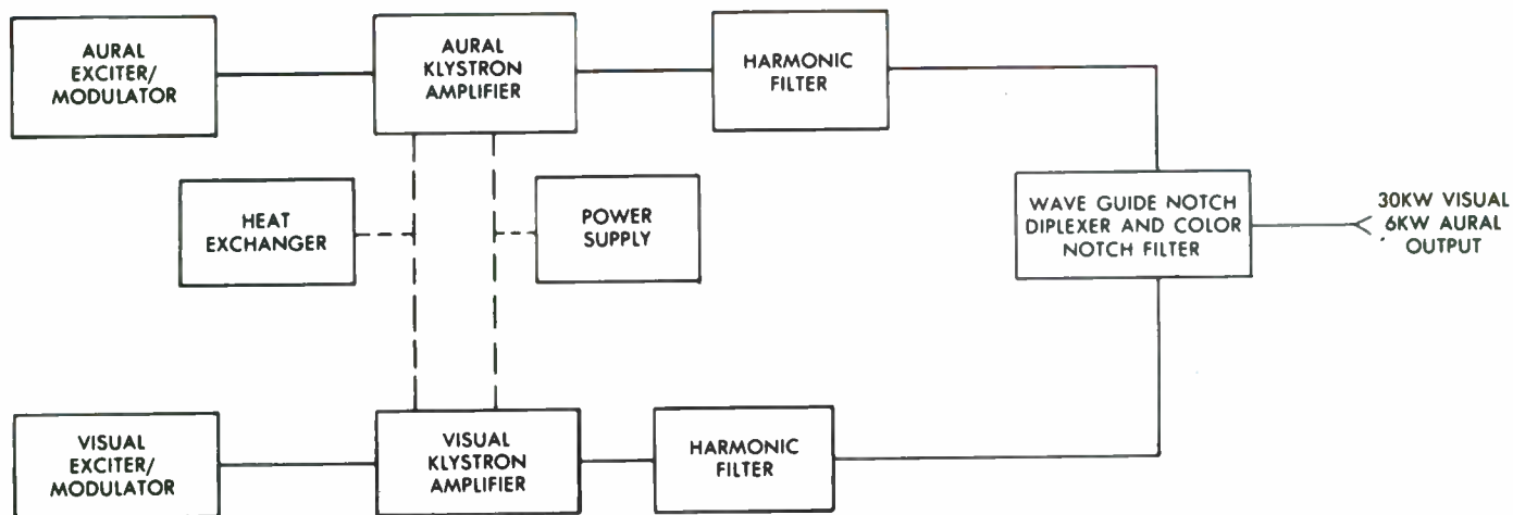
BLOCK DIAGRAM TV-30U
