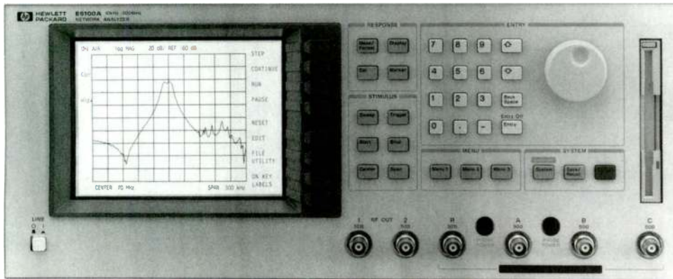
HP E5100A/B
