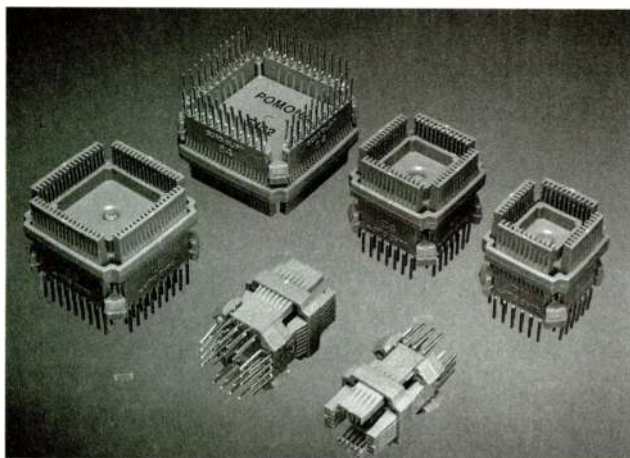
HP E2422A
