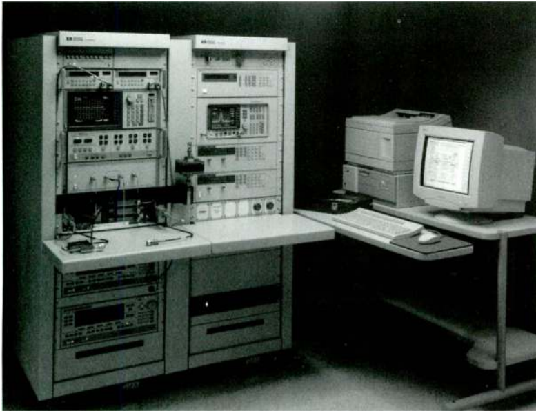
HP 85118A
