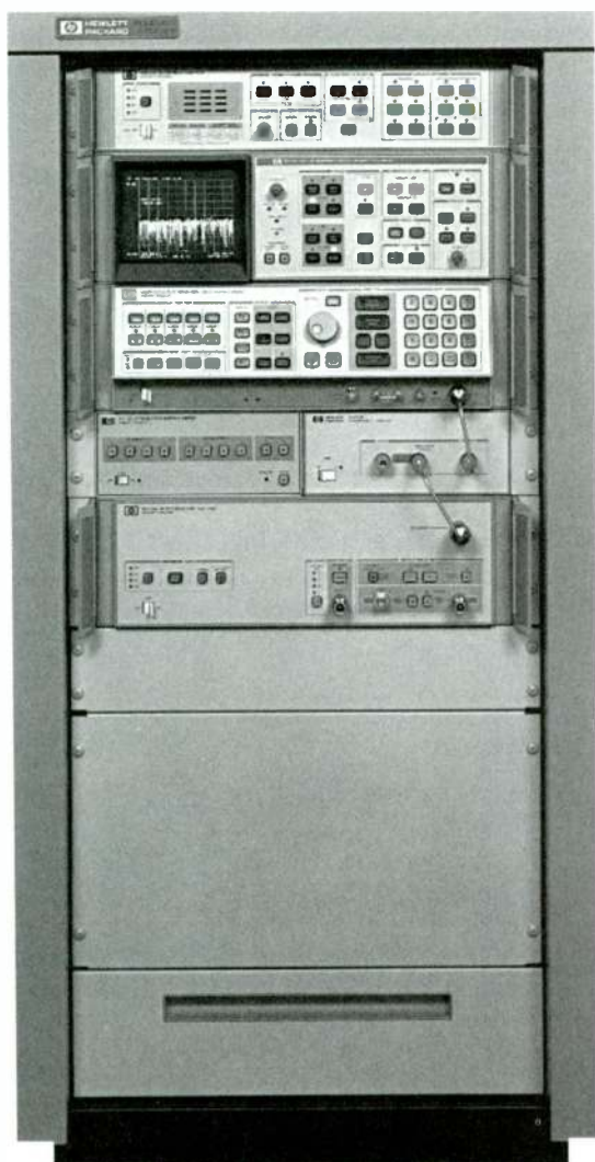
HP 8572A
