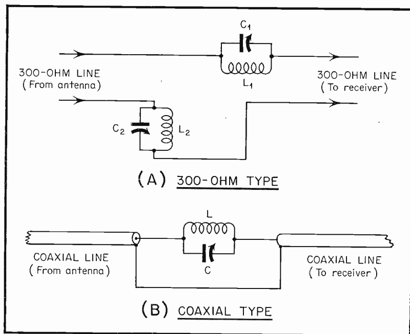
Fig. 4. Wavetrap Filters for TVI.
