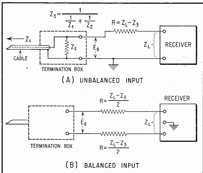
Fig. 3. Resistor-Type Dummy Antennas.
