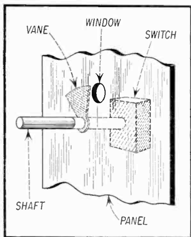
Fig. 4. Switch Flag
