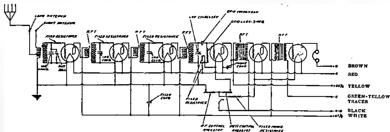
FIG. 45. WIRING DIAGRAM—MODELS 33 AND 49.
