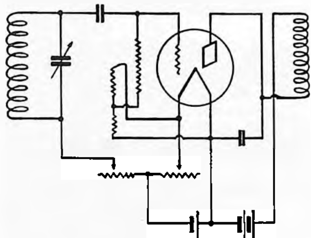
FIG. 15. DETECTOR CIRCUIT.
