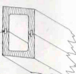
FIG. E HOLLOW BOX SPAR
