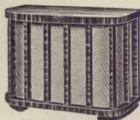
Eltrodyn 32 Elektro-dynamischer Lautspre- cher mit Fremderregung und Ab- wärts-Transformator. Klangfärber eingebaut. — Für Gleichstrom. RM 62.— Gewünschte Spannung angeben.
