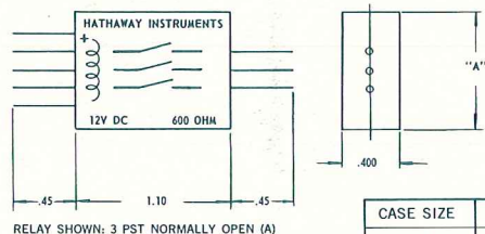
WIDTH DIMENSIONS
