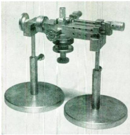
Fig. 2—Harmonic generator.
