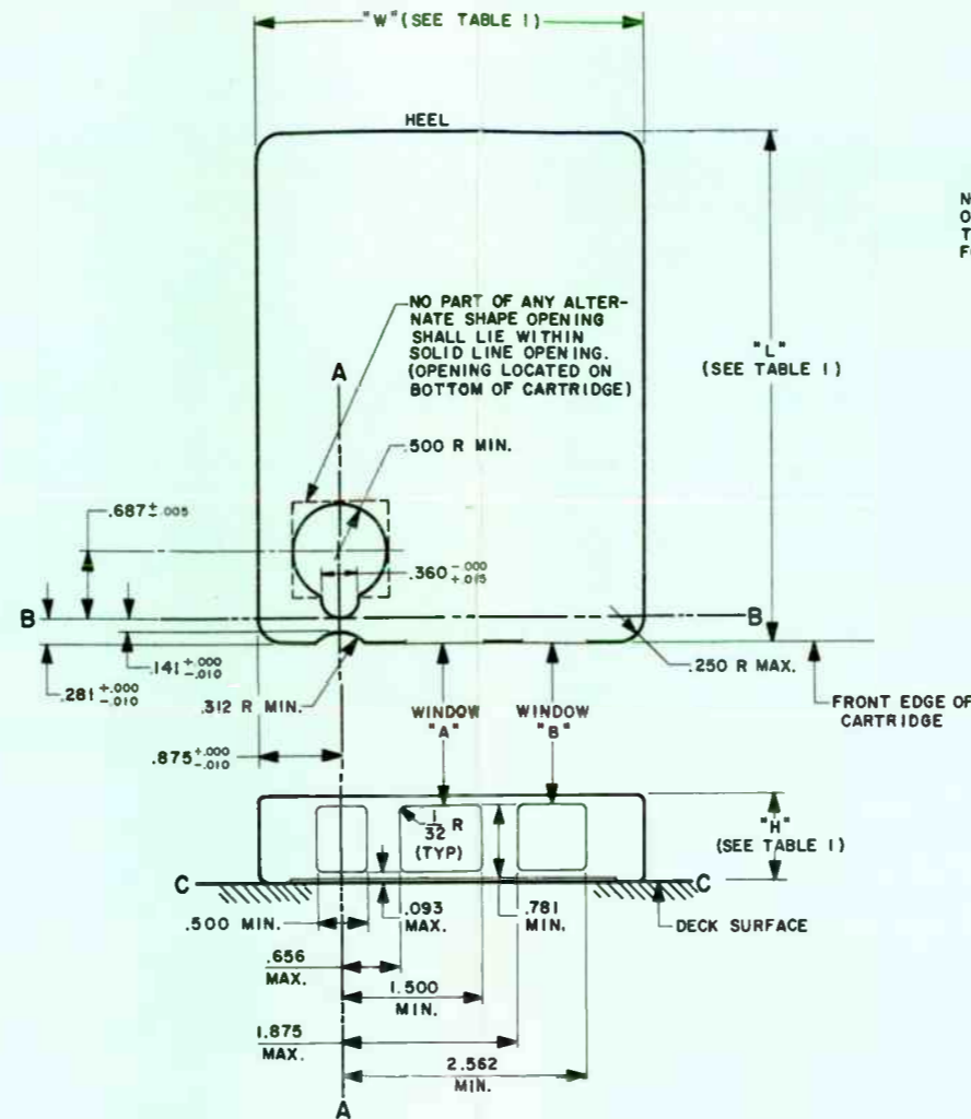
FIG. 3 CARTRIDGE DIMENSIONS
