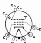
- J - ULTOR = G_2 + CL
