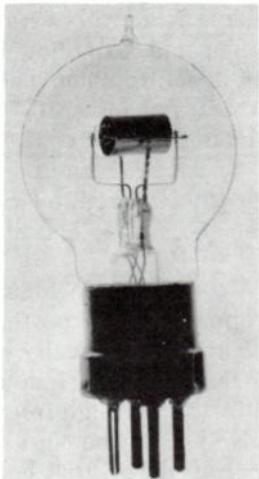
Fig. 10-4. TM Métal tube.
