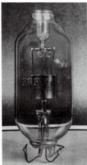
Fig. 18-21. Marconi-Osram ERECT diode.
