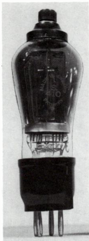
Fig. 18-29. Marconi-Osram S410.
