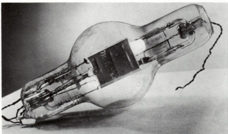
Fig. 22-1. Hansen Gmb 2/250 tube.
