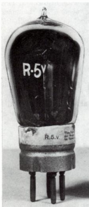
Fig. 18-25. Marconi-Osram R5V valve.
