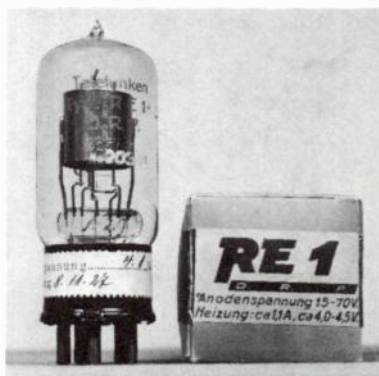
Fig. 21-16. Telefunken RE1 tube.
