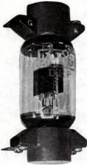
Fig. 12-15. Telefunken K6 tube. (Reproduced from A. Forstmann and E. Schramm, Die Elektronenröhre , Berlin: R. C. Schmidt, 1927.)
