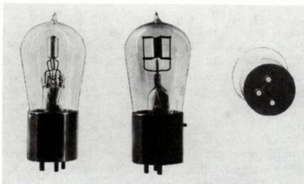
Fig. 8-16. Kenotron TB1 tube.
