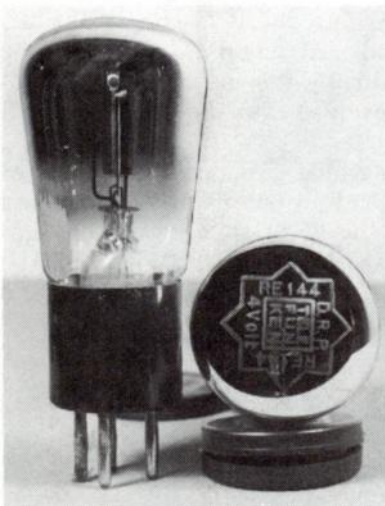
Fig. 21-21. Telefunken RE144 tube.
