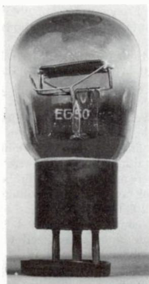
Fig. 22-10. Ostar EG50 110-volt rectifier tube.
