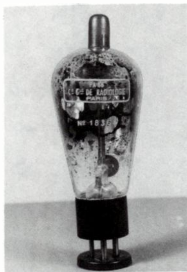
Fig. 19-15. CGR PA68 rectifier.
