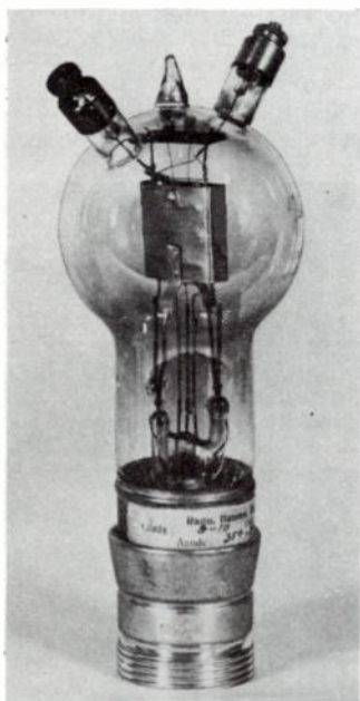
Fig. 22-4. Undesignated Hansen triode.
