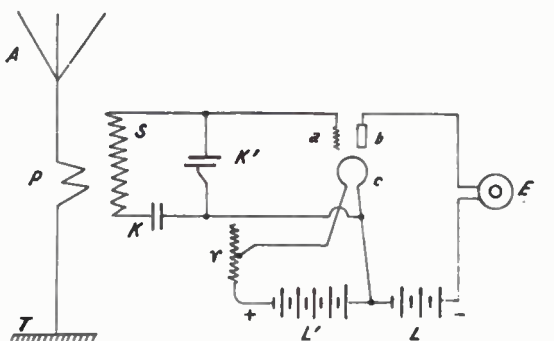
Récepteur de Forest avec lampe Audion
