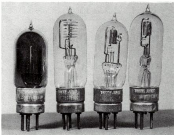
Fig. 19-20. Triode Junot Detecteurs and Amplificateurs.
