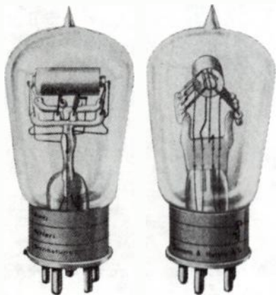
Fig. 21-8. Siemens & Halske Type BO. (Reproduced from Elekt. NachrTech. , Mar. 1925.)
