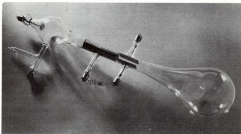
Fig. 2-8. Thomson e/m tube.
