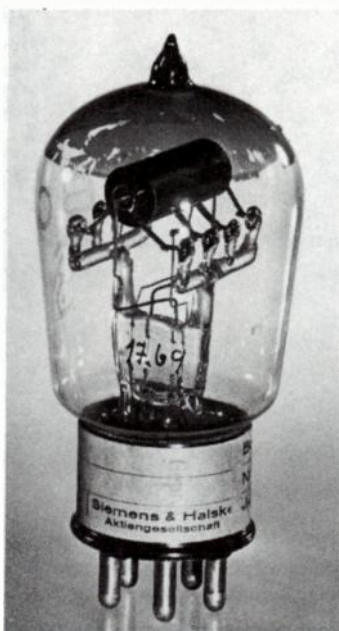
Fig. 21-6. Siemens & Halske BF tube.
