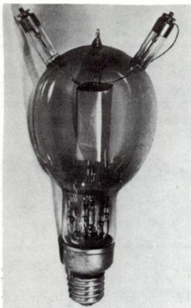
Fig. 22-3. Hansen Gmb 3/500 tube.
