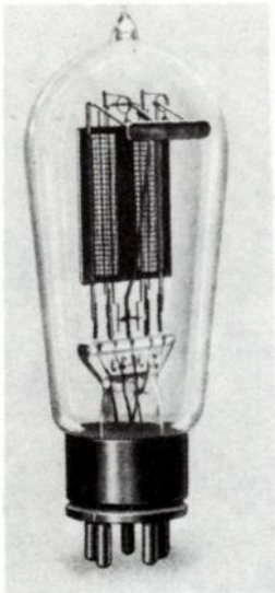
Fig. 21-11. Siemens & Halske CO tube. (Reproduced from Veröff. NachrTech. , 1935, 5.)
