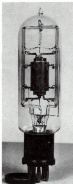
Fig. 21-5. Siemens & Halske OR tube.
