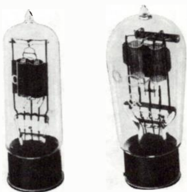
Fig. 21-9. Siemens & Halske OCK tube. Left: OCK of 1925. Right: OCK of 1930. (Reproduced from Veröff. NachrTech. , 1935, 5.)
