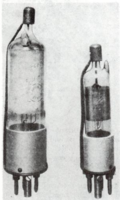
Fig. 21-44. Schott u. Gen tubes. Left: Type k. Right: Type m. (Reproduced from E. Nesper, Handbuch der drahtlosen Telegraphie und Telephonie , Vol. II, Berlin, 1921.)
