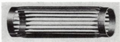
Fig. 21-3. Grid structure of Siemens & Halske R tube. (Reproduced from Veröff. NachrTech. , 1935, 5.)
