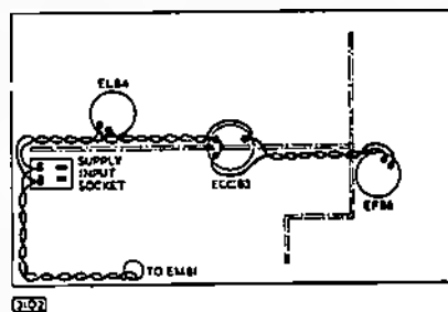
Fig. 9—HEATER WIRING
