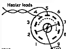
Fig. 11—EF86 VALVEHOLDER
