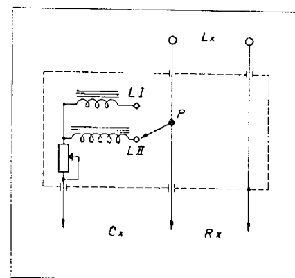
Obr. 6. Doplněk pro měření L
