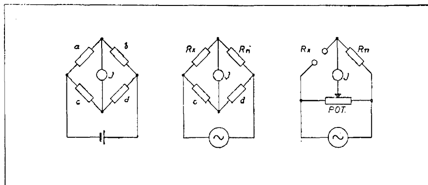
Obr. 2. Základ můstku
