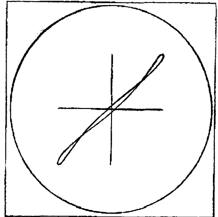
Obr. 7. Správné nastavení fáze v případě, že v signálu chybí druhá a čtvrtá harmonická
