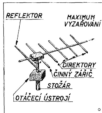
Obr. 9. Antena s direktory.
