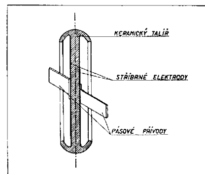
Obr. 5. Taliřový keramický kondensátor pro vysoké napětí.
