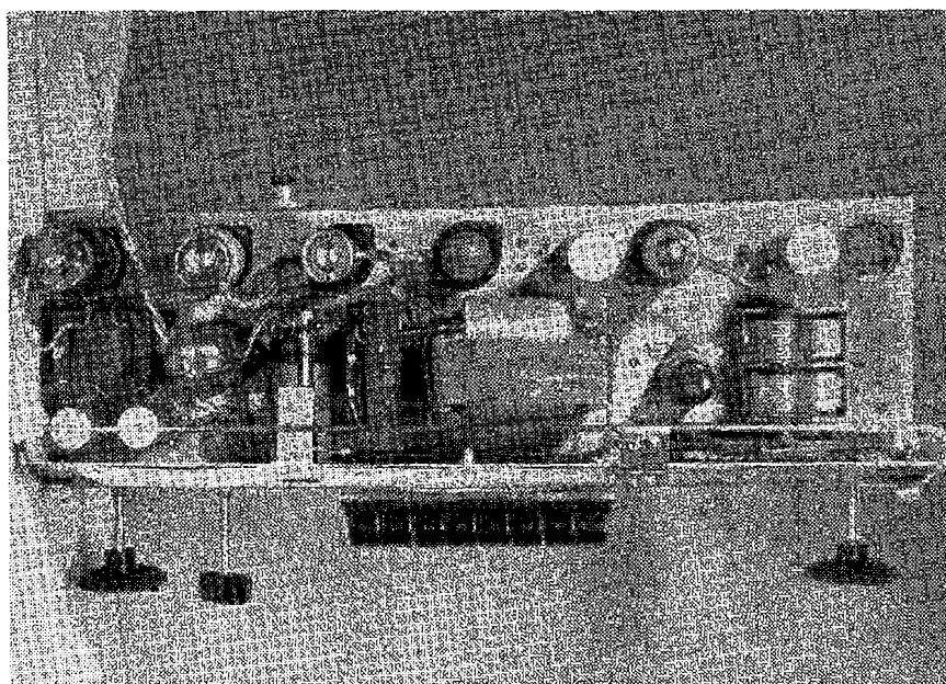
Pohled shora na rozmístění jednotlivých součástek.
