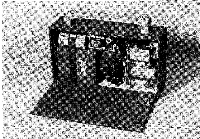
Obr. 3. Víko s rámovou antenou odklopeno. Vlevo od reproduktoru umístěny zdroje.
