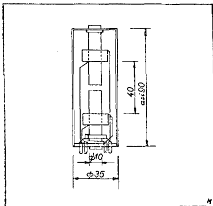
Obr. 5. Cívky: 55 závitů, vf kablík 20×0,07 mm. Ladící kapacita: 200 pF Jádru M7.
