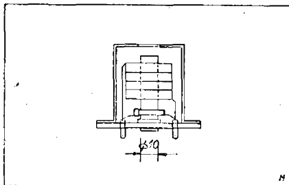
Obr. 7. Cívka: 800 závitů, drát 0,1 mm CuSm. Ladící kapacita: 200 pF. Jádru M7.
