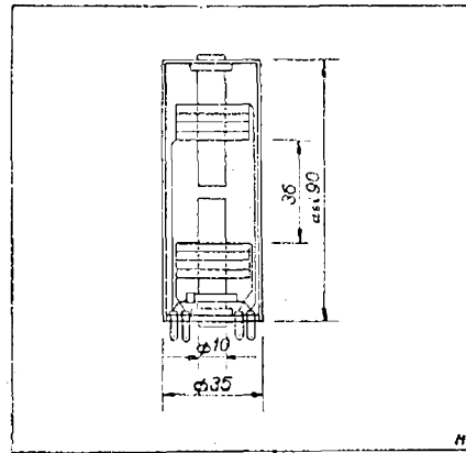
Obr. 8. Cívky: 800 závitů, drát 0,1 mm CuSm. Ladící kapacita: 200 pF. Jádru M7.
