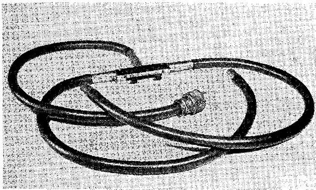
Obr. 4. Funkční sestava přepínače s příslušnými sousými kabely.
