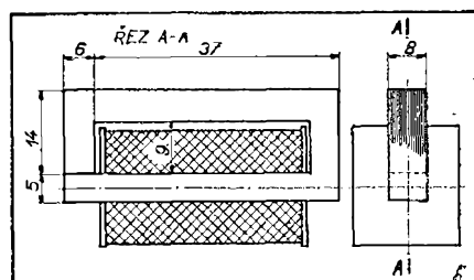
Obr. 8. Náčrt vstupního transformátoru. Na okrajích je stažen 6 mm širokými hliníkovými pásky
