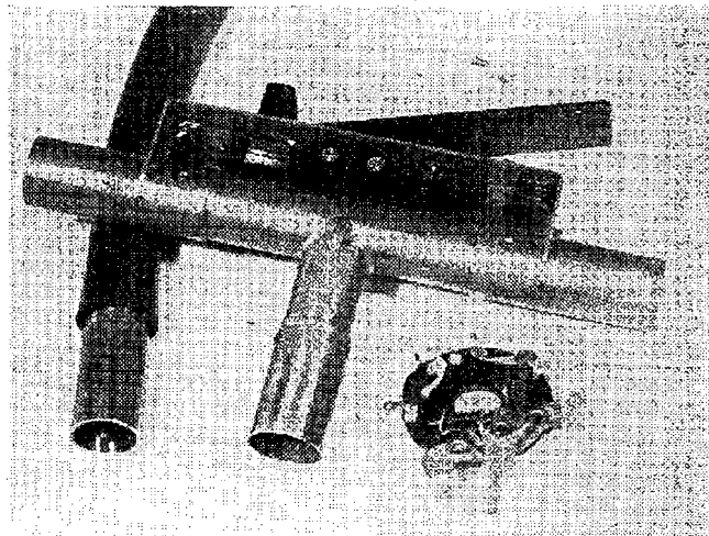
Obr. 5. Na obrázku vpravo dole je přepínač pro 50–650 MHz, který popíšeme příště. Je zhotoven z mžikového přepínače Tesla.
