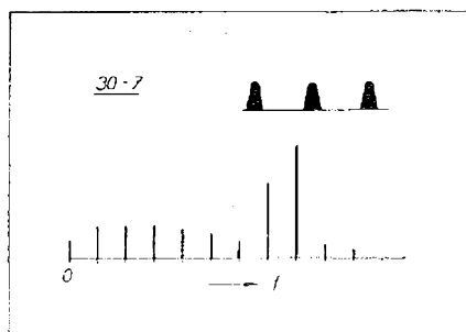
Obr. 30-7: Rozklad průběhu zesíleného zesílení v třídě C na jednotlivé harmonické.
