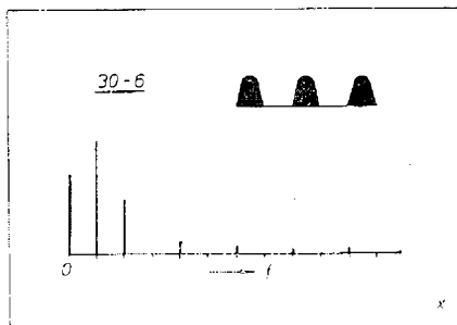
Obr. 30—6: Rozklad průběhu zkresleného zesílení v třídě B na jednotlivé harmonické.
