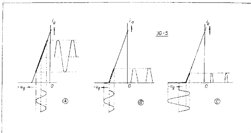
Obr. 30—5: Třídy zesílení: V třídě A se pracovní bod pohybuje po přímé části převodní charakteristiky elektronky, v třídě B je řídící mřížka polarizována do bodu zániku anodového proudu a v třídě C je mřížka polarizována za bod zániku anodového proudu — elektronkou teče proud jen menší část periody.
