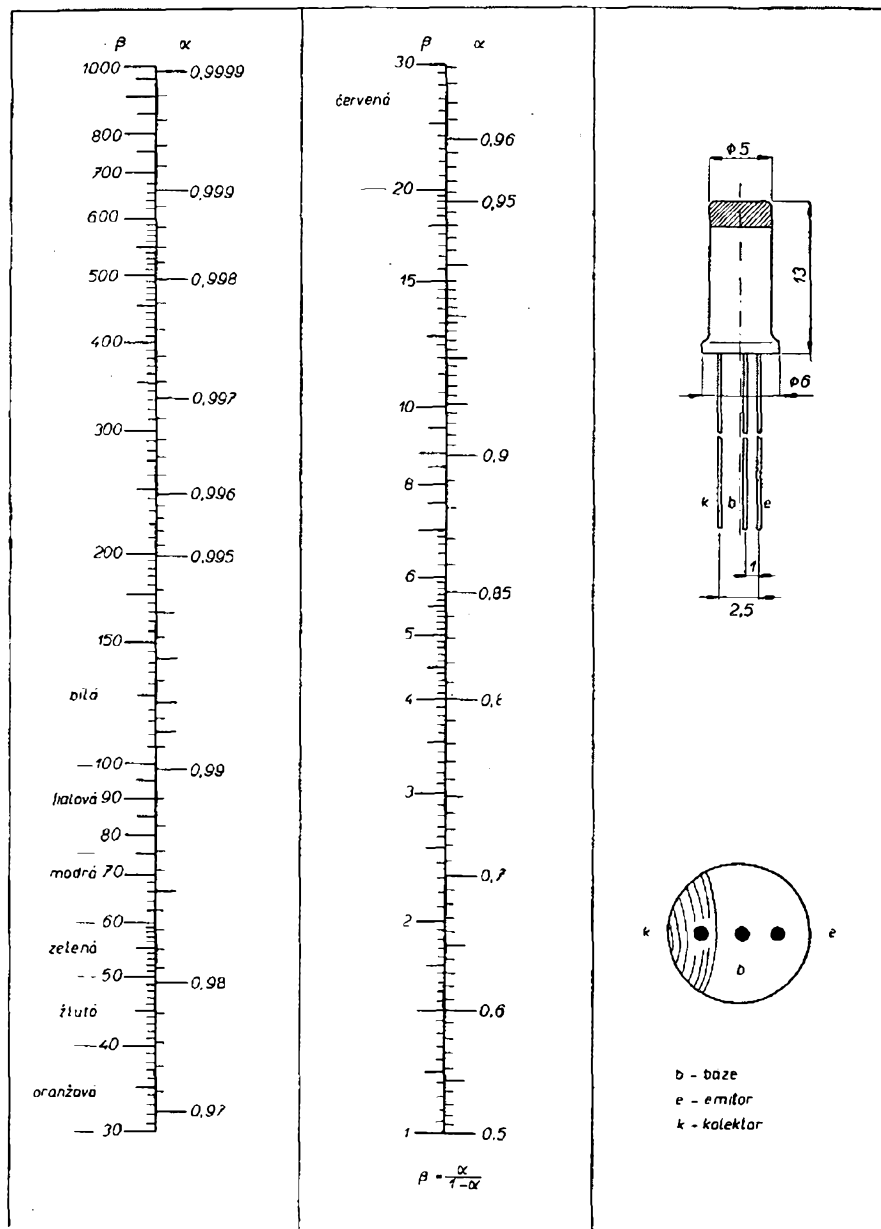
Převod zesilovacího činitele s uzemněnou (vlevo) bází, (vpravo) emitorem
