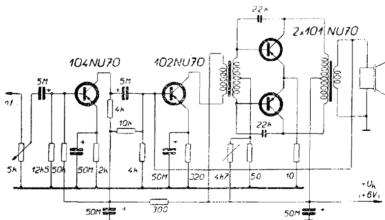
Vzory zapojení jednoduchého přijímače, zpětnovazební přijímače, nf zesilovače
