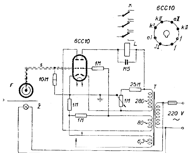
Zapojení fotorelé
