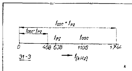
Obr. 31—3: Součtový a rozdílový kmitočet.
