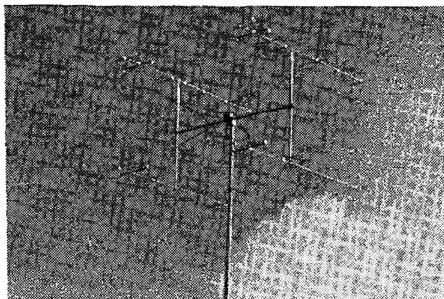
Vlevo: Dvoupatrová anténa pro 420 MHz, kterou podle OK1SO postavili pro PD1959 ve stanici OK1KDO. Vpravo: jeden z našich nejznámějších VKV amatérů OK2VCG inž. Ivo Chládek u svého zařízení
