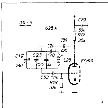
Obr. 30-4: Příklad zapojení oscilátoru v přijímači TESLA 625 A (Hymnus). Hodnoty platí pro první rozsah středních vln.
