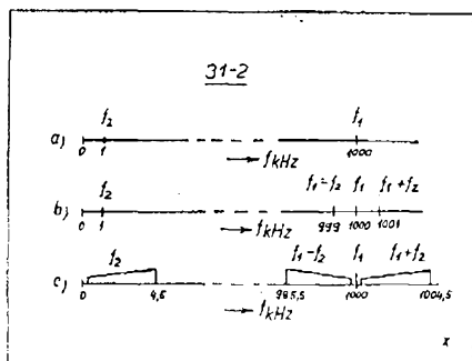
Obr. 31—2: Modulace: a) dva signály před modulací, b) po modulaci c) transpozice kmitočtového pásma.
