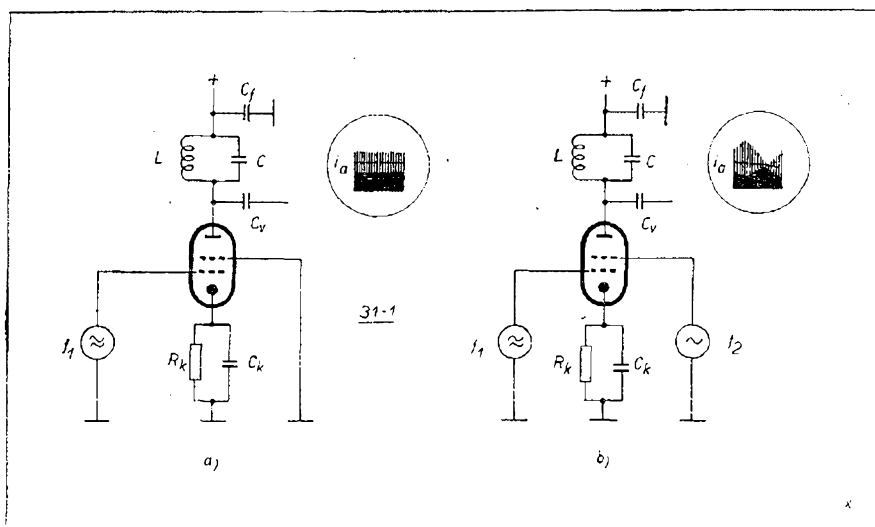
Obr. 31 — 1: Funkce směšovací elektronky: a) druhá řídící mřížka bez signálu, b) signál s různým kmitočtem na obou mřížkách.
