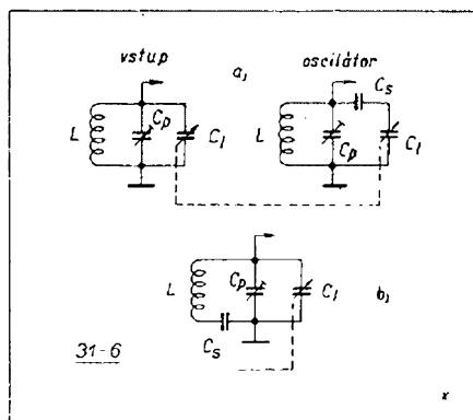
Obr. 31—6: Zajištění souběhu sériovým kondenzátorem: a — princip; b — praktická úprava oscilačního obvodu.
