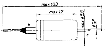
Ge hrotová dioda
