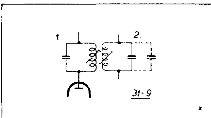
Obr. 31-9: Při sladování jednoho z vázaných rezonančních obvodů je třeba druhý rozladit přidavným kondenzátorem.
