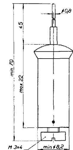
Ge plošný usměrňovač
