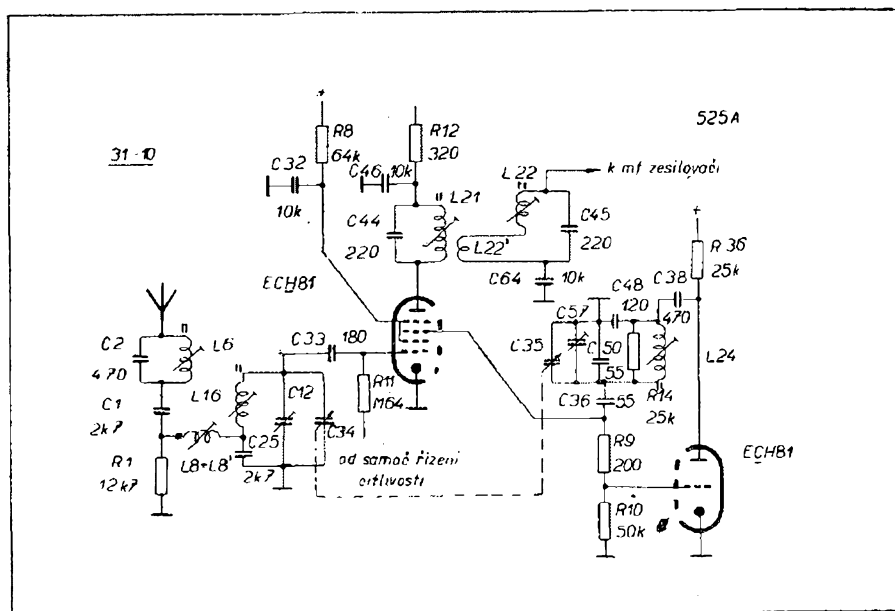
Obr. 31-10: Příklad směšovacího stupně s oscilátorem z přijímače TESLA 525A Kvarteto (dlouhovlnný rozsah).
