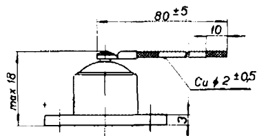
Ge výkonový usměrňovač
