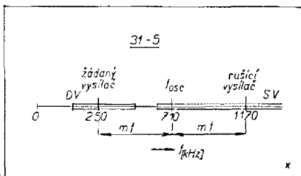
Obr. 31—5: Výklad zrcadlového kmitočtu.
