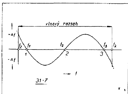
Obr. 31-7: Typický průběh chyby souběhu: f_2, f_4 – začátek a konec rozsahu; f_1, f_2, f_3 – sladovací body.
