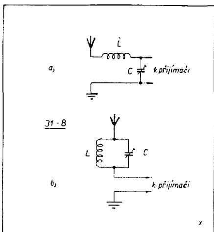
Obr. 31-8: Odladovač zrcadlového (a) a mezi-frekvenčního (b) kmitočtu.
