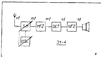
Obr. 31—4: Blokové schéma superhetu: SM — směšovač, OSC — místní oscilátor, MFZ — mezifrekvenční zesilovač, DET — detektor, NFZ — nízkofrekvenční zesilovač.
