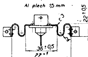
Chladicí plochy pro zvýšení odebraného výkonu
