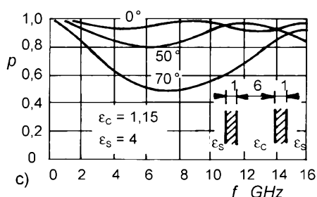
Obr. 3.5 - 2a, 2b, 2c. Elektrické vlastnosti radomů: a) tenkostěnný, b) půlvlnný, c) A - sendvič
