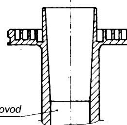
Obr. 3.4 - 3. Tlumivkový trychtýř
