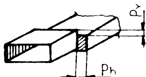
Obr. 2.2 - 4. Paralelní posunutí vlnovodů
