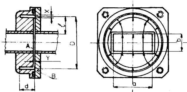
Obr. 2.2 - 2. Tlumivková příruba
