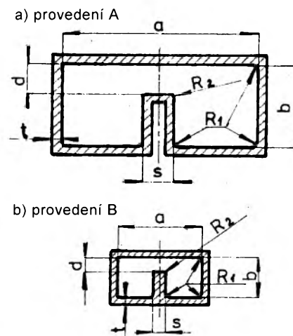
Obr. 1.8 - 2a, 2b. Vlnovod \pi
