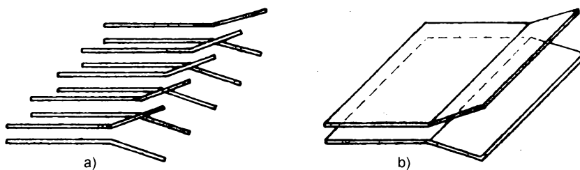
Obr. 1.4 - 4a, 4b. Možnost zvětšení ústí
