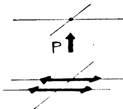
Obr. 3.4 - 14. Elektrické silochary na koncích krátkého páskového vedení
