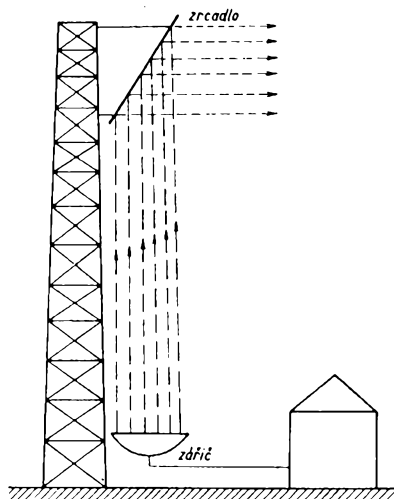
Obr. 3.4 - 1. Periskopická anténa
