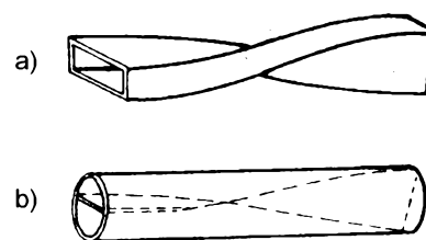
Obr. 2.2 - 15a, 15b. Vlnododové zkruty: a) zkrut na pravouhlém vlnovodu, b) zkrut na kruhovém vlnovodu
