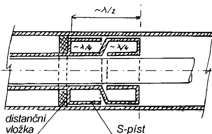
Obr. 2.1 - 20. Bezkontaktní kovový zkrat na koaxiálním vedení
