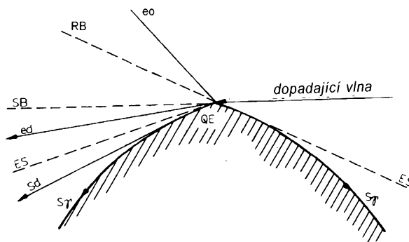
Obr. 1.6 - 1. Dopadající, odražené a rozptýlené paprsky včetně předložených stínů a rozhraní odrazu. Průběh do roviny kolmé ke hřebetu v místě rozptylu
