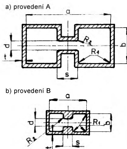
Obr. 1.8 - 1a, 1b. Vlnovod H
