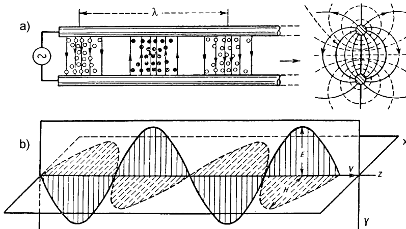
Obr. 1.3 - 5a, 5b. a) Uspořádání elektrických a magnetických siločar v podélné i příčné části nekonečně dlouhého vedení (● směr siločary do nákresny, ○ směr siločary z nákresny), b) Prostorové rozložení elektrického a magnetického vektoru
