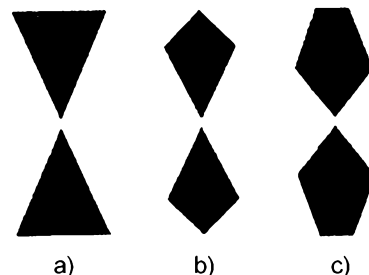
Obr. 3.4 - 11a až 11c. Příklad tištěných zářičů: a) trojúhelníkový dipól, b) trojúhelníkový dipól s čepičkou, c) lichoběžníkový dipól
