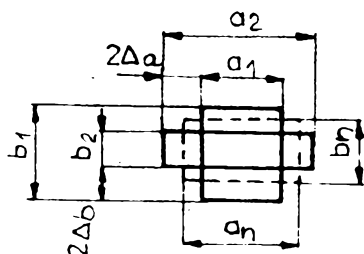
Obr. 2.2 - 3. Nejhorší případ spojení pravoúhlých vlnovodů
