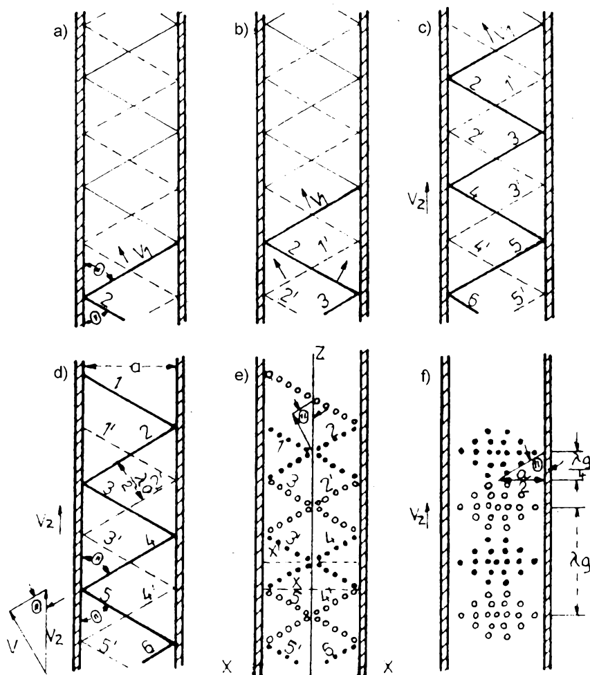
Obr. 1.7 - 1a až 1f. Šíření několikanásobně odraženého čela vlny mezi dvěma kovovými deskami. — elektrické siločáry, - - - - magnetické siločáry ○ - směr z nákrešny, ● - směr do nákrešny
