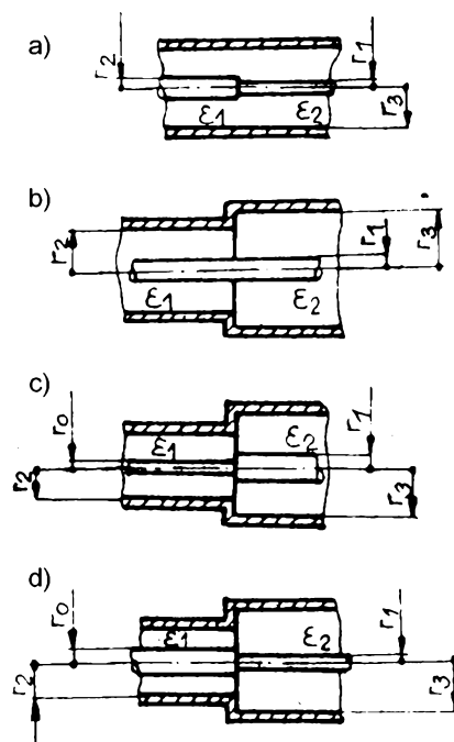
Obr. 2.1 - 9a až 9d. Některé typy skokových diskontinuit v koaxiálním vedení
