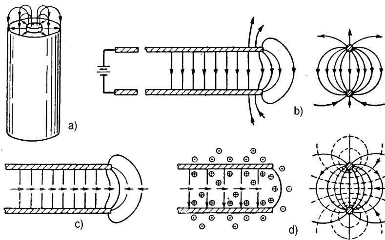
Obr. 1.3 - 1a, 1b, 1c, 1d. Systém siločar, popisující přenos energie stejnosměrného proudu podél dvoudrátového vedení (— elektrické siločáry, - - - magnetické siločáry, ⊕ směr siločáry do náčrtu, ⊙ směr siločáry z náčrtu)
