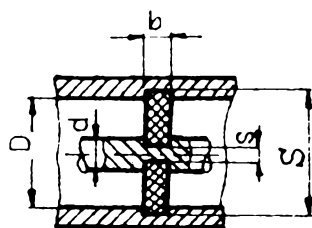
Obr. 2.1 - 4. Kompenzovaná podpěra
