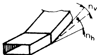
Obr. 2.2 - 5. Vzájemný náklon vlnovodů
