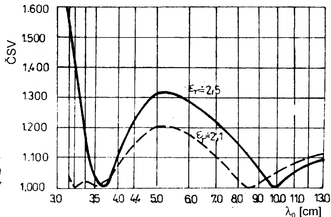
Obr. 2.1 - 19. Činitel stojatých vln (PSV) konektoru N pro různé kmitočty a různé permittivity dielektrické vložky
