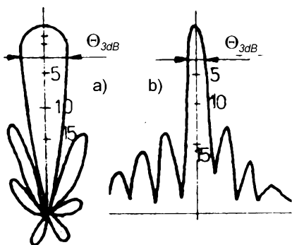
Obr. 3.1 - 2a, 2b. Příklad vyzařovacího diagramu: a) v polárních souřadnicích, b) v pravouhlých souřadnicích
