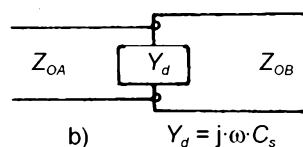
Obr. 2.1 - 8a, 8b. Diskontinuita v koaxiálním vedení: a) rozložení elektrických siločar, b) náhradní schéma
