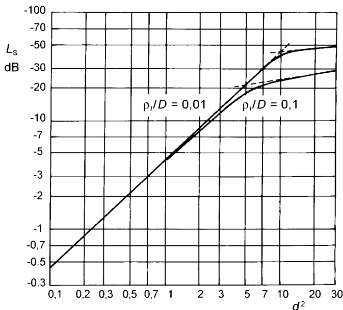
Obr. 3.2 - 8. Ztrátový činitel a povrchová nepřesnost reflektoru
