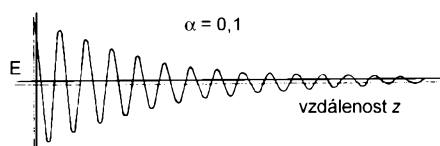
Obr. 1.3 - 6. Vliv útlumu vedení na postupující vlnové čelo
