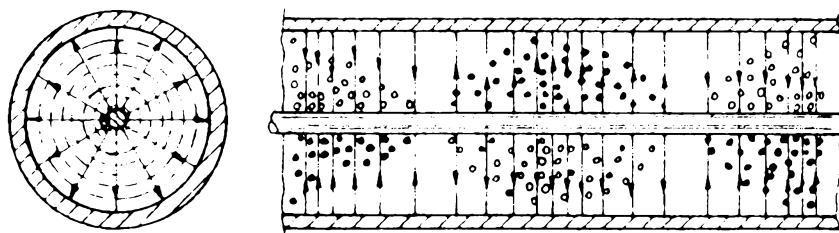
Obr. 1.7 - 7. Uspořádání elektrických a magnetických siločar v příčném a podélném řezu koaxiálním vedením. — elektrické siločáry, ---- magnetické siločáry, ○ - směr z nákresy, ● - směr do nákresy
