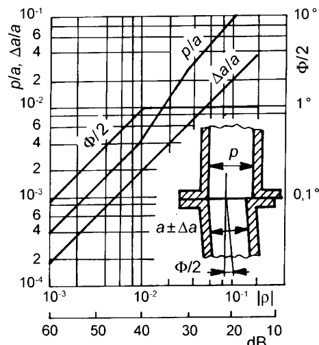
Obr. 2.2 - 8. Závislost koeficientu odrazu na povolené montážní odchylce
