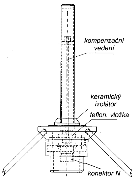
Obr. 3.4 - 8. Unipólová anténa s protiváhou
