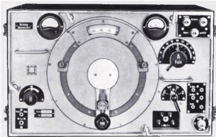
Přístroje z konce první generace spojovací techniky pozemního vojska byly ještě konstruovány s nožičkovými elektronkami. Na fotografiích je rádiová sada Fu 10 s třicetivattovým vysílačem (dole vlevo) a přijímačem E445Bs (dole vpravo), předchůdcem přijímače Torn Eb. Kompletem byly vybaveny průzkumné vozy wehrmachtu. Na přístrojích je patrná konstrukční škola Telefunken. V roce 1936 těmito stanicemi byly vybavovány lehké pancéřované průzkumné vozy (Sd. Kfz. 223)
