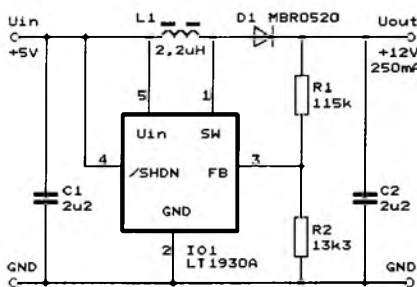
Obr. 15. Zvyšující měnič 5 V/12 V s výstupním proudem 250 mA s obvodem LT1930A
