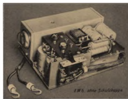
Vibrační měnič pro přijímač Torn Eb
