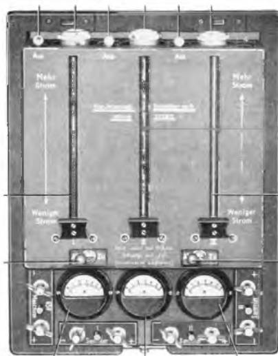
Pro nabíjení žhavicích a měničových akumulátorů byly k nabíjecím soupravám dodávány takovéto rozvaděče
