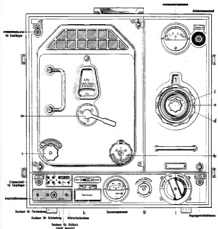
Stowattový vysílač od firmy Lorenz označený 100 WS. Spolu s přijímačem E 445Bs tvořil rádiovou sadu podle standardu z roku 1936 Fu 11
