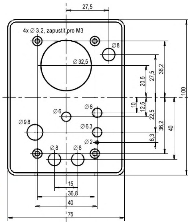
Obr. 6. Vrtání horní stěny krabice U-03-114C testeru (bez měřítka). Průměry a popř. rozmístění děr je nutné upravit podle rozměrů skutečně použitých součástek!
