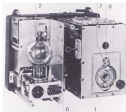
Vysílač FuG 200, 1 - vf vysílací díl, 2 - modulační tyatron, 6 - nastavení kmitočtu, 7 - kluzná spojka, 8 - usměňovací dioda LG12
