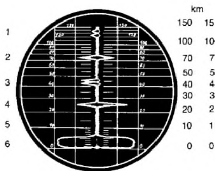
Obr. 1. Obraz na stínitku obrazovky přifunkce lokátoru 1 - pozemní cíl vlevo, 2 - námořní cíl přesně vpředu, 3 - námořní cíle vlevo, 4 - námořní cíl vpředu vpravo, 5 - šumová hladina přijímače, 6 - startovací impuls „mořský had“
