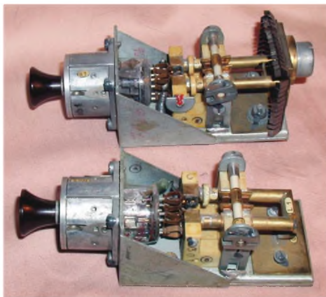
Perfektně provedené vstupní obvody přijímače. Nahoře směšovač s diodou LG7, pod ním oscilátor s tródou LD1. Tyčové rezonanční obvody se ladily v pásmu okolo 550 MHz. U novějších modelů FuG 200 určených pro Luftwaffe bylo možno pomocí motorku přeladit pracovní frekvenci během letu
