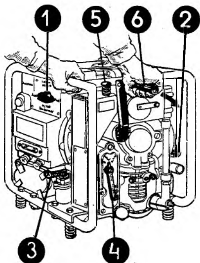
Pro zajištění provozu rádiových stanic, které byly ve výbavě tanků, obrněných transportérů a radiovozu, byla dodávána celá řada nabíjecích soustrojí o výkonu od 100 W do 5 kW (orázek nahoře a dole)
