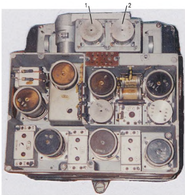
Pohled na přijímač. Nahoře vstupní obvod (1 - směšovací dioda LG7, 2 - oscilátorová tróda LD1). Pod tím blok mezifrekvenčního zesilovače
