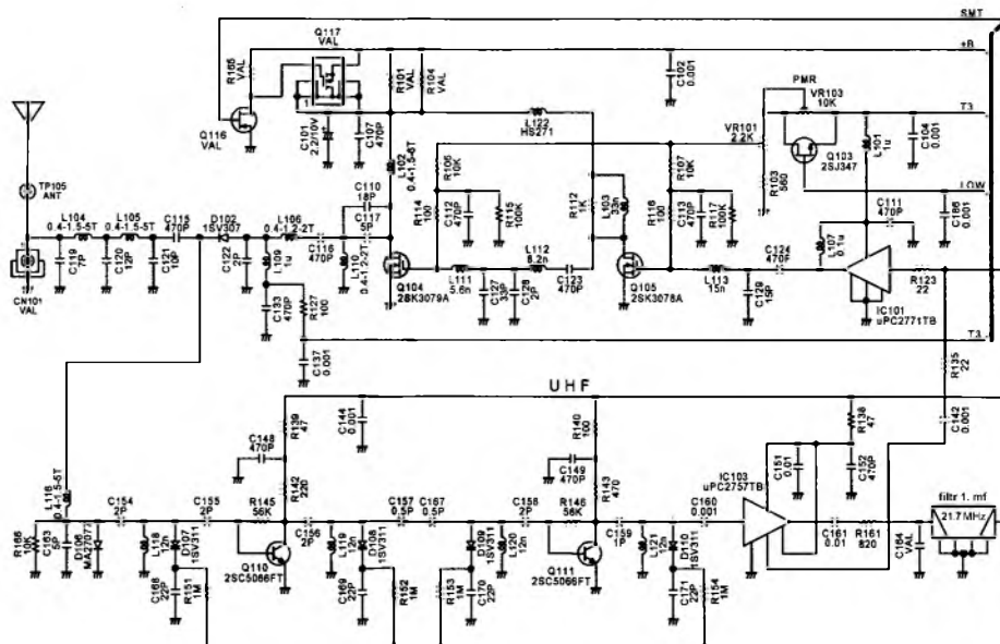
Obr. 17. Zapojení vf dílu radiostanice ALINCO DJ-S45CQx
