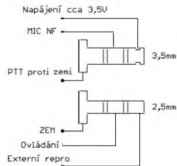
Obr. 29. Zapojení konektorů JACK u stanic KENWOOD
