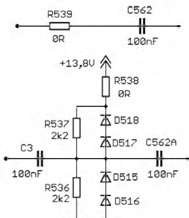
Obr. 24. Přidavné diody pro ochranu vstupů ALINCO DX-77E. Nahoře je původní zapojení v DX-77E, dole je upravené zapojení s ochrannými diodami převzaté z DX-707
