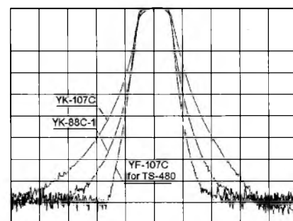
Obr. 40. Charakteristika CW filtru 500 Hz typu YF-107C. Vodorovná osa: 500 Hz/dílek, střední kmitočt 10,695 MHz, svislá osa: 10 dB/dílek
