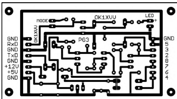
Obr. 80a. Obrázek spojů na desce převodníku PG3 (měř.: 1 : 1, skutečný rozměr 80 x 44 mm)
