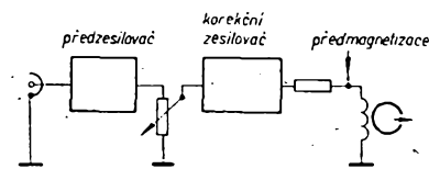
Obr. 58. Blokové zapojení záznamového zesilovače magnetofonu
