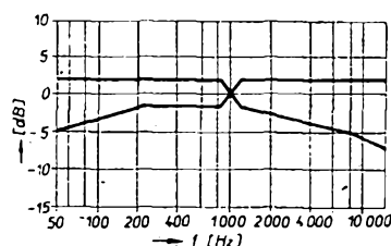
Obr. 34. Toleranční pole kmitočtové charakteristiky sluchátek
