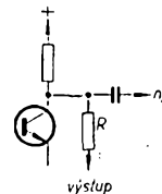
Obr. 61. Běžné provedení napěťového výstupu magnetofonů se sériovým odporem R
