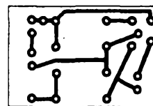
Obr. 65. Deska s plošnými spoji impedančního měniče
