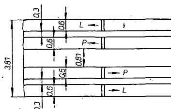
Obr. 11. Uspořádání stop u kazetových přístrojů pro stereofonní provoz
