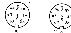
Obr. 47. Provedení konektoru s možností dálkového ovládání a připojení elektretového mikrofonu (a) a zásuvky (b)
