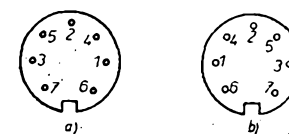
Obr. 46. Provedení konektoru s možností dálkového ovládání (a) a zásuvky (b)
