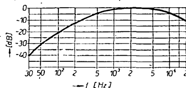
Obr. 57. Kmitočtová charakteristika propustí pro měření odstupu rušivých napětí (křivka A)
