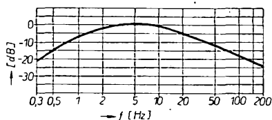
Obr. 56. Kmitočtová charakteristika měřiče kolísání rychlosti posuvu pásky
