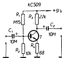
Obr. 64. Zapojení předzesilovače
