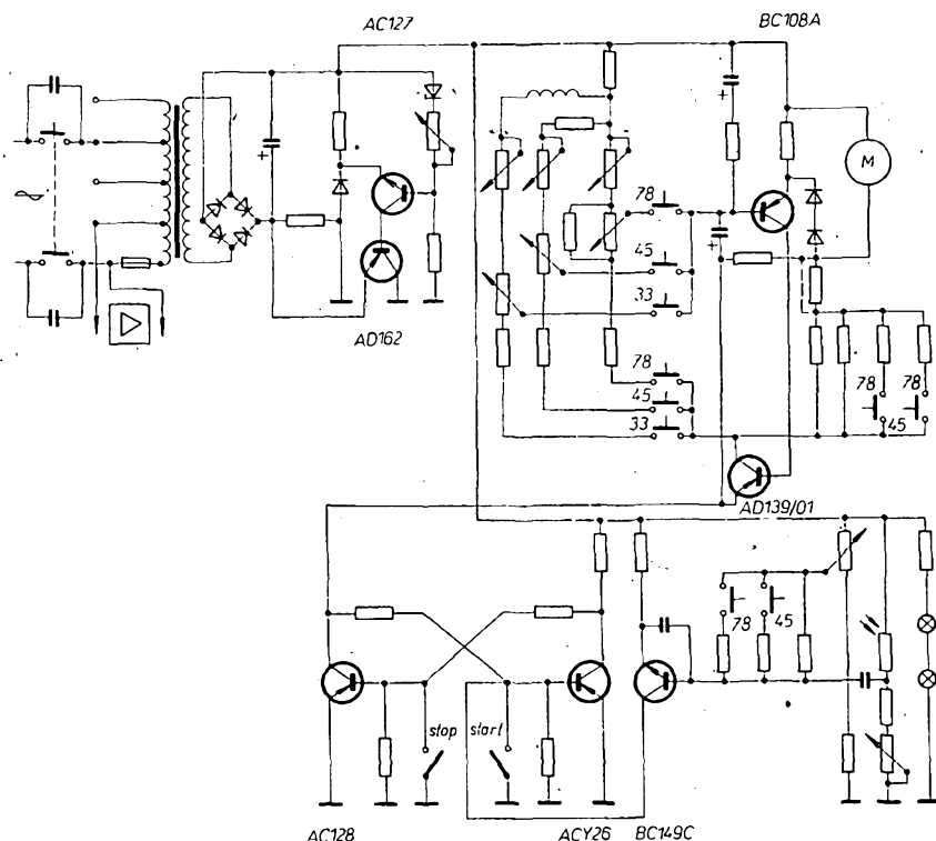
Obr. 3. Schéma zapojení elektronické regulace gramofonu Philips
