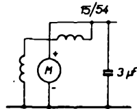
Obr. 86. Odrušení motoru stěračů v pásmu SV, DV
