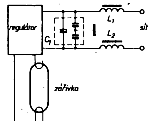
Obr. 56. Odrušení stmívače žárovky; C_1 – WK 72491/50 nF + 2 \times 2,5 nF , L_1 , L_2 – WN 68206 ( 2 \times 6,3 mH )
