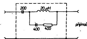
Obr. 91. Umělá anténa podle ČSN 367090
