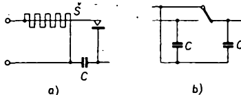
Obr. 22. Jednoduché odrušení termostatu kondenzátorem; kapacita kondenzátoru C je asi 50 až 100 nF (0,05 až 0,1 \mu F )
