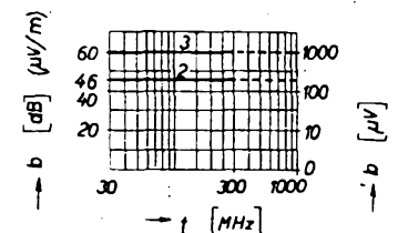
Obr. 7. Meze rušivých polí v pásmu 30 až 300 MHz pro elektrické stroje, přístroje a zařízení (stupeň odrušení 2, 3)
