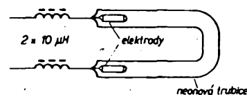
Obr. 68. Vř tlumivky 10 \mu H navinuté na feritové tyčince \varnothing 3 mm (20 závitů o \varnothing 4 mm CuL) omezi rušivé vyzařování neonové reklamy na kmitočtech nad 30 MHz
