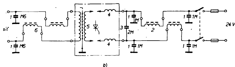
b) odrušení měniče 1 kVA na mez 1. 1, 3, 7 – odrušovací kondenzátory, 2 – odrušovací dvojítlumivka 28 μH, 2 × 75 A, 3 – tlumivky k omezení proudu, 5 – výstupní transformátor, 6 – odrušovací dvojítlumivka 2 × 65 μH, 6 A
