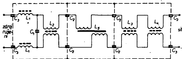
Obr. 119. Síťový filtr pro nejnáročnější použití. C_1 – svítkový kondenzátor 1000 pF/600 V, C_2 – průchodkový kondenzátor 1,25 až 2,5 nF (např. WK 713 31), C_3 – keramický průchodkový kondenzátor 470 pF/250 V, L_1 – VKV tlumivka 10 \mu H/2,5 A, L_2 , L_3 – toroidní dvojité tlumivky 2 \times 4 mH (WN 68211), L_4 – dvojité tlumivky 2 \times 2,5 mH (WN 682 03), L_5 – dvojité VKV tlumivky WF 607 10. Při konstrukci je nutno dodržet naznačené přepážky
