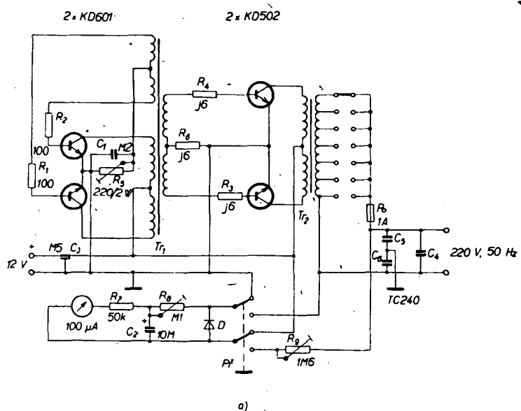
Obr. 63a. Odrušení střídače 12 V/220 V/50 Hz. Na stejnosměrné straně je zařazen průchodkový kondenzátor WK 71340 (0,5 μF), na výstupu 220 V/50 Hz širokopásmový kondenzátor TC 240;
