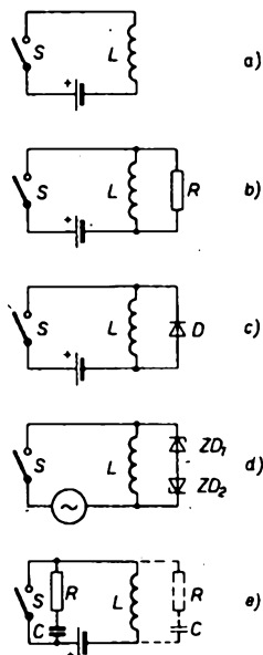
Obr. 20. Vznik rušení na rozepínajícím kontaktu v obvodu s indukčností (a), omezení rušení paralelním odporem k cívce (b), omezení rušení kontaktu paralelní diodou (c), Zenerovými diodami (d) a zřáhacím obvodem RC (e)
