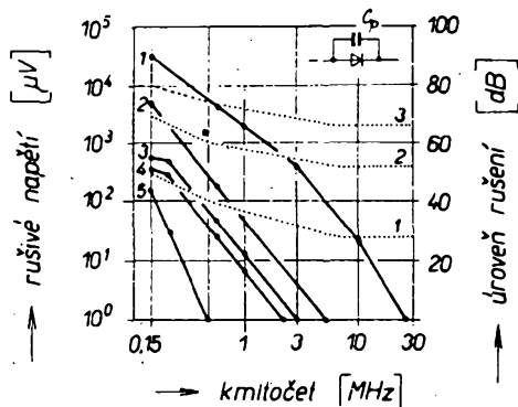
Obr. 52. Kmitočtový průběh rušivého napětí křemíkového jednocestného usměrňovače při zapojení kondenzátorů o různých kapacitách; 1 – bez zapojeného kondenzátoru, 2 – C_p = 0,01 \mu F , 3 – C_p = 0,025 \mu F , 4 – C_p = 0,05 \mu F , 5 – C_p = 0,5 \mu F
