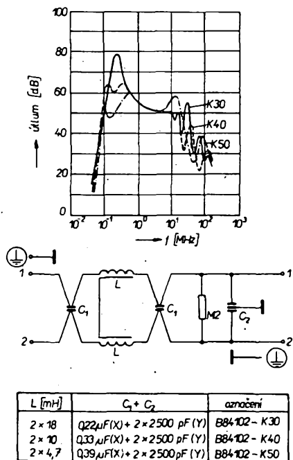
Obr. 118. Zapojení síťového filtru Siemens B 84 102 a graf závislosti útlumu na kmitočtu. Použité kondenzátory jsou širokopásmové. Odpor 200 \Omega/0,5 W odstraňuje zbytkový náboj kondenzátorů po odpojení od sítě
