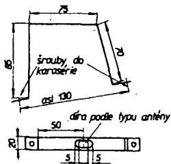
Obr. 96. Příchytka pro autoanténu, umístěnou v zadní části kapoty motoru automobilu Wartburg 353
