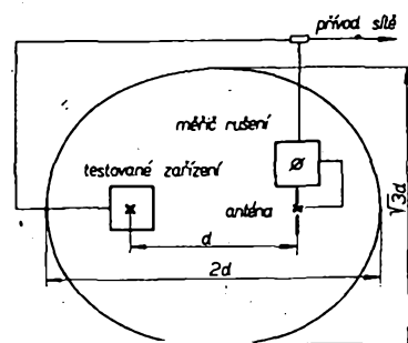
Obr. 19. Minimální požadavky na volný prostor při měření rušivého pole. Rozměry elipsy se odvozují od měřicí vzdálenosti d (ta je podle typu rušivého zdroje určena normou na 3 m, 10 m, 30 m nebo 100 m)
