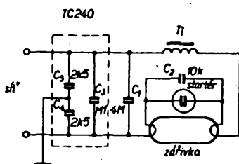
Obr. 64. Zapojení odrušovacích kondenzátorů u zářivky; C_1 – kompenzace účinníku; C_2 je již vestavěn v pouzdrů startéru; C_3 , C_4 , C_5 odrušovací kondenzátor TC 240
