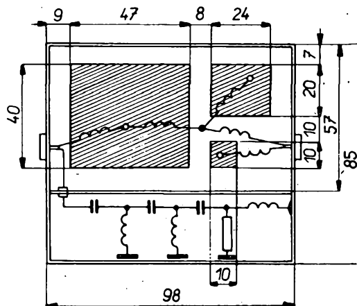
Obr. 120. Absorpční filtr k amatérskému vysílači s výkonem do 50 W. Mezní kmitočet 40 MHz. Rozměry odpovídají kupřetitu s tloušťkou 0,7 mm (oboustranně plátovaný)
