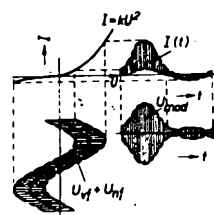
Obr. 111. Vznik absorpční modulace na nelinearitách obvodu
