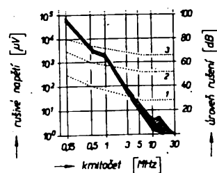
Obr. 51. Kmitočtový průběh rušivého napětí křemíkového usměrňovače při proudu I_d = 10 \text{ A} a síťovém napětí 15 až 220 V, 50 Hz
