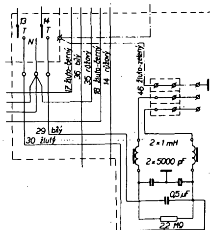
Obr. 30. Odrušení automatické pračky Supertatramat. Kromě centrálního filtru v síťovém přívodu doplňuje odrušení dvojitý člen RC 0,2 \mu F + 50 \Omega přepínače 1 programátoru
