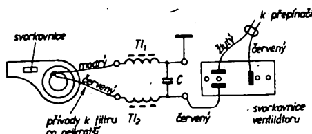
Obr. 88. Dodatečné odrušení ventilátoru topení osob. vozů ŠKODA; T_1 , T_2 jsou vinuty na feritovém jádru o \varnothing 6 mm, l = 30\text{ mm} , 35 z drátu o \varnothing 0,8 mm CuL. Kondenzátor C je keramický, 47 nF až 0,1 \mu\text{F} . Filtř je upevněn k tělesu motoru ventilátoru
