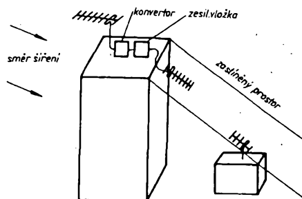
Obr. 121. Nedovolený způsob distribuce TV signálu
