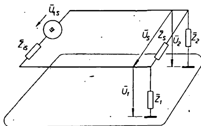
Obr. 2. Náhradní schéma neuzemněného zdroje rušení
