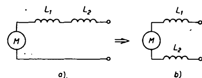
Obr. 32a, b. Symetrické zapojení satorových cívek L_1 , L_2 komutátorového motorku je základní podmínkou odrušení
