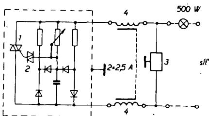
Obr. 60. Stmívač z obr. 57 s regulátorem v kovovém krytu s ochranou nulováním; 1 – triak, 2 – diak, 3 – odrušovací kondenzátor 0,1 μF + 2 × 2,5 nF, 4 – tlumivka 2 × 6,3 mH
