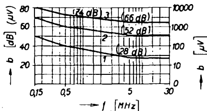
Obr. 5. Meze rušivých napětí pro elektrické stroje, přístroje a zařízení (stupeň odrušení 1, 2, 3)
