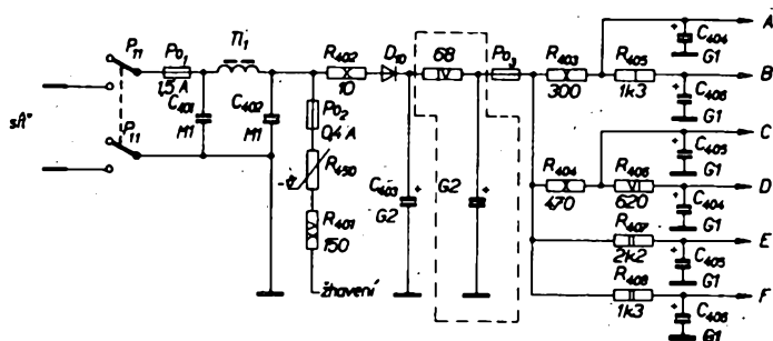
Obr. 108. Úprava napájecího dílu starších televizních přijímačů TESLA filtrem RC (68 \Omega , 200 \mu\text{F} )
