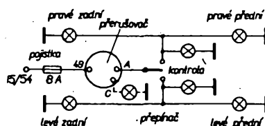
Obr. 89. Obvyklé zapojení přerušovače směrových světel
