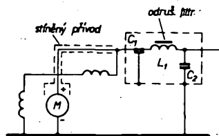
Obr. 87. Odrušení motoru stěračů filtrem C_1 – průchodkový kondenzátor WK 71335 (50 nF), C_2 – 2,5 \mu\text{F}/50\text{ V} , L_1 – WN 68211 (2 \times 4 mH) v sérii
