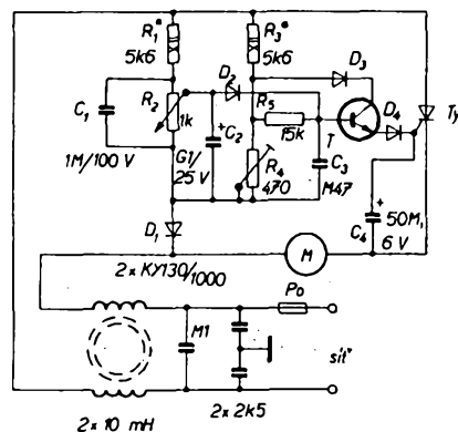
Obr. 62. Odrušení regulátoru otáček filtrem z dvojité toroidní tlumivky WN 682 12 (2 × 10 mH) a širokopásmového kondenzátoru TC 240 (0,1 μF + 2 × 2,5 nF)
