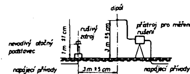
Obr. 10. Uspořádání měřicího pracoviště pro měření rušivých polí v pásmu 30 až 300 MHz
