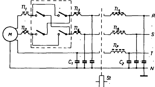
Obr. 29. Odrušení automatické plynové pračky Moretta typ 855; M – motor, St – stykač, T_1 až T_8 – WF 60708 (tlumivka UKV 12 \mu H, 2,5 A, 250 V), T_1 až T_8 – TL 10000 (2,5 mH) C_1 , C_2 – TC 11011, 3 \times 0,1 \mu F + 5 nF/380V~
