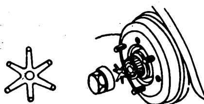
Obr. 90. Dodatečná úprava pro spojení disku kola s hřídelí (u nepoháněných kol)
