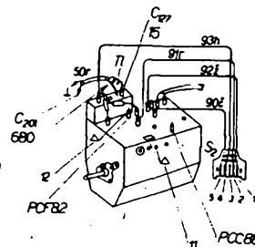
Obr. 101. Omezení rušivého vyzářování kanálového voliče KP 21 (Dajana, Blanky, Oliver atd.) tlumivkou na mříž výstupu
