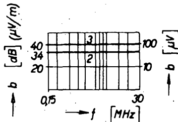
Obr. 6. Meze rušivých polí v pásmu 0,15 až 30 MHz pro elektrické stroje, přístroje a zařízení (stupeň odrušení 2, 3)
