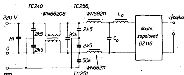
Obr. 70. Odrušení svítilny se sodíkovou výbojkou a doutnavkovým zapalovačem. WN 68211 má indukčností 2 \times 4 mH
