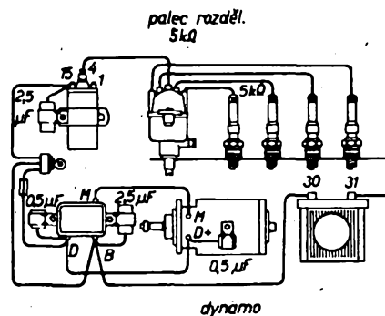
Obr. 83. Použití základních odrušovacích prvků pro odrušení v pásmu DV, SV. Kondenzátory mohou být průchodkové. Odrůšení zapalovacích kabelů se liší podle typu vozu
