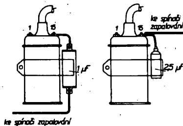
Obr. 93. Umístění a zapojení odrušovacích kondenzátorů u zapalovací cívky
