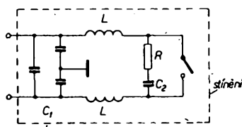
Obr. 25. Velmi účinné odrušení kontaktu (kombinace odrušovacích prostředků a stínění); C_1 – průchodkový kondenzátor 0,1 \mu F + 2 \times 2,5 nF , C_2 - 0,1 až 1 \mu F , R - 20 až 100 \Omega , L - 1 mH
