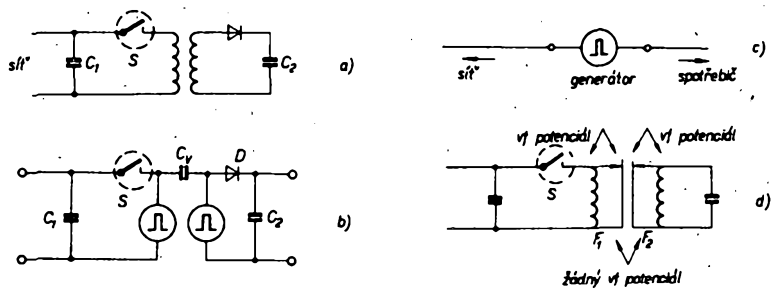
Obr. 106. Princip potlačení rušení konstrukcí transformátoru. ( S – spínací prvek – tyristor, tranzistor); F 1 , F 2 stínící fólie
