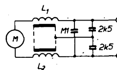
Obr. 33. Odrušení komutátorového motoru širokopásmovým kondenzátorem
