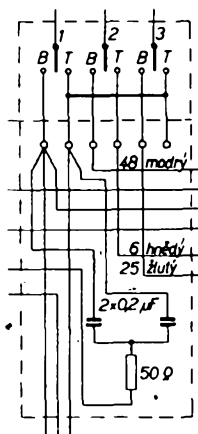
Obr. 30. Odrušení automatické pračky Supertatramat. Kromě centrálního filtru v síťovém přívodu doplňuje odrušení dvojitý člen RC 0,2 \mu F + 50 \Omega přepínače 1 programátoru
