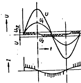
Obr. 74. Průběh napětí a proudu při kapacitních průrazech izolační vrstvy
