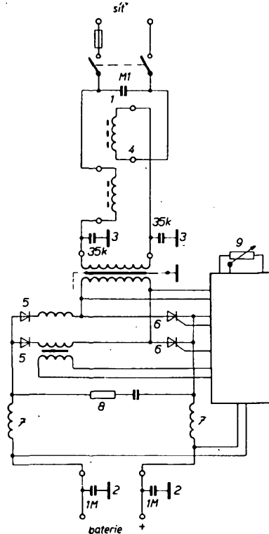
Obr. 55. Základní zapojení s odrušením pro mez „2“; 1, 2, 3 – odrušovací kondenzátory, 4 – odrušovací dvojtlumivka 2 \times 2 A 1,1 mH , 5 – křemíkové diody, 6 – tyristory, 7 – vyhlazovací tlumivky, 8 – člen RC, 9 – řídicí člen
