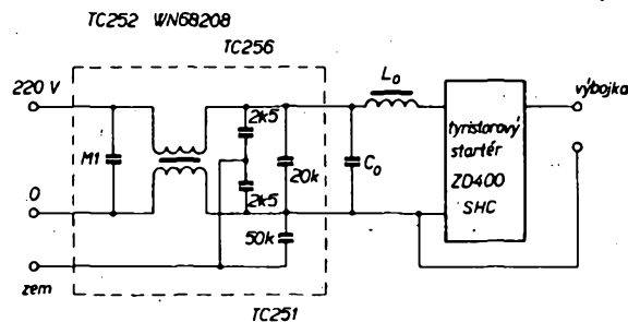
Obr. 69. Odrušení svítilny se sodíkovou výbojkou a tyristorovým startérem. Tlumivka WN 68208 má indukčností 2 \times 6,2 mH. L_0 – pracovní tlumivka, C_0 – kompenzační kondenzátor
