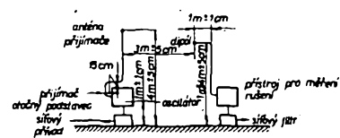
Obr. 12. Uspořádání pracoviště pro měření rušivého vyzářování rádiových přijímačů v pásmu 30 až 1000 MHz
