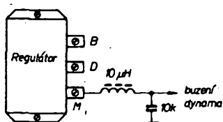
Obr. 81. Odrůšení svorky M regulátoru pro omezení rušení v pásmu UKV
