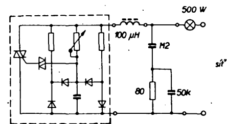
Obr. 57. Odrušení stmívače žárovky. Kryt regulátoru z plastické hmoty nebo kovový (viz obr. 58)
