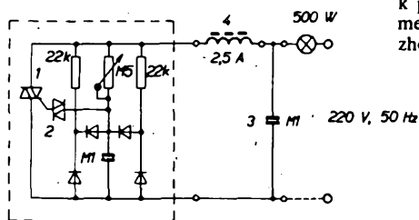
Obr. 59. Odrušení stmívače z obr. 57 na mez 2; 1 – triak, 2 – diak, 3 – odrušovací kondenzátor 0,1 μF/250 V, 4 – odrušovací tlumivka na toroidním jádře 6,3 mH. Regulátor v izolovaném krytu
