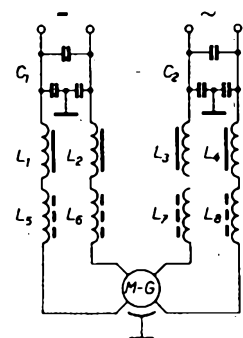
Obr. 43. Odrušení měniče na mez č. 1; C_1, C_2 - \text{širokopásmový kondenzátor } 0,1 \mu\text{F} + 2 \times 2,5 \text{ nF} , L_1, L_2, L_3, L_4 - 0,4 až 2 \text{ mH} , L_5, L_6, L_7, L_8 - 10 \mu\text{H}
