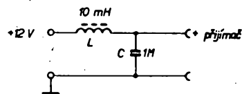
Obr. 98. Filtr do napájecího přívodu autorádia, C – WK 71342, 1 μF, L – WN 68212 (zapojena 1 sekce, 10 mH)
