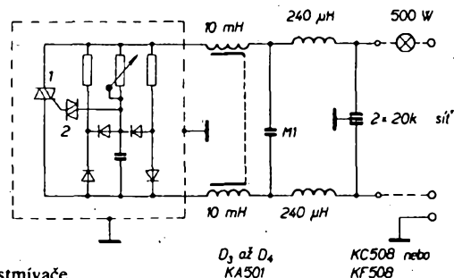
Obr. 61. Stmívač z obr. 57 s regulátorem v kovovém krytu (ochrana nulováním) odrušeným na mez 1. Průběh rušivého napětí obr. 58, křivka 6
