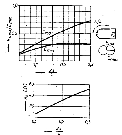
Obr. 54. Vyzářovací diagram a reálný vstupní odpor antény U
