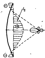
Obr. 106. Nevhodné ozáření paraboly
