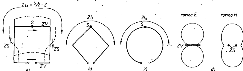
Obr. 56. Smyčkové antény a jejich vyzářovací diagram
