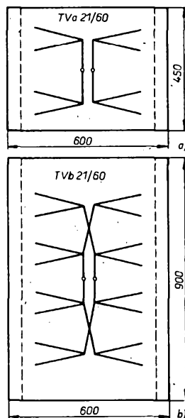
Obr. 97. Antény Kovožávodu Plzeň („madrace“)
