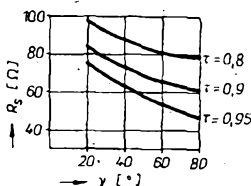
Obr. 90. Vstupní reálný odpor rovinné antény LP
