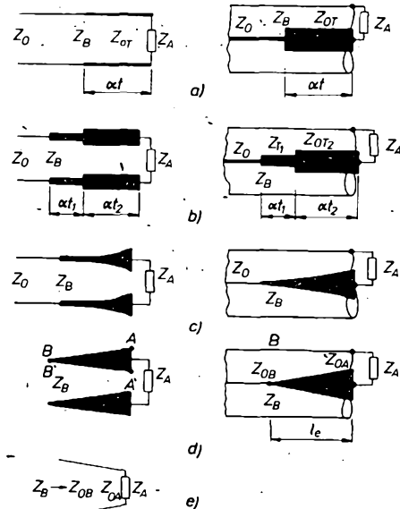
Obr. 20. Linkové transformátory
