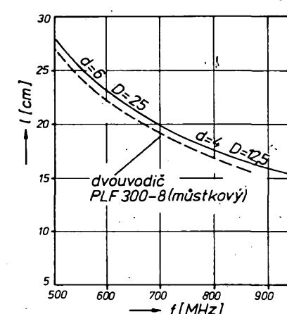
Obr. 51. Optimální délka skládaného dipólu z trubek a z dvou vodiče
