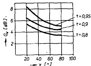
Obr. 89. Zisk rovinné antény LP
