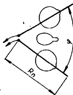
Obr. 77. Vznik výsledného vyzařovacího diagramu
