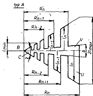
Obr. 73. Tvar základní jednotky logaritmicko-periodické antény
