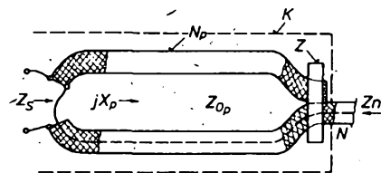
Obr. 33. Balun se zlepšenou symetrií
