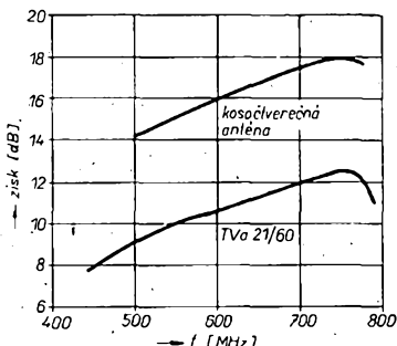
Obr. 12. Průběh zisku
