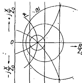
Obr. 15. Pravouhlý impedanční diagram
