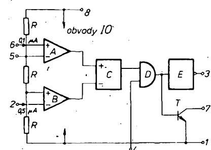
Obr. 2. Blokové schéma IO NE555. A, B – komparátory, C – klopný obvod, D – součinný obvod, E – výstupní obvod; vývody: 1 – zem, 2 – dolní práh (spouštění), 3 – výstup, 4 – nulování, 5 – napěťová kontrola, 6 – horní práh, 7 – vybití, 8 – napájení
