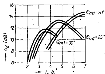
Obr. 64. Průběh zisku typických kosočtverečných antén
