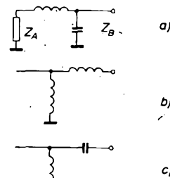
Obr. 23. Varianty impedančního přizpůsobení
