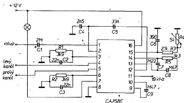
Obr. 9. Schéma zapojení CA758E
