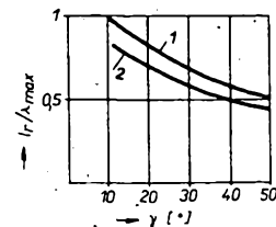
Obr. 79. Závislost I_r na \gamma
