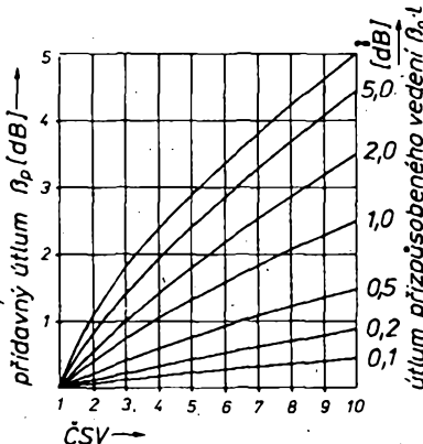
Obr. 3. Přídavné ztráty vedení
