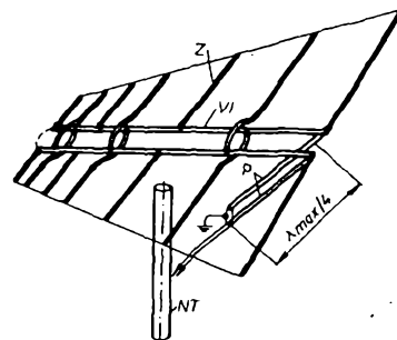
Obr. 91. Rovinná anténa LP
