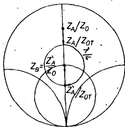
Obr. 21. Impedanční průběh na jedno- stupňovém transformátoru.
