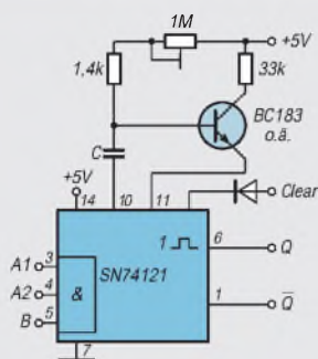
Bild 18: Mit einem Transistor erweiterte Schaltung für die Erzeugung langer Verweildauern bei Vermeiden großer Widerstandswerte.
