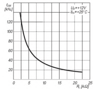
Bild 2: Abhängigkeit des Mute-Ansprechhubs vom Lastwiderstand zwischen Pin 7 und 10
