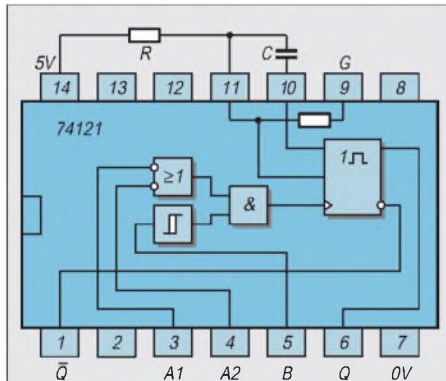
Bild 13: Pinning und Innenschaltung des monostabilen Kippschaltglieds SN 74121 N aus der TTL-Familie mit seiner äußeren Beschaltung durch ein RC-Glied.
