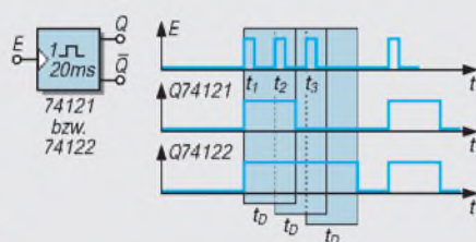
Bild 20: Vergleich der Ausgangssignale beim nicht-nachtrIGGERbaren 74121 und dem nachtrIGGERbaren 74122.
