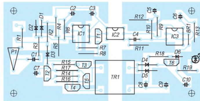
Bild 4: Platinenlayout
