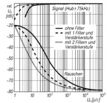
Bild 5: Begrenzungs- und Rauschverhalten
