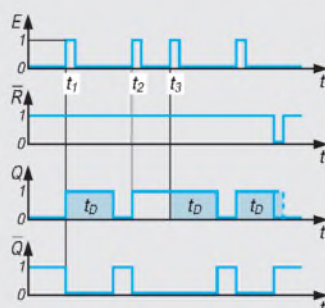
Bild 21: Ausgangssignale bei nachtriggerbarem Monoflop und Verwenden des Clear-Impulses am 0-aktiven Rücksetzeingang.
