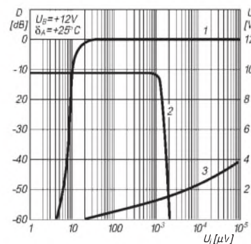
Bild 3: Wiederhergestelltes Audiosignal (1), AGC-Gleichspannung zwischen Pin 13 und 15 (2) sowie Spannung für die Abstimmanzeige an Pin 13 (3) über der Eingangsspannung
