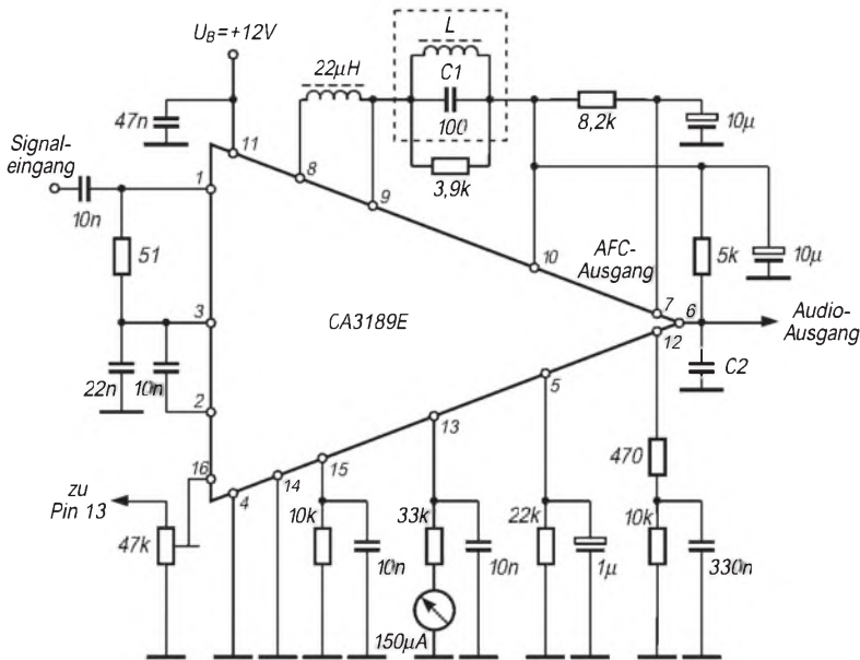
Bild 7: Test- und Einsatzschaltung mit einfacher Abstimmung durch L und C1 für 10,7 MHz ZF
