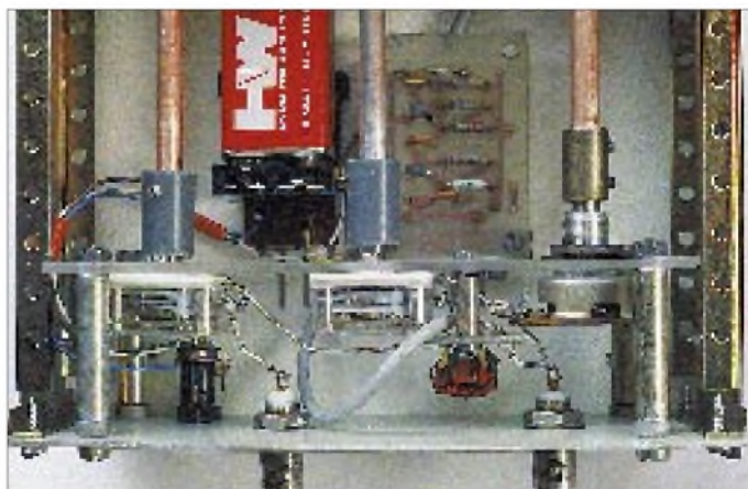
Bild 5: Blick in das Gerät. Das Potentiometer und die beiden Drehkondensatoren sind auf einer Acrylplatte isoliert montiert. Die Drehkondensatorachsen erhielten isolierte Achskuppelungen. Die Freiluftverdrahtung ist deutlich erkennbar. Fotos: Autor
