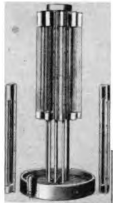
Eine neue amerikanische Riesen-senderöhre, die während des Betriebes dauernd an der Vakuumpumpe hängt
