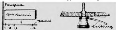
Abb. 1 und 2. Die Gitterbatterie wird verkehrt auf die Stöpsel gestülpt, die von unten durch die Montageplatte durchgehen u. gleichzeitig so die Batterie halten.
