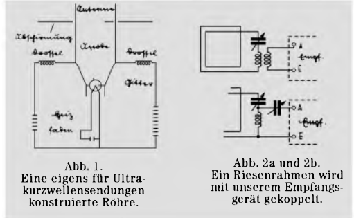
Abb. 1. Eine eigens für Ultrakurzwellensendungen konstruierte Röhre. Abb. 2a und 2b. Ein Riesenrahmen wird mit unserem Empfangsgerät gekoppelt.
