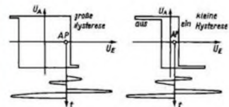
Bild 5.19: Arbeitspunkteinstellung am Schmitt-Trigger
