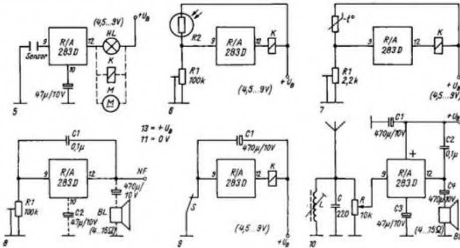
Bild 5: Sensorschalter
