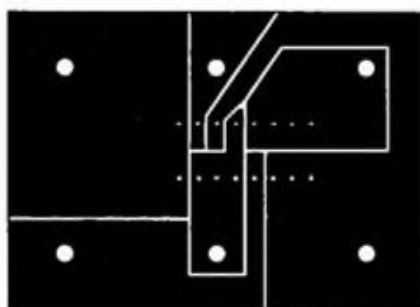
Bild 2: Leiterführung der Platine für das A-283-Modul (55 mm x 40 mm)
