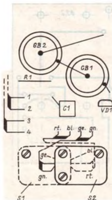
Bild 21: Bestückungsplan der Leiterplatte nach Bild 20
