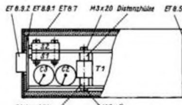
Bild 30: Anordnung der Uhrenfunktionseinheit im Gehäuse
