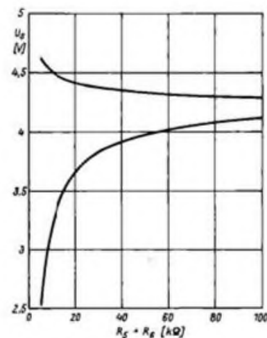
Bild 2: Die Abhängigkeit der Umschaltspannungen von R_5 + R_6
