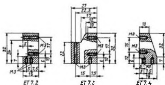
Bild 26: Baugruppe BG8 „Gehäuse“
