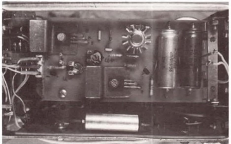
Bild 3: Blick von rechts in das Gerät auf die Platine der Dualspannungsquelle für die Stromversorgung von Operationsverstärkern
