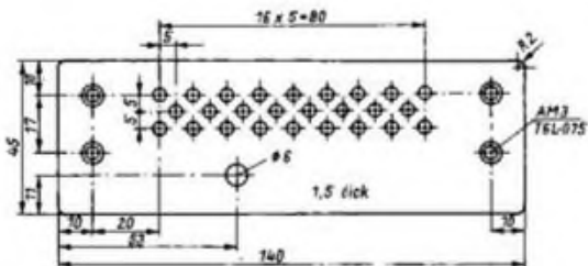
Bild 29: Einzelteil ET 8.7. „Rückwand“
