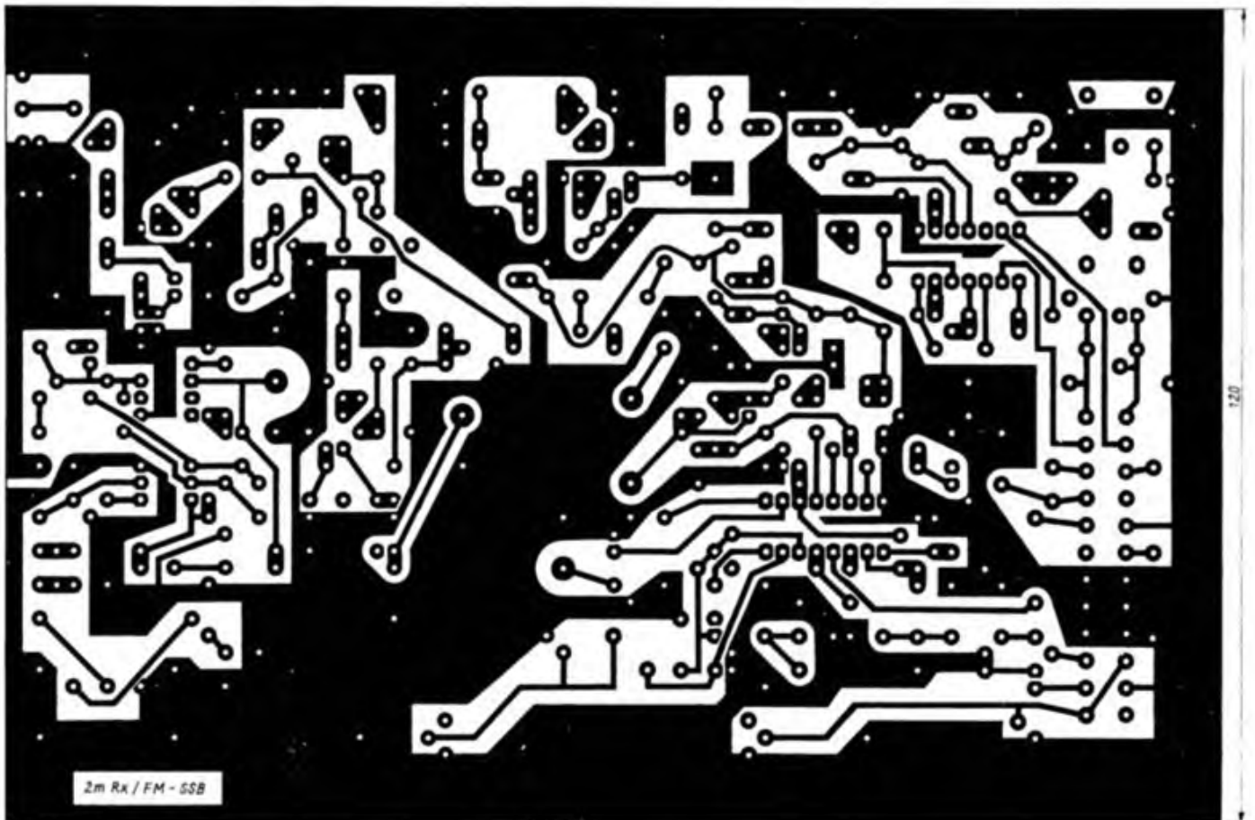
Bild 10: Leitungsführung der Platine für den Empfänger 800403
