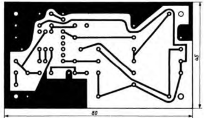
Bild 5: Leitungsführung der Leiterplatte 2 für die NF-Endstufenschaltung des Spielzeug Radios
