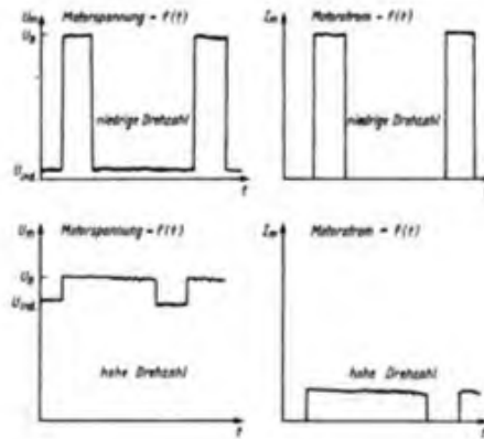
Bild 4: Oszillogramme zur Verdeutlichung der Funktionsweise (qualitativ)
