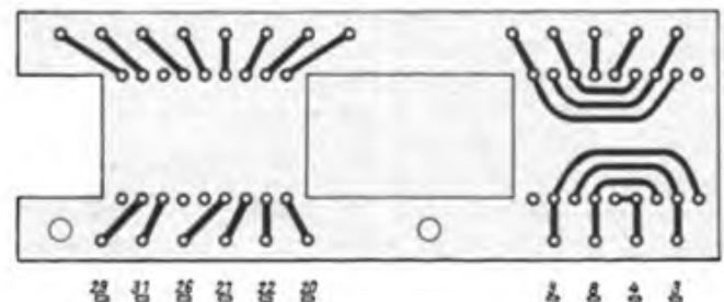
Bild 13: Bestückungsplan der Leiterplatte C
