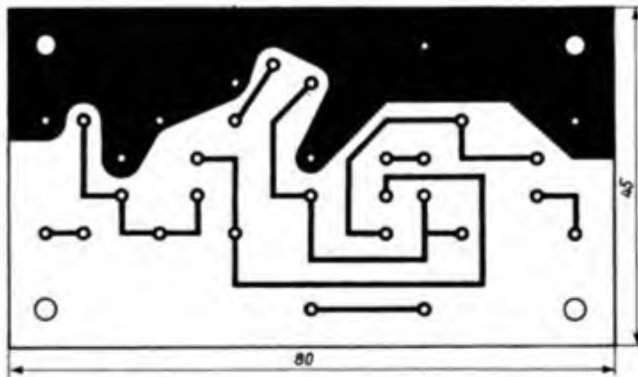
Bild 3: Leitungsführung der Leiterplatte 1 für HF Demodulator und NF-Verstärker
