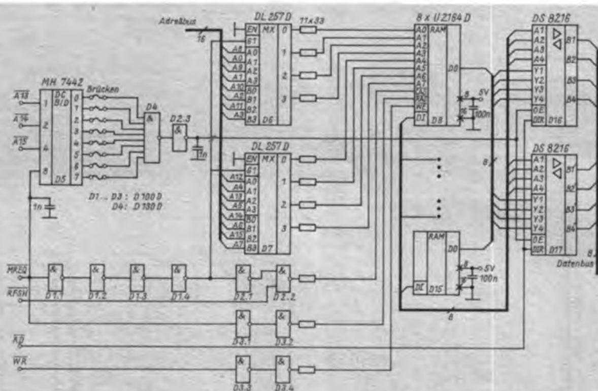
Bild 2: Stromlaufplan der beschriebenen Speichererweiterung für den Amateurcomputer „AC 1“
