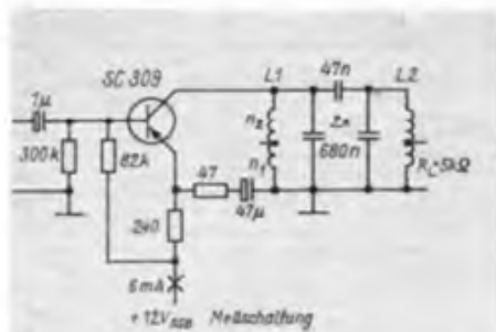
Bild 13: Stromlaufplan eines LC-Filters für Telegrafie-Empfang
