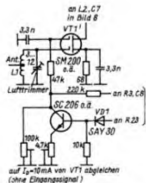
Bild 9: Vorstufenstromlaufplan im Einsatz eines Dual-Gate-FET mit zusätzlichem Regeltransistor L1 = 8,5 Wdg.; 1-mm-CuL auf 6-mm-Dorn, Anzapfung 1 Wdg. vom kalten Ende
