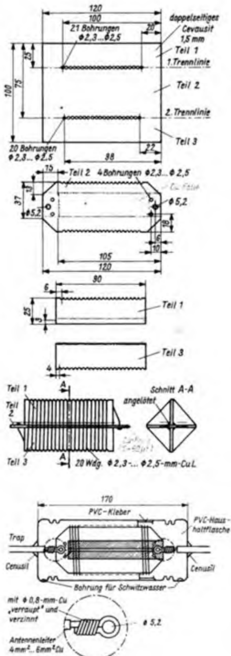
Bild 1: Die Abmessungen des Cevauststücks für einen Trap, darunter die der Einzelteile (Spulenkörper und Folienkondensator)
