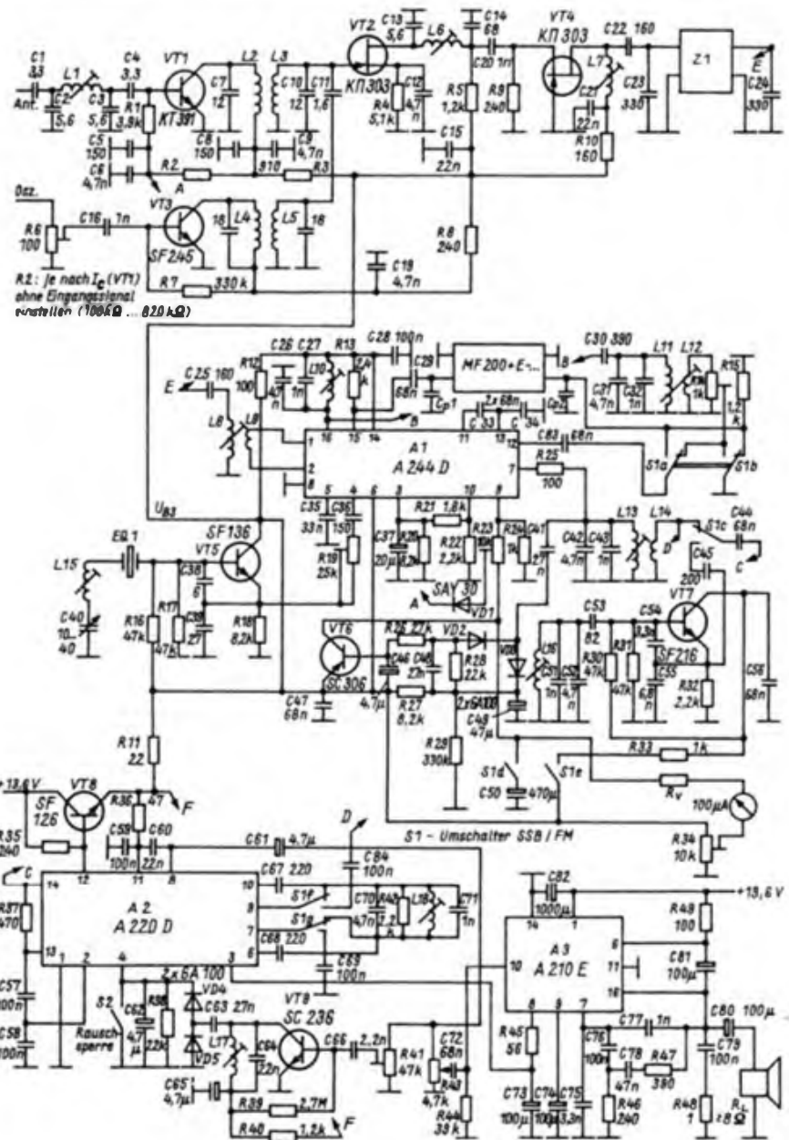
Bild 8: Stromlaufplan des 2-m-Doppelsupers 800403
