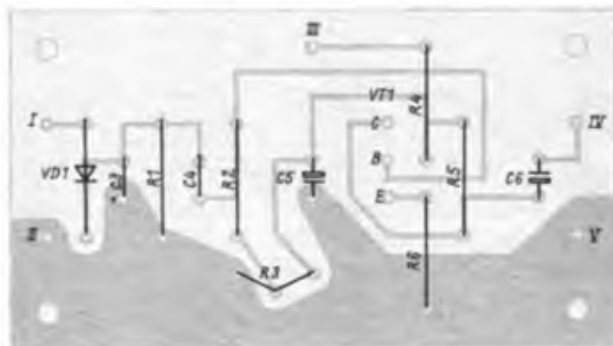
Bild 4: Bestückungsplan für die Leiterplatte 1 (Demodulator und NF-Verstärker)
