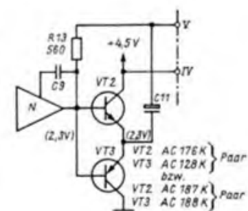
Bild 2: Eine andere Schaltungslösung verwendet Germaniumtransistoren in der NF-Endstufe des Spielzeug Radios
