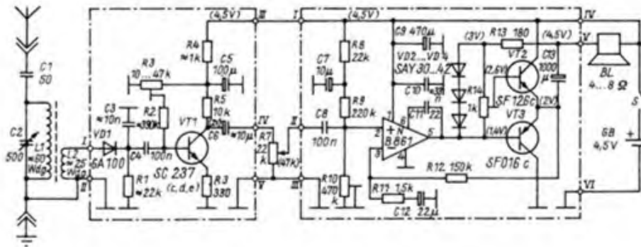
Bild 1: Gesamtschaltungsaufbau des Spielzeug-Radios, für dessen Aufbau zwei Platinen vorgesehen sind
