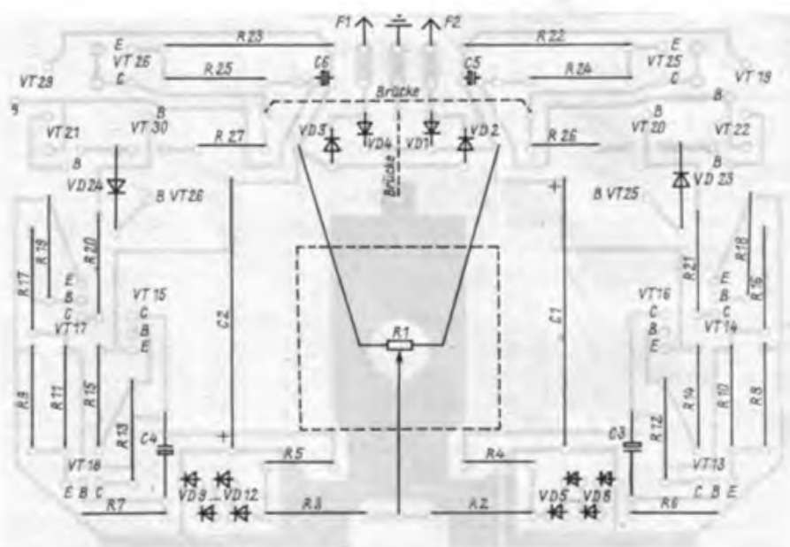
Bild 3: Bestückungsplan der Leiterplatte. Das Potentiometer wird direkt auf der Leiterplatte montiert und über kurze Litzen angeschlossen.
