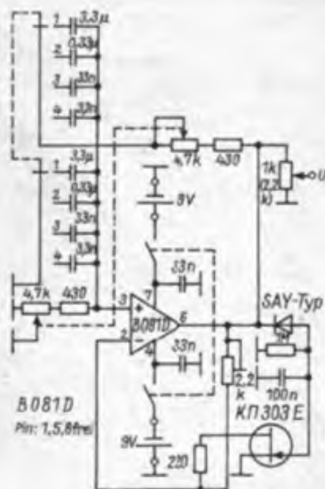
Bild 11: Wienbrückengenerator mit einstellbarer Frequenz und Amplitude
