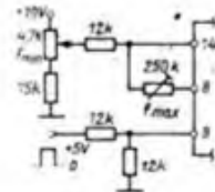
Bild 5: Beschaltung des IA 338 D zur Frequenzumtastung
