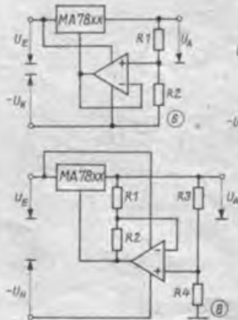
Bild 6: Durch eine negative Hilfsspannung kann U_A verringert werden
