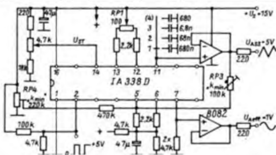
Bild 6: Verbesserter Funktionsgenerator mit BifET-OV-Ausgangsstufen für 20 Hz bis 200 kHz
