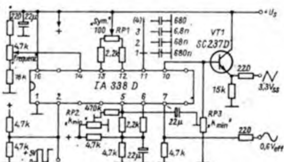
Bild 4: Einfacher Funktionsgenerator über 4 Dekaden ( R_{P1} = 100 k\Omega )
