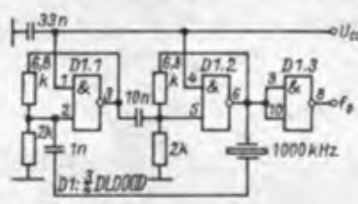
Bild 7: Einfacher RC-TTL-Generator
