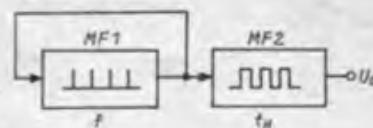
Bild 1: Prinzip eines Impulsgenerators für Prüfzwecke
