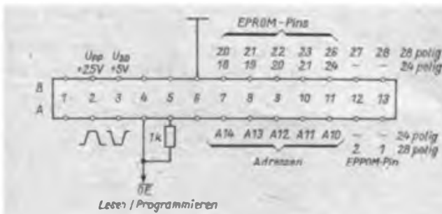
Bild 2: Beschaltung des Programmiersteckers
