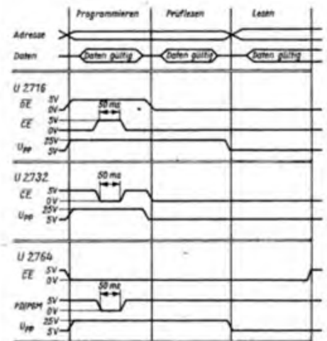
Bild 3: Impulsdigramme des Programmiervorgangs
