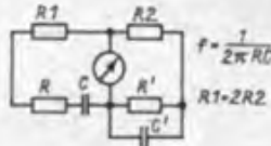
Bild 10: Prinzip der Wienbrücke
