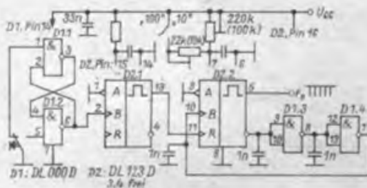
Bild 2: Ausgeführte Schaltung eines Impulsgenerators
