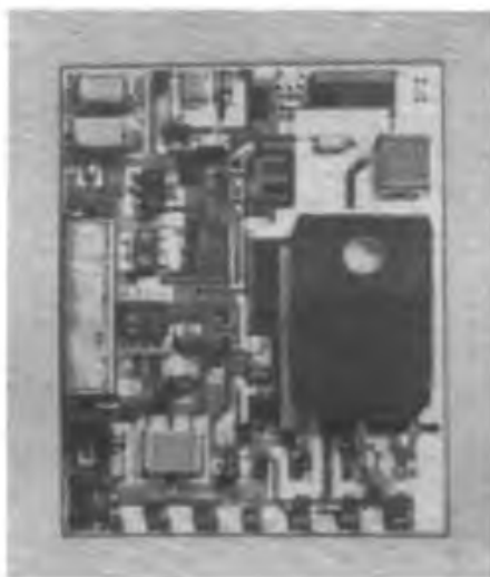
SMD-Technologie in der Anwendung – die elektronische Zündanlage ESE 4 H (VEB Kombinat Keramische Werke Hermsdorf), u. a. auch im Wartburg 1.3 eingesetzt
