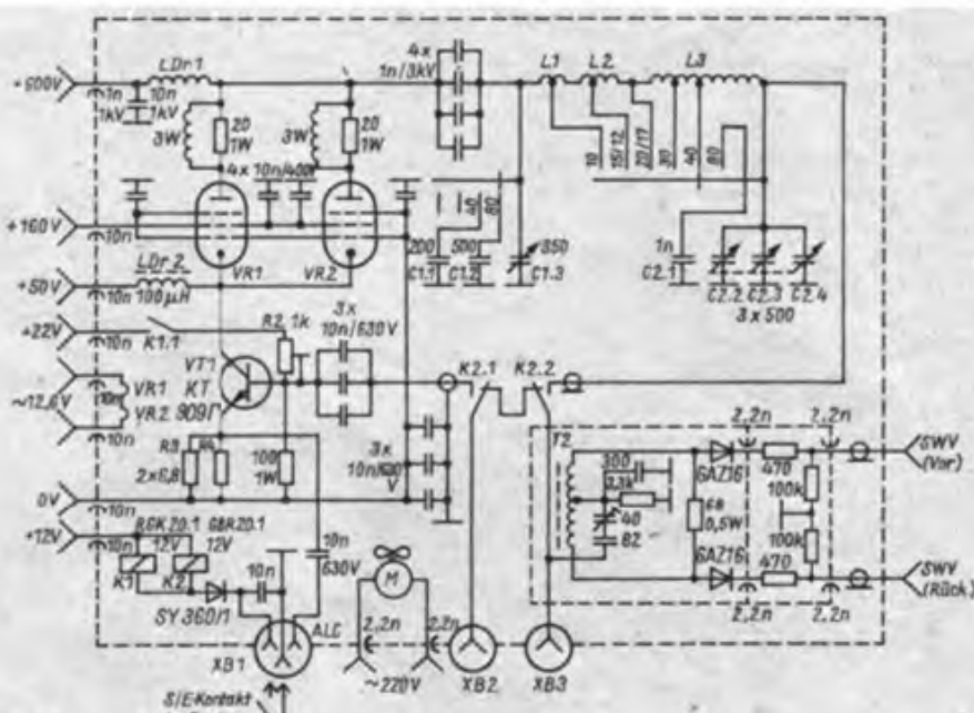
Bild 4: Stromlaufplan des HF-Teils der Endstufe
