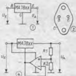
Bild 1: Grundschematische Stromlaufpläne
