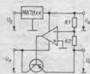
Bild 11: Erzeugung einer negativen Ausgangsspannung, deren Betrag von der positiven abweichen kann
