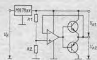
Bild 11: Erzeugung einer negativen Ausgangsspannung, deren Betrag von der positiven abweichen kann
