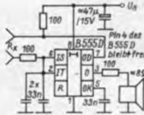
Bild 9: Akustische Prüfschaltung für Widerstände
