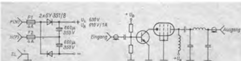
Bild 1: Spannungsverdopplung direkt aus dem Netz
