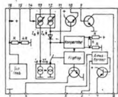
Bild 1: Prinzipinnenschaltung
