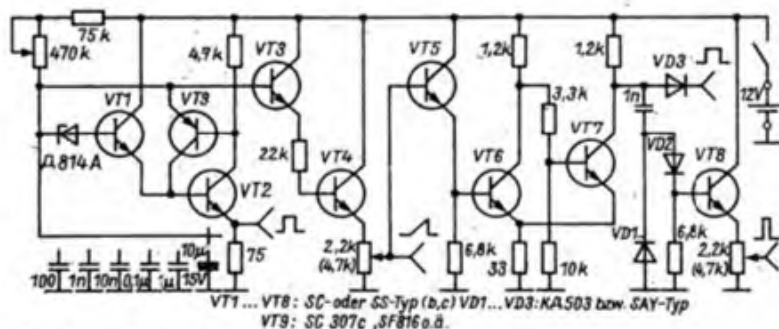
Bild 6: Universeller Signalgenerator mit Transistoren [2]
