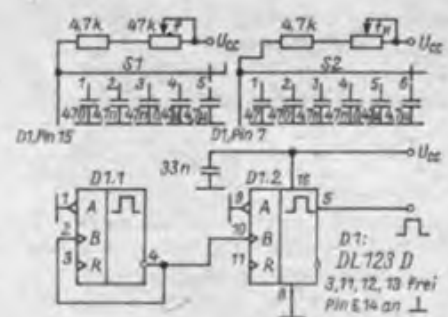
Bild 1: Prinzip eines Impulsgenerators für Prüfzwecke
