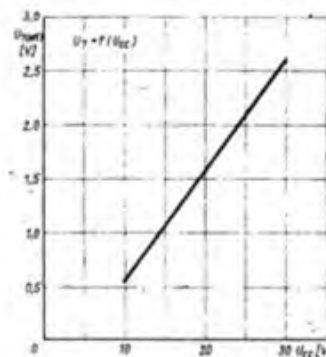
Bild 12: Ausgangsspannung des Sinusformers als Funktion der Betriebsspannung
