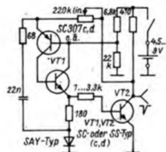
Bild 5: Nadelimpulsgenerator nach [1]
