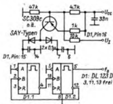
Bild 4: Ein vielseitig nutzbarer VCO nach [1]
