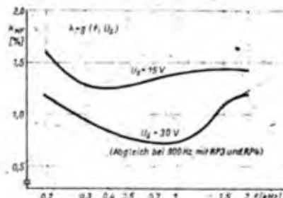
Bild 3: NF Klirrfaktor der Grundscharlung nach Bild 2 bei 1 kHz
