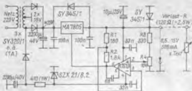
Bild 9: Stromlaufplan für ein wenig aufwendiges Experimentiernetzteil mit dem Festspannungsregler MA7805. Als OV kommt ein B 761 D zum Einsatz.
