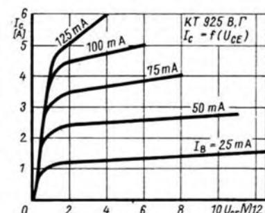
Bild 9: Ausgangskennlinienfeld der Transistoren KT 925 B und KT 925 Γ
