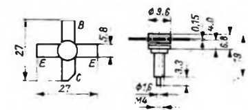
Bild 1/2: Maßbild und Anschlußbelegung
