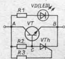
Bild 3: Grundstromlaufplan der elektronischen Sicherung
