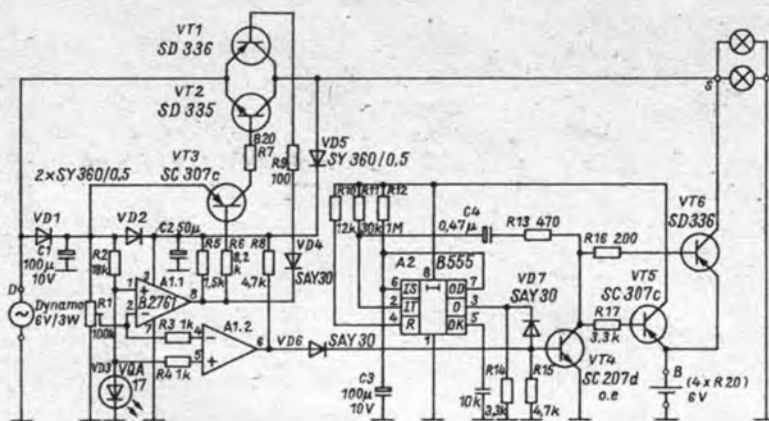
Bild 1: Stromlaufplan der Umschaltelektronik
