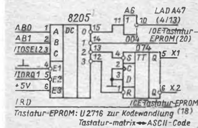
Bild 2: Stromlaufplan der Zusatzschaltung zum Anschluß einer ASCII-Tastatur an den Z 1013
