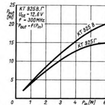
Bild 12: Ausgangsleistung als Funktion der Eingangsleistung beim KT 925 B und KT 925 Γ
