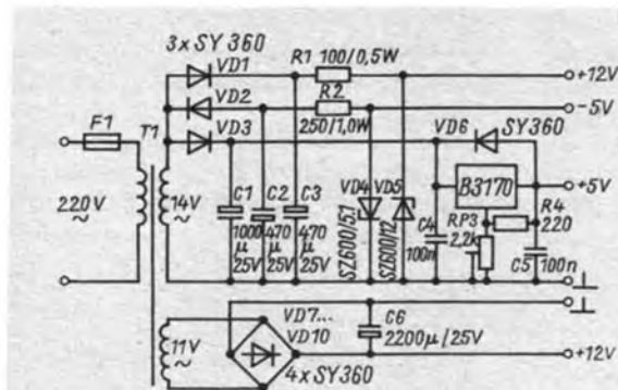
Bild 4: Stromlaufplan des Netzteils, das auch die zusätzlichen Betriebsspannungen zum Einsatz von 1-K-EPROMs erzeugt
