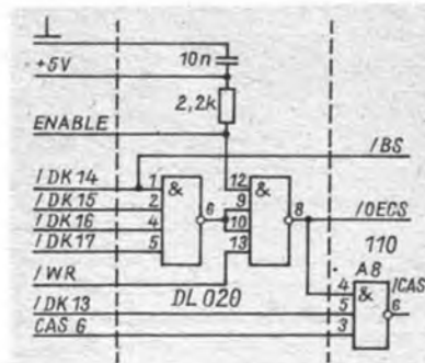
Bild 1: Stromlaufplan der Zusatzschaltung zur Abschaltung des Monitor-ROMs
