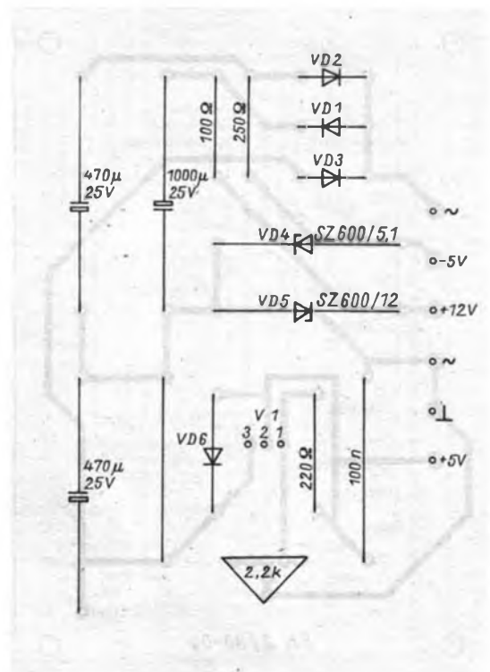
Bild 6: Bestückungsplan der Netzteilplatte
