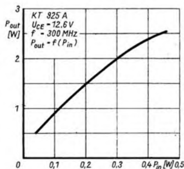
Bild 10: Ausgangsleistung als Funktion der Eingangsleistung beim KT 925 A
