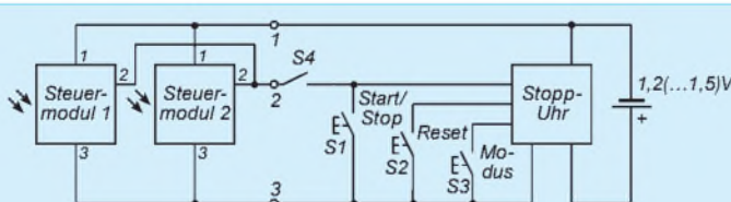
Bild 10: Experimentiervorschlag: Doppellichtschranke zur Zeitnahme mit Taster für definierten Anfangszustand und Erweiterungsmöglichkeit für Zwischenzeiten. „Steuer-modul“ siehe Bild 9, neu dargestellt sind nur die Ergänzungen
