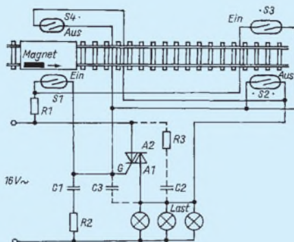
Bild 15: Anwendungsbeispiel der Schaltung nach Bild 14. SRKs - durch Magnete in Fahrzeugen betätigt - können Verbraucher ein- und ausschalten. ( R1 = 100\Omega , R2 = 560\Omega , R3 = 47\Omega , alle 0,5W ; C1 = 1\mu F/63V , C2, C3 = 0,1\mu F/100V )
