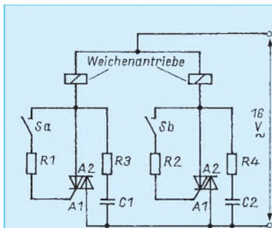
Bild 12: Stromlaufplan für einen Weichenantrieb ( R1, R2 = 1k\Omega/0,5W ; R3, R4 = 47\Omega/0,5W ; C1, C2 = 0,1\mu F/100V )
