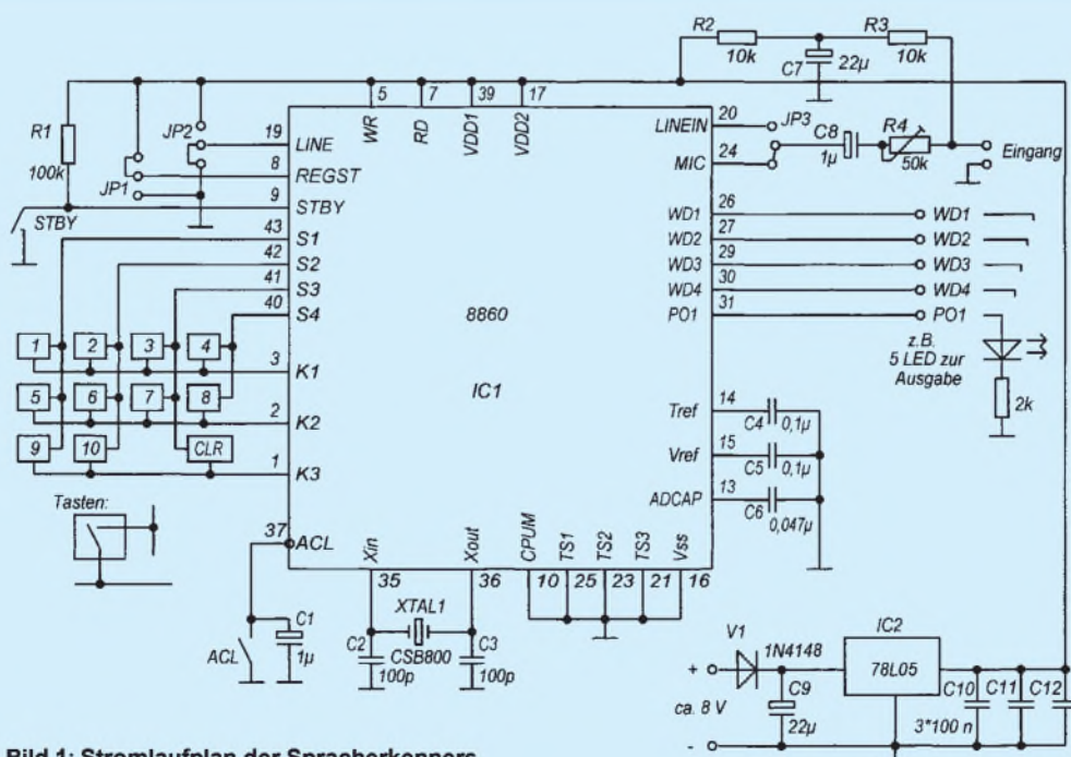
Bild 1: Stromlaufplan der Spracherkenners
