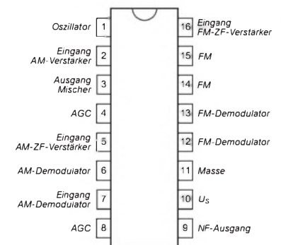
Bild 1: Pinbelegung
