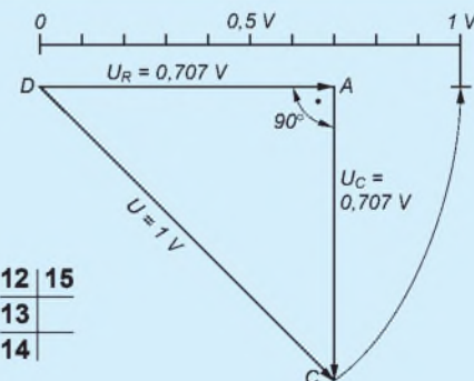
Bild 12: Mit konstanter Frequenz gespeister Phasenschieber
