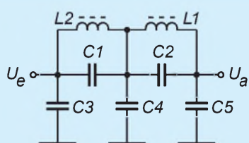
Grundschialtung des Antennen-Tiefpaß-filters; die Dimensionierung erfolgt nach Tabelle
