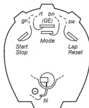
Bild 3: Adaptieren der Steuereingänge einer Billig-Stoppuhr mit eingesteckten 0,3- bis 0,5-mm-Messing- oder Leiterplattenhalbeingangsplättchen sowie thermisch eingeführter Minusanschluß in der Batteriekammer
