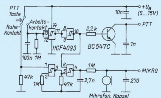
Stromlaufplan des Rogerpiep mit dem CMOS-Schaltkreis 4093
