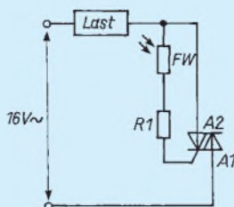
Bild 13: Der Triac als lichtgesteuerter Schalter. Fällt Licht auf den Foto-Widerstand FW, so zündet der Triac für die Dauer des Lichteinfalls.
