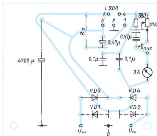
Bild 3: Layout der Leiterplatte für die 2-A-Version für 3 bis 24 V (Maßstab 1:1). Die Bohrungen sind anzukennzeichnen.
