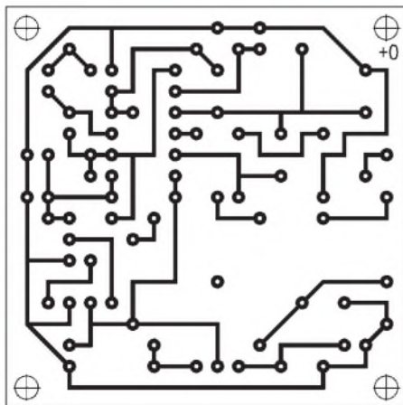
Bild 4: Platinenlayout
