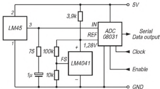
Bild 7: Ausgabe der Temperatur als seriellen Datenstrom durch einen A/D-Wandler. Der Einsatztemperatur- bzw. Anzeigebereich beträgt 0 bis 128 °C.
