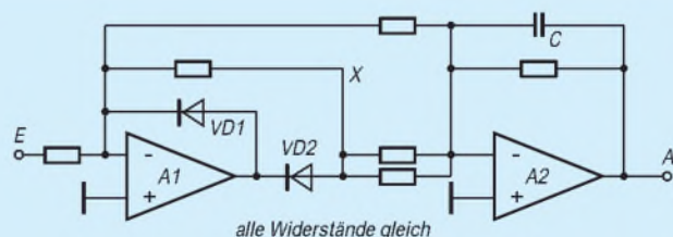
Bild 2: Prinzip des Präzisionsgleichrichters mit OV
