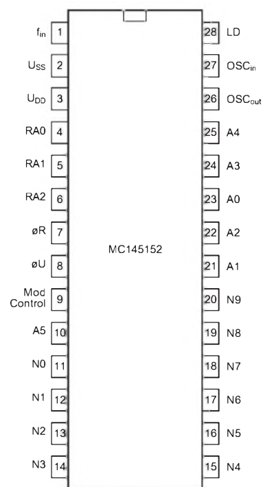
Bild 1: Pinbelegung des DIL-Gehäuses
