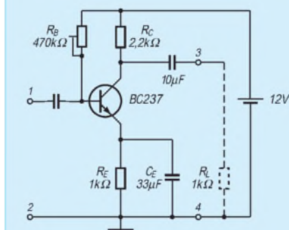
Bild 6: Transistorstufe mit einfachem Vorwiderstand R_B zur Einstellung des Arbeitspunkts.
