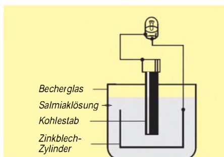
Bild 2: Unsere Spannungsquelle
