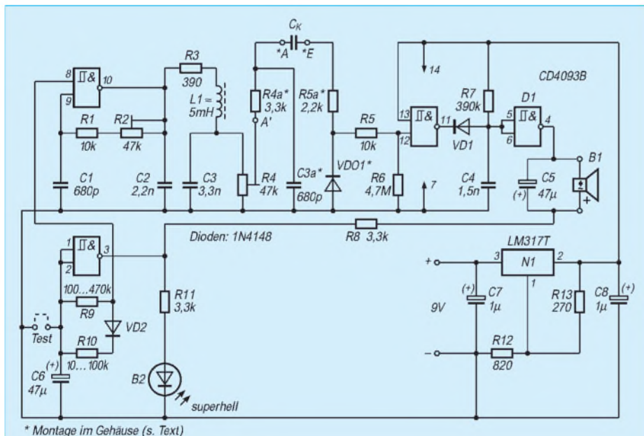
Bild 3: Gesamtschaltung mit periodischer Einschaltung, Aktivsignal per LED und Trockenwarnung über Piezo-Generator
