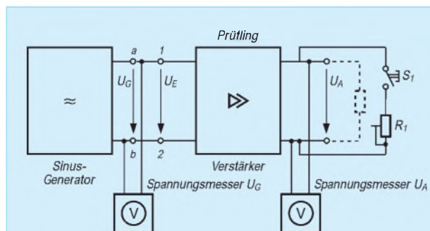
Bild 7: Meßschaltung zur Ermittlung des Ausgangswiderstands von aktiven Schaltungen.
