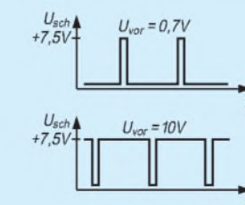
Bild 3: Impulsdiagramm der Ausgangsspannung des Dreieckspannungsgenerators mit dem OV A3c, gemessen am Punkt 1 (Bild 5)
