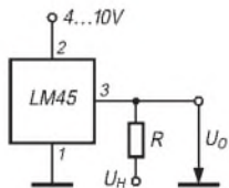
Bild 4: Schaltung für Messungen ab -20 °C mit negativer Hilfsspannung ( R = U_H / -50\text{ }\mu\text{A} )
