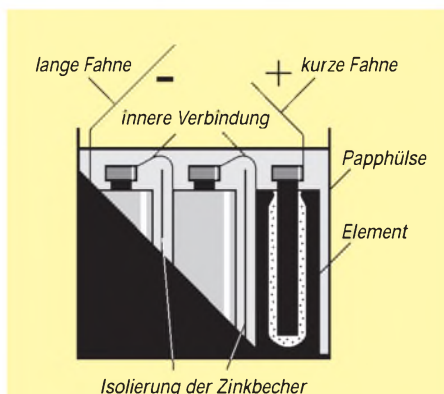
Bild 1: Flachbatterie
