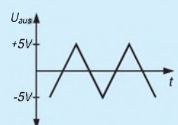
Bild 4: Impulsdiagramm der Steuerspannung für die CMOS-Analogschalter, gemessen am Punkt 2 (Bild 5), in Abhängigkeit von U_{\text{vor}}
