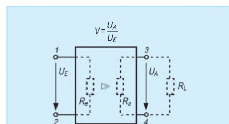
Bild 2: Blockschaltbild eines Verstärkers allgemein mit seinem Eingangswiderstand R_e und seinem Ausgangswiderstand R_a .
