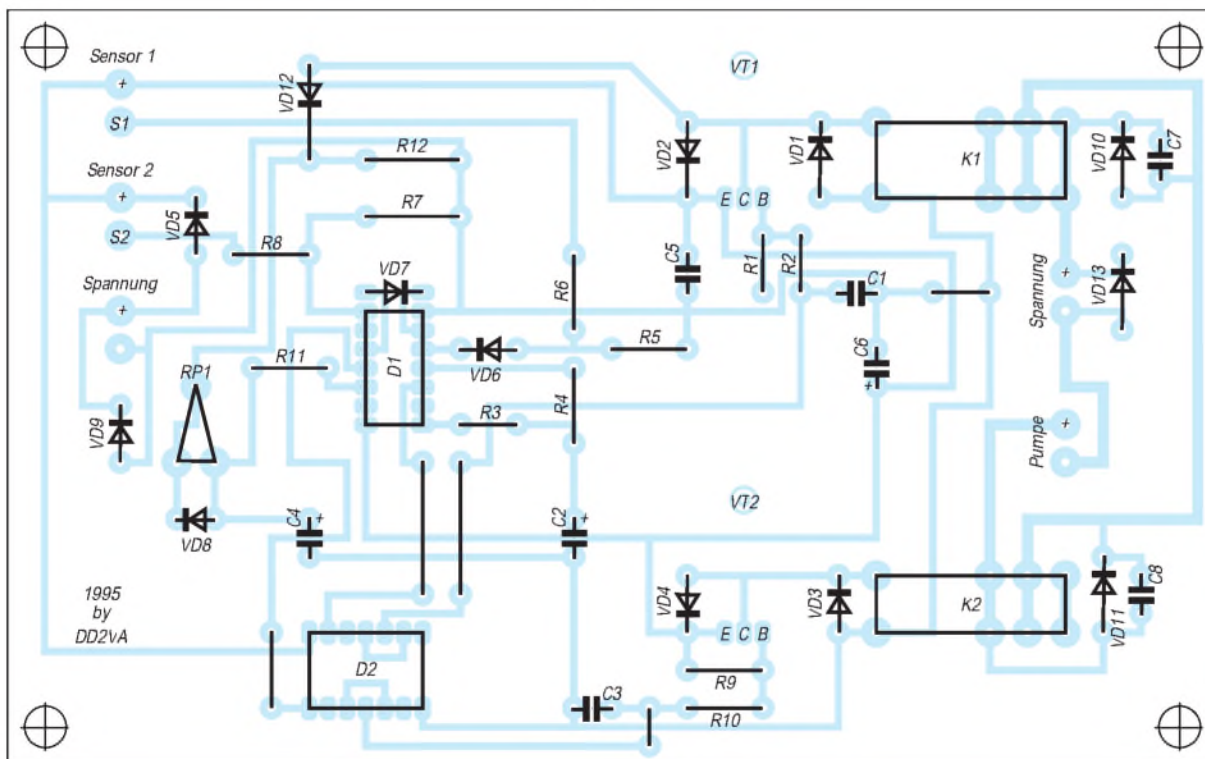
Bild 3: Platinenlayout
