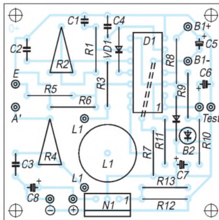
Bild 5: Bestückungsplan
