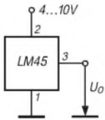
Bild 3: Schaltung für Messungen ab 2,5 °C
