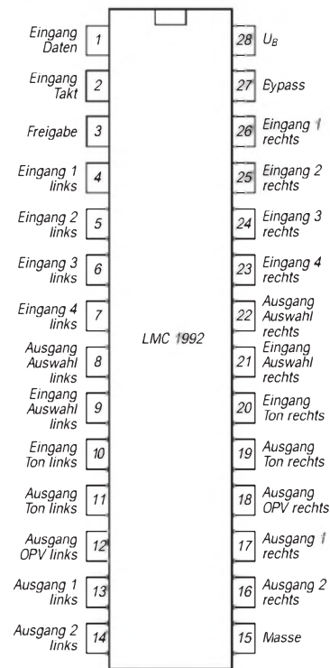
Bild 2: Anschlußbelegung
