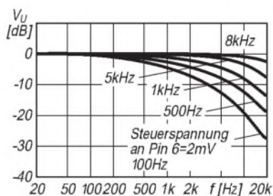
Bild 2: Frequenzabhängigkeit der Bandbreite bei konstanter Steueramplituden
