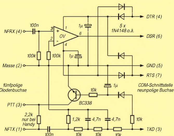
Bild 10: Simplen-Modem nach DL2JTT
