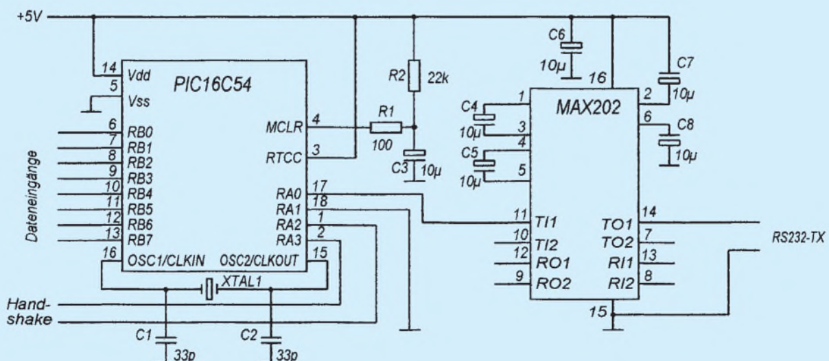
Bild 1: Beispiel für die Verwendung des PIC 16C54 als asynchroner serieller Senderschaltkreis
