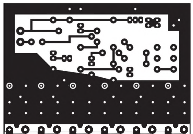
Selektiver HF-Verstärker (Preselektor) für Kurzwellen FA 10/95, S. 1086
