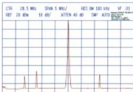
Nah-Nebenaussendungen bei 28,500 MHz, gemessen mit 30 dB Vordämpfung.
