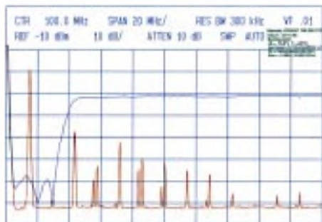
Nebenaussendungen bei einer Nutzfrequenz von 14,25 MHz, gemessen mit 30 dB Vordämpfung und Hochpaßfilter; Referenz ist die blaue Kurve des Hochpasses!
