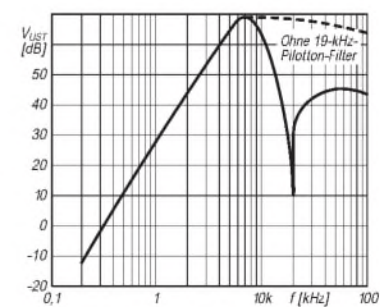
Bild 4: Frequenzabhängigkeit der Verstärkung des internen Spannungverstärkers mit und ohne Pilottonfilterbeschaltung
