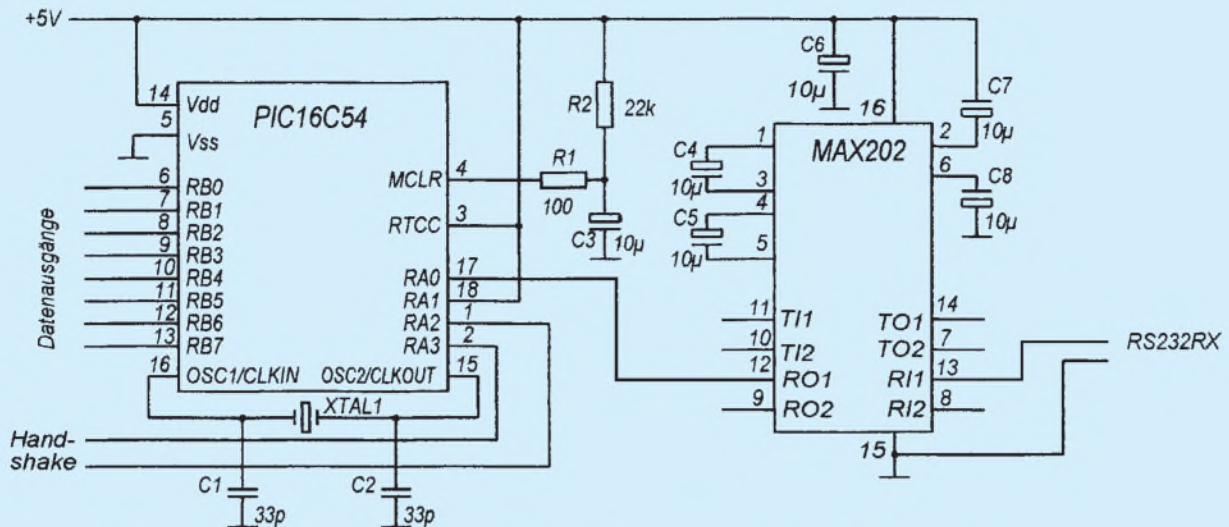
Bild 2: Beispiel für die Verwendung des PIC 16C54 als asynchroner serieller Empfängerschaltkreis
