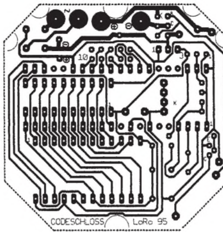
Bild 2: Platinenlayout
