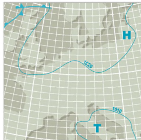
Die Wetterkarte vom 29.7.95 zeigt ein ausgedehntes Hoch über der Ostsee.
