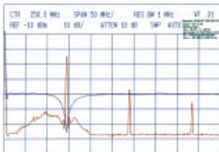
Nebenaussendungen bei einer Nutzfrequenz von 145,000 MHz, gemessen mit 20 dB Vordämpfung und Notchfilter; Referenz ist die blaue Kurve des Notchfilters!
