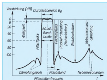
Bild 1: Typische ZF-Filter-Durchlaßkurve
