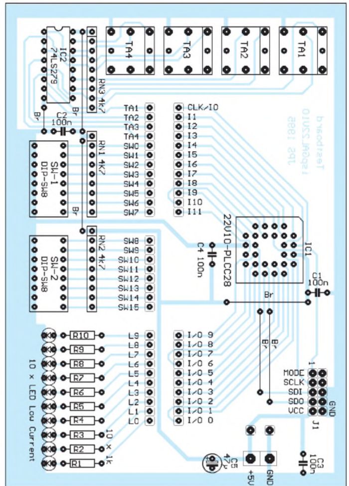
Bild 7 : Bestückungsplan für das Test- und Entwicklungsboard
