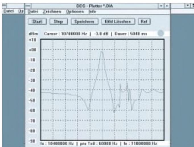
Bild 1: So erfolgen Darstellung und Ausdruck von Meßkurven im Programm DIAG4
