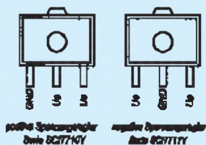
Bild 2: Die Serie SCI 7710 und 7711 wird im SOT-89-Gehäuse hergestellt
