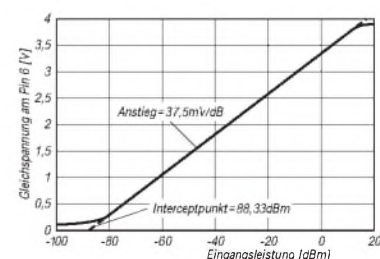
Bild 2: Typischer Verlauf der Übertragungsfunktion
