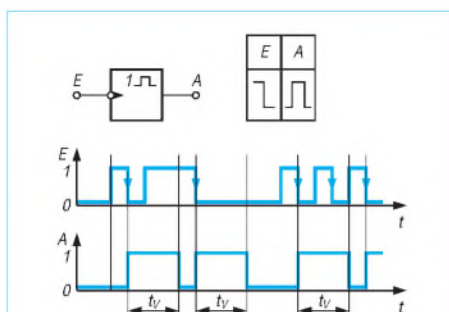
Bild 6: Genormtes Schaltzeichen, Signal-Zeit-Diagramm und Triggertabelle für ein mit negativer Flanke gesteuertes, nichtnachtrigbares Mono-Flop.
