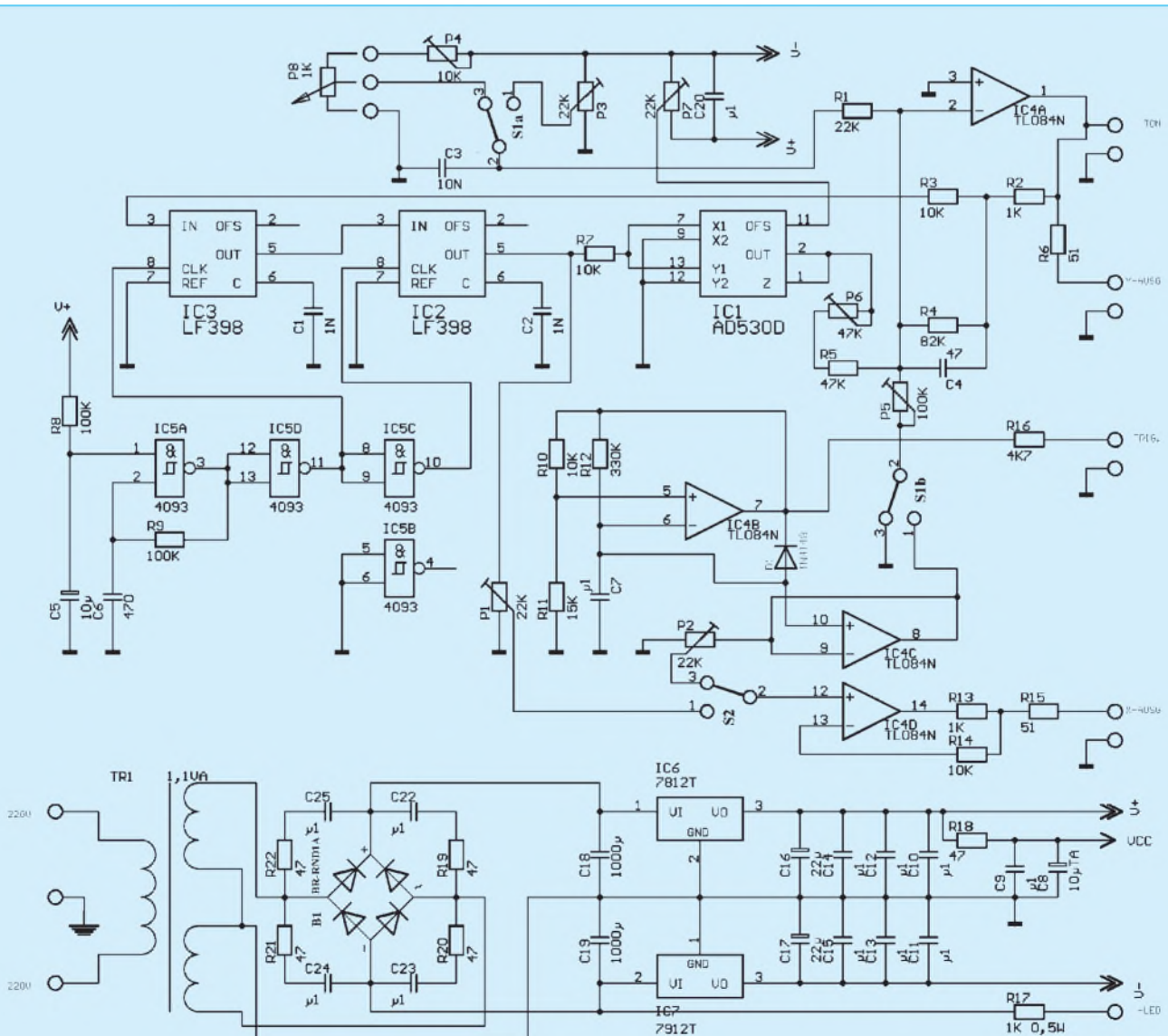
Bild 1: Stromlaufplan des Chaos-Generators
