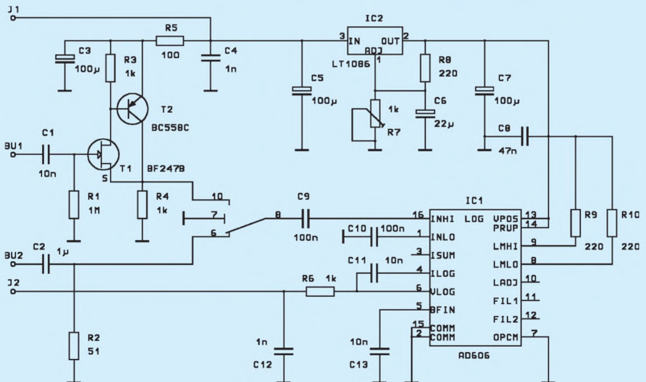
Bild 2: Die Schaltung des logarithmischen Meßverstärkers LOG1
