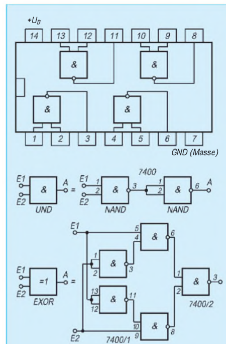
Bild 5: Schaltungen eines mit dem NAND-Baustein 7400 aufgebauten UND-Glieds (oben) und eines EXOR-Glieds (unten).
