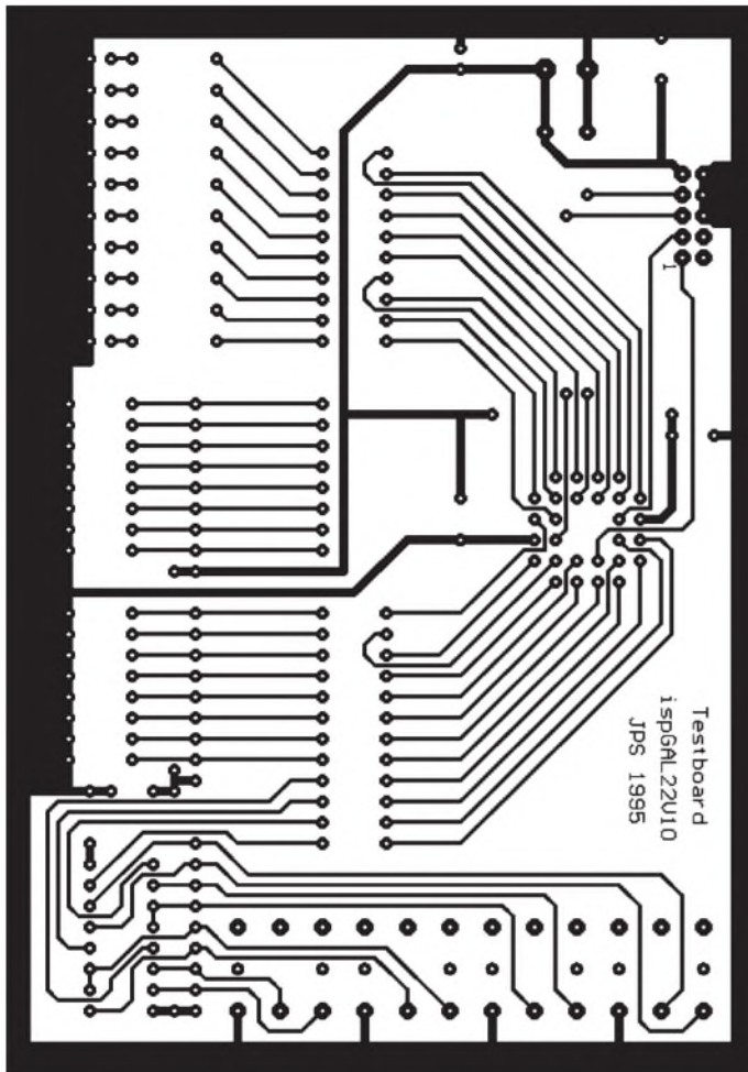
Bild 6 : Leiterplattenvorschlag für das Test- und Entwicklungsboard
