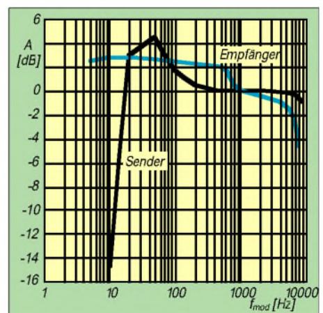
Bild 3: Frequenzgang von Senders (Einspeisung in die DATA-Buchse) und Empfänger, bei einem Hub von 1 kHz
