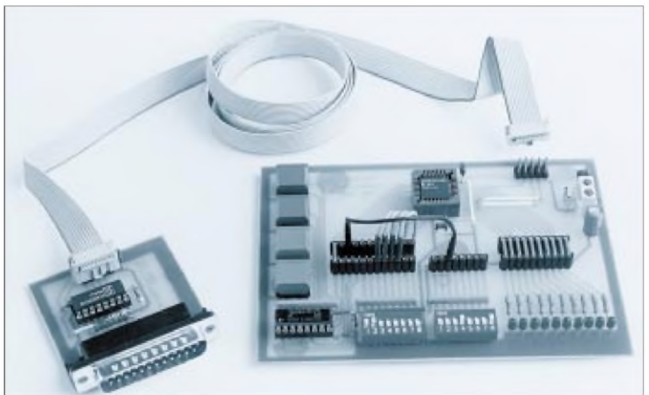
Bild 8: Das komplette Experimentier-Set
