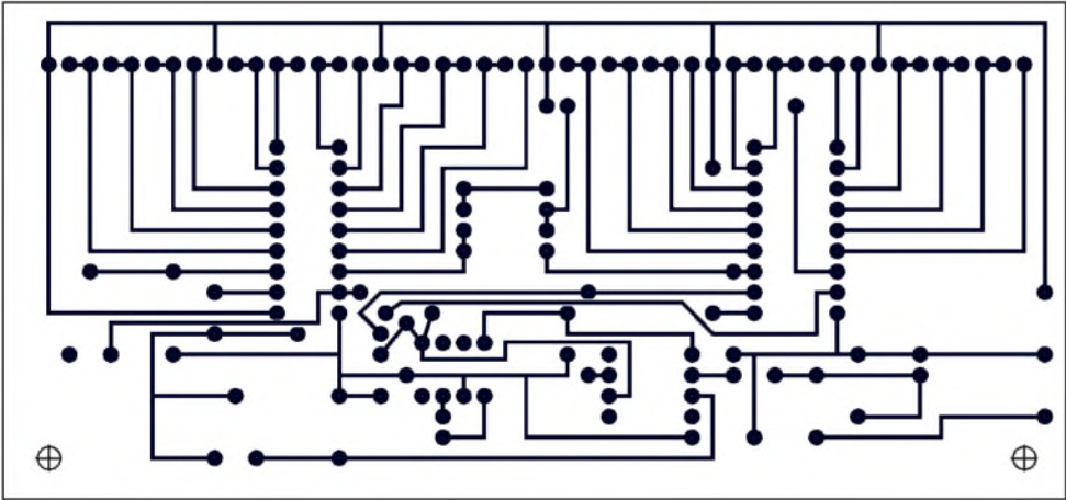
Bild 2: Leiterplattenlayout
