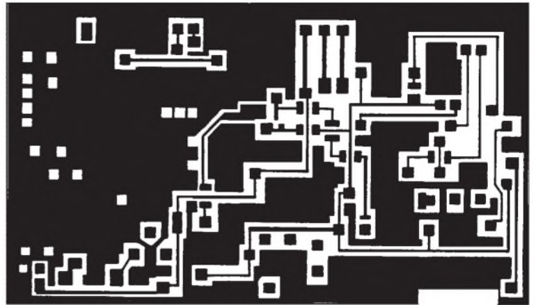
Bild 2: Leitungs- führung der Platine für die Haupt- baugruppe (Oberseite)
