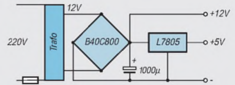
Bild 3: Stromlaufplan des Timer-Moduls
