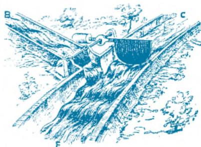
Auch in die Transistor-Zeit wurde das bildhafte Prinzip hinübergerettet. Der Strom im Kanal B (Basis) kann den ungleich stärkeren Strom von C nach E (Collector/Emitter) im selben Rhythmus beeinflussen – der Transistor als Verstärker.
