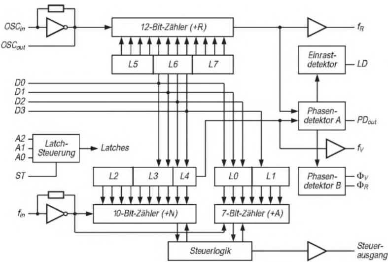
Bild 1: Innere Struktur des PLL-Frequenzsynthesizer-Schaltkreises mit drei diversen Teilern und Datenbus für Strobesignal (ST) und Adressen (A0 ... A2)
