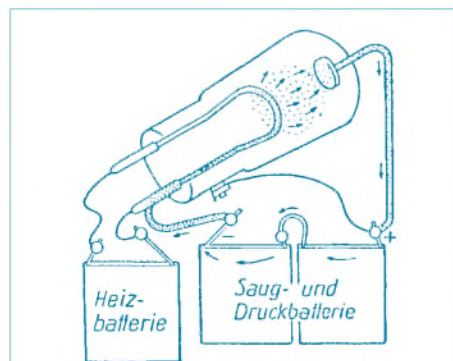
So war die Röhre leicht zu verstehen: Dieses Bild zeigt instruktiv, wie der Elektronenfluß zwischen Heizfaden und Anode zustandekommt.
