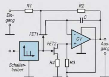
Bild 5: Grundsaltung eines Sample/Hold-Schaltkreises mit nur einem Operationsverstärker und Feldeffekt-Transistoren als Schalter zur Umsteuerung.
