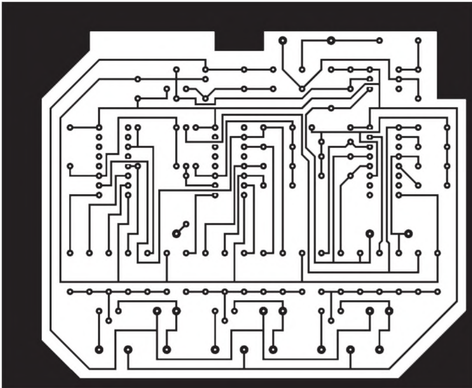
Bild 2: Platinenlayout
