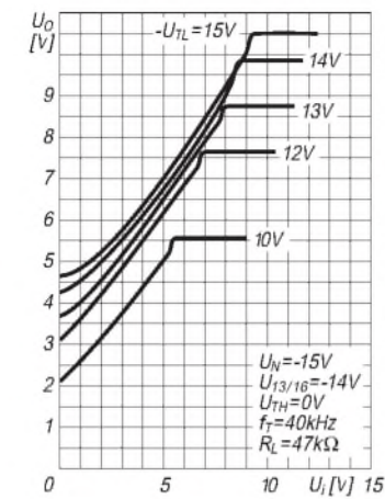
Bild 2: Zusammenhang zwischen Ein- und Ausgangsspannung mit der L-Taktspannung als Parameter
