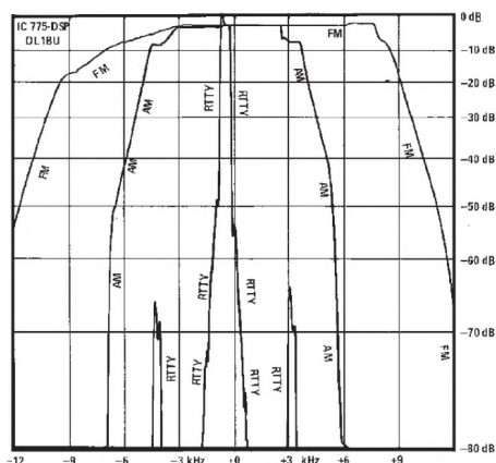
Bild 11: Gesamtselektion FM, AM und RTTY der Standardbestückung
