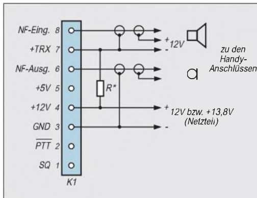
Bild 6: Beispiel für eine Zusammenschaltung von Papagei und 12-V-Handy bei Nutzung der Stromsensor-Trägererkennung. R14 muß in diesem Fall bestückt sein oder besser extern zwischen Stift 2 und 6 von X1 gelegt werden. X3 muß gesteckt sein.
