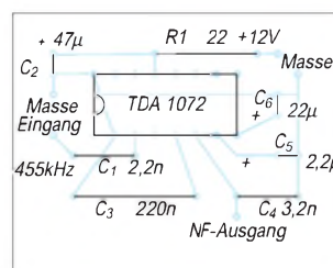
Bild 3: Bestückungsplan
