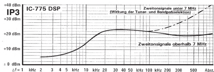
Bild 12: Eingangs-Interzeptpunkts 3. Ordnung in Abhängigkeit vom Abstand der starken (!) HF-Doppelsignale und Wirkung der Vorselektion (mit Antennenabstimmgerät) ohne Vorverstärker bei 7 MHz. Zur Messung des IP_3 wurden zwei rauscharme Meßsendersignale über einen Leistungssummierer hoher Entkopplung zusammengefügt, die Ausgangspegel wurden auf \pm 0,2 dB justiert und einer 1-dB-Stufeneichleitung zugeführt. Die Frequenzabstände wurden auf 1 kHz bis 1 MHz und der Pegel des Doppelsignals so eingestellt, daß 0,1 \mu V, 1 \mu V bzw. 10- \mu V-IM-Signale am Empfänger entstehen (-127 dBm, -107 dBm, -87 dBm). Vergleichssubstitution mit Meßsender. IP_3 = 0,5 \text{ IMA} + P_{in}
