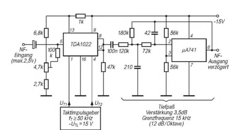
Bild 5: Typische Anwendungsschaltung des Eimerketten-Schaltkreises. Die hohe Flankensteilheit des Tiefpasses garantiert eine exakte Signalformregeneration.
