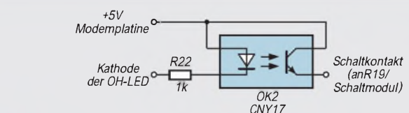
► Bild 1: Stromlaufplan des Eingangs- und Schaltmoduls
