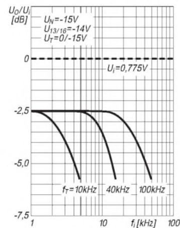
Bild 4: Frequenzgang der Verstärkung für drei Taktfrequenzen
