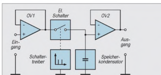
Bild 4: Schematische Darstellung der Schaltung eines Sample/Hold-Schaltkreises.
