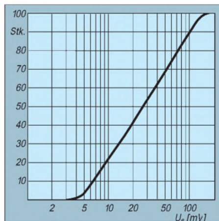
Bild 4: Anzeige (in Skalenteilen) des HF-Indikators in Abhängigkeit von der Eingangsspannung. Sie erfolgt über 35 dB recht exakt logarithmisch.
