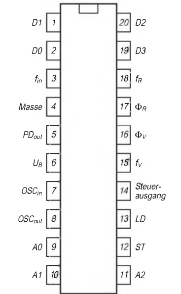
Bild 2: Anschlußbelegung des PLL-Schaltkreises
