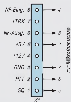
Bild 7: Zweites Beispiel für eine Zusammenschaltung von Papagei und einem FT-912 (mit „Packet-Modifikation“ lt. Handbuch) bei Nutzung von 5 V und „Busy“-Signal aus der Mikrofonbuchse. X3, R14 und A3 müssen, alle sonstigen optionalen Bauteile können unbestückt bleiben.
