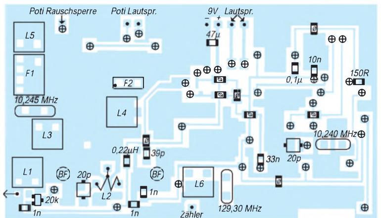
Bild 3: Bestückungs- plan der Leiterplatte der Haupt- baugruppe (Oberseite)
