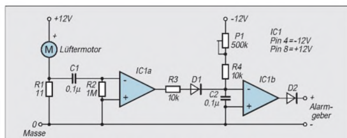
Bild 1: Stromlaufplan der Lüfterüberwachung
