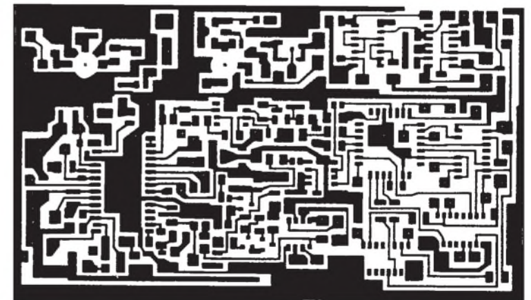
Bild 4: Leitungs- führung der Platine für die Haupt- baugruppe (Unterseite)
