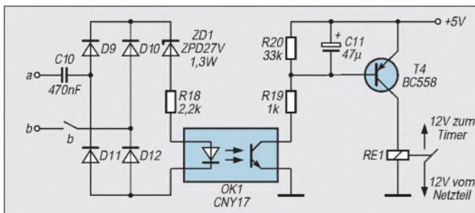
► Bild 1: Stromlaufplan des Eingangs- und Schaltmoduls
