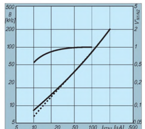
Bild 5: Meßwerte des Filters nach Bild 4
