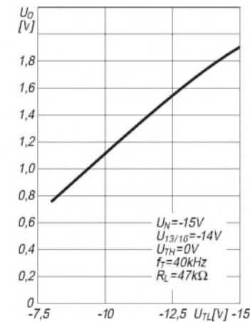
Bild 3: Abhängigkeit der Ausgangsspannung von der L-Taktspannung
