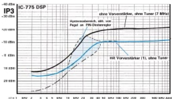
Bild 13: Verlauf des Interzeptpunktes 3. Ordnung ohne Antennenabstimmgerät, mit (obere Kurve) und ohne Vorverstärker (untere Kurve) bei schwachen Eingangssignalen, IM etwa 1 \mu V. Die Messung erfolgte wie bei Bild 12.
