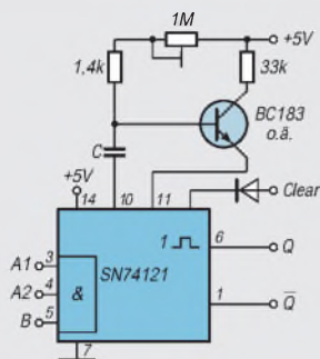
Bild 18: Mit einem Transistor erweiterte Schaltung für die Erzeugung langer Verweildauern bei Vermeidung großer Widerstandswerte.
