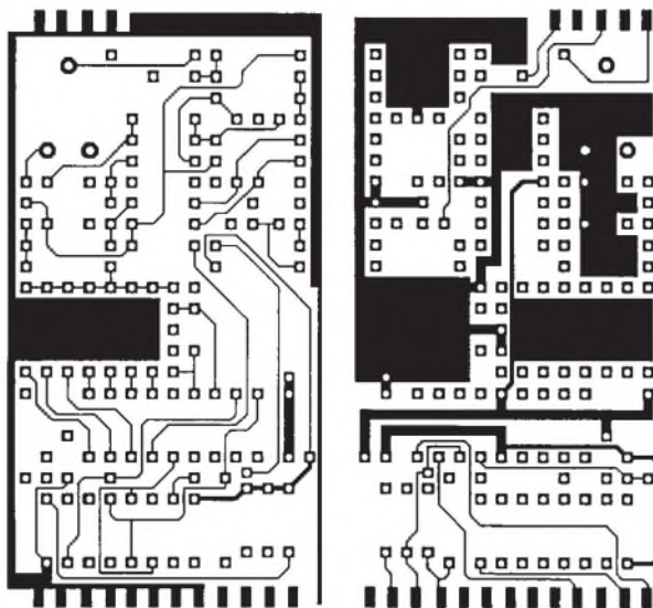
Bild 4: Leitungsführung der PICPAR-Platine (Leitungsseite) Bild 5: Leitungsführung der PICPAR-Platine (Bestückungsseite) Bild 6: Bestückungsplan der Leiterplatte für das PICPAR-Modem
