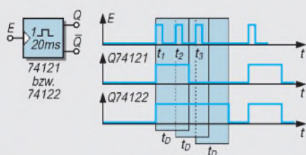
Bild 20: Vergleich der Ausgangssignale beim nicht-nachtriggerbaren 74121 und dem nachtriggerbaren 74122.
