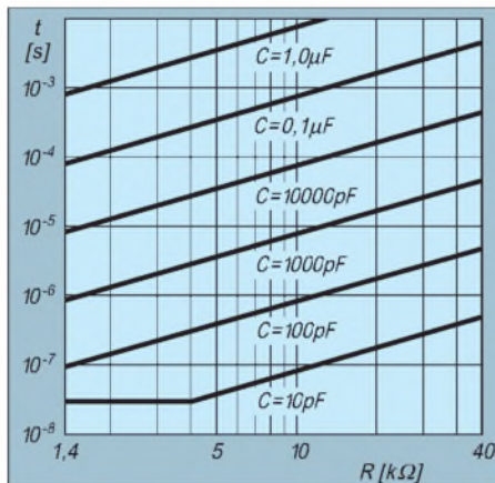
Bild 14: Diagramm zur Festlegung der Werte von R und C für die äußere Beschaltung des Bausteins 74121.
