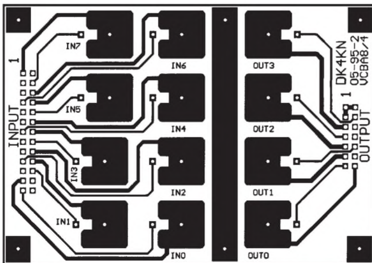
Bild 6: Layout der Verbindungs- platine
