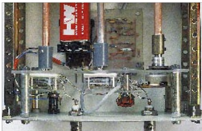
Bild 4: Rückansicht der Meßbrücke mit den Buchsen für das Meßobjekt und den Empfänger
