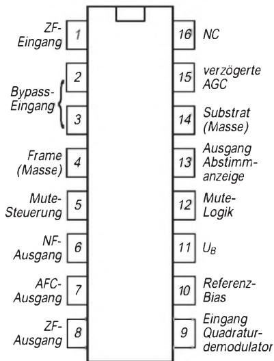
Bild 1: Pinbelegung der 16poligen Gehäuse PDIP und CDIP Bild 2: Pinbelegung beim Gehäuse SOIC
