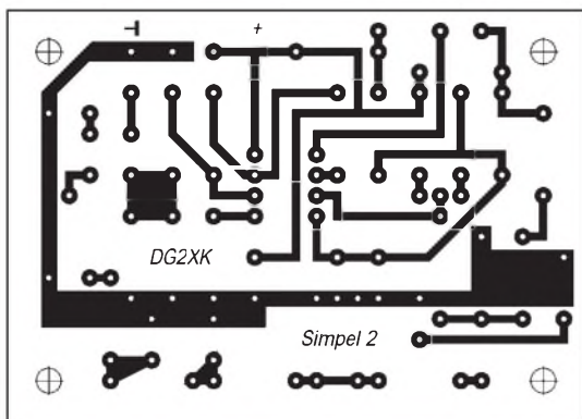
Bild 2: Layout der Platine für das Komparator- Modem „Simpel 2“
