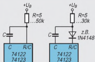
Bild 22: Zwei Fälle der möglichen äußeren Beschaltung bei den Bausteinen 74122 und 74123.
