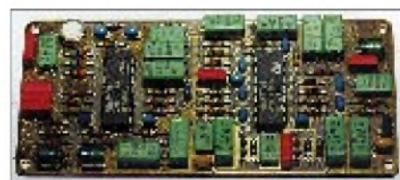
Die Kreationen von HFB-Elektronik stellen immer etwas Besonderes dar. Dieses schmale NF-Filter ist auf einer vergoldeten Platine aufgebaut und sieht super aus.
