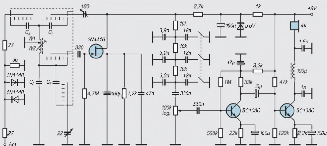
Bild 8: KW-Einkreiser für die Amateurfunkbänder
