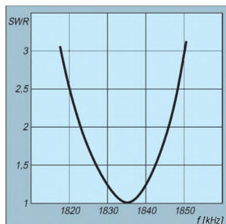
Bild 4: Gemessene Stehwellenkurve der R1. Die Bandbreite für s = 2 beträgt reichlich 20 kHz.
