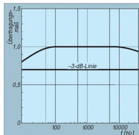
Bild 3: Frequenzgang
