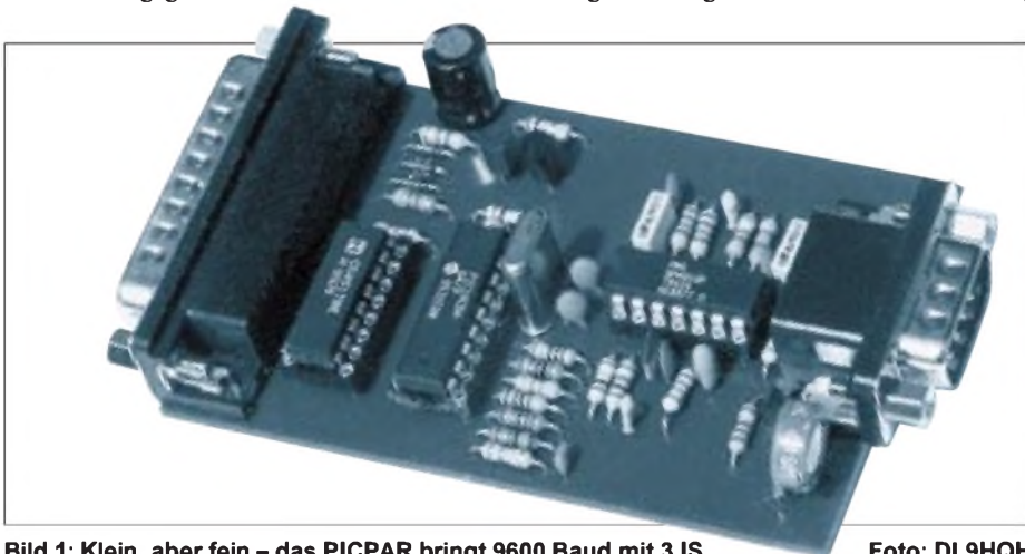
Bild 1: Klein, aber fein – das PICPAR bringt 9600 Baud mit 3 IS.
