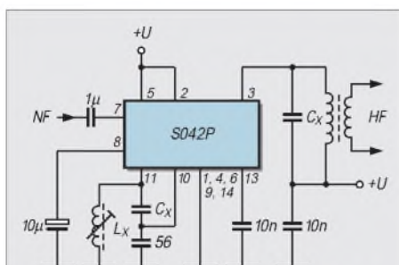
Bild 4: Oszillator mit einer integrierten Schaltung und Zuführung des NF-Signals zur Amplitudenmodulation
