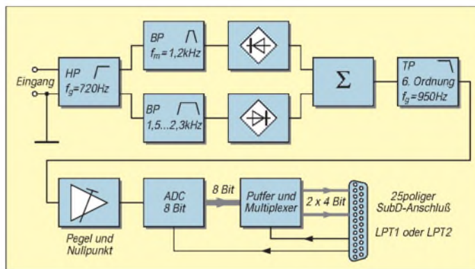
Bild 7: Übersichtsschaltplan vom Empfangsteil des ViewPort-VGA-Konverters.
