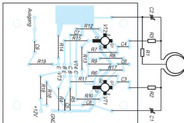
Bild 3: Bestückungsplan der Verstärkerplatine für die Magnetantenne
