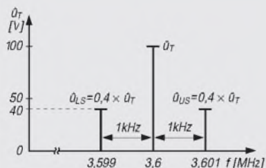
Bild 1: Darstellung des Frequenzspektrums für den Fall, daß bei der Amplitudenmodulation zu Meßzwecken mit nur einer Tonfrequenzschwingung moduliert wurde ( m = 0,8 , f_T = 3,6 MHz, f_{NF} = 1 kHz)
