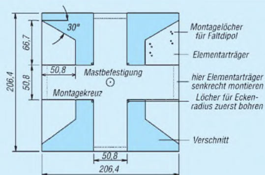
Bild 5: Montagekreuz für eine 70-cm-Lindenblad-Antenne. Plexiglas oder anderes nichtleitendes Material verwenden (etwa 6 mm dick)
