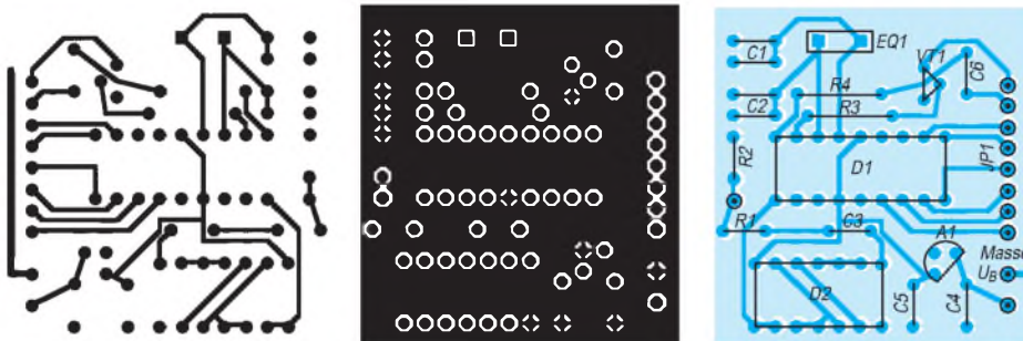
Bild 5: Leitungs-führung der Platine für den Zeitfolge-Eichmarkengeber (Leitungsseite) Bild 6: Durchgehende Bestückungsseite der Platine für den Zeitfolge-Eichmarkengeber mit Freileitungen (Bestückungsseite) Bild 7: Der Bestückungsplan der Leiterplatte des Zeitfolge-Eichmarkengebers enthält noch eine Option für den Elbug-Einsatz.
