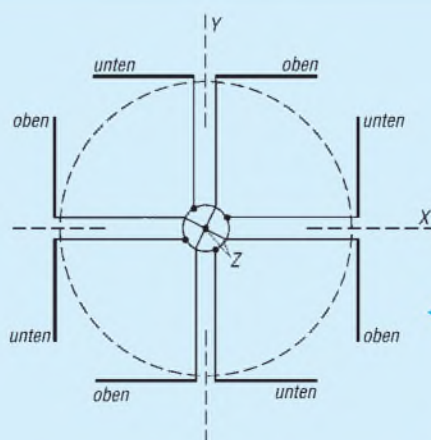
Bild 2: Schematische Darstellung der Speisung der einzelnen Dipole (Draufsicht)
