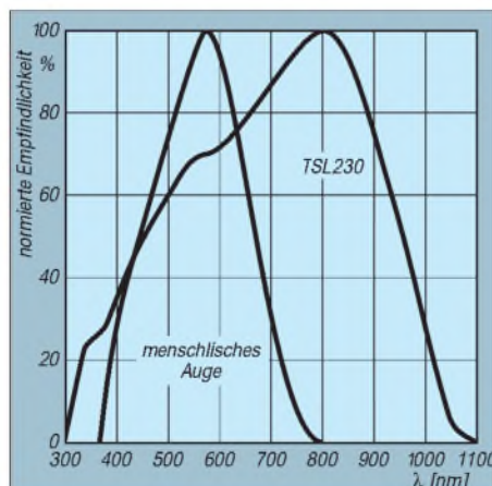
Bild 2: Empfindlichkeitsvergleich
