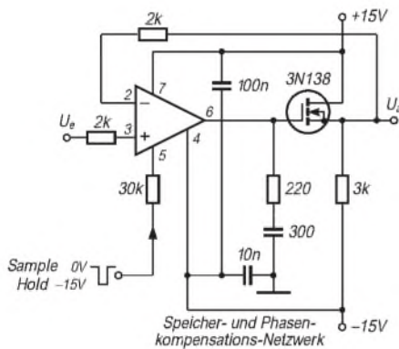
Bild 5: Einfache Sample-and-Hold-Schaltung. Im Sample-Betrieb beträgt die Slew Rate 1,3 V/μs.
