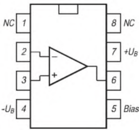
Bild 2: Pinbelegung bei den Inline-Gehäusen
