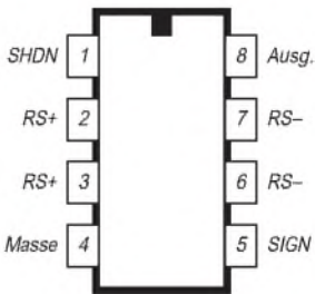
Bild 2: Pinbelegung MAX 471 (MAX 472: Pin 2 NC und Pin 7 UB)
