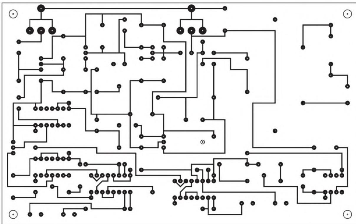
Bild 4: Platinenlayout Leiterseite
