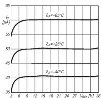
Bild 8: Die Stromaufnahme der Schaltkreise als Funktion der Spannung an Pin 3
