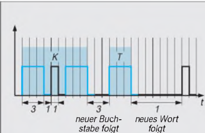
Bild 1: Jedes Element im Morsezeichen besteht aus einzelnen Zeiteinheiten, in denen das Signal den Wert 1 oder 0 hat. Die Pause zum in der Übertragung nächsten Zeichen ist die letzte Zeiteinheit im Zeichen und gehört somit zum Zeichen immer dazu.
