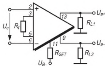
Bild 3: Grundbeschaltung MAX 435
