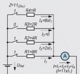
Bild 1: Prinzipschaltung eines 4-Bit-D/A-Wandlers
