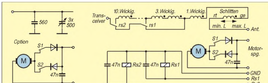
Bild 5: Stromlaufplan der Baugruppe veränderbare Induktivität mit Option veränderbare Kapazität
