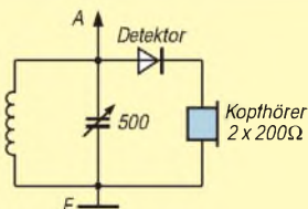
Bild 1: Die Originalschaltung des „Mars-Detektorapparates“
