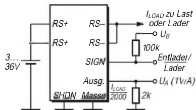
Bild 3: Beim MAX 471 genügen zwei externe Widerstände.
