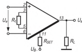
Bild 4: Grundbeschaltung MAX 436
