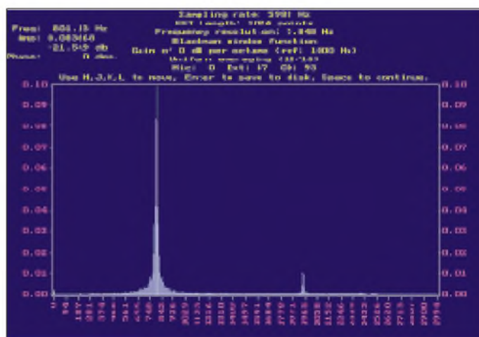
Bild 2: Ungestörtes Amtor-Signal in zweidimensionaler Darstellung
