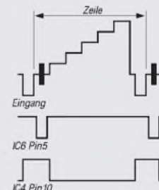
Bild 2: Zeitverhältnisse des Horizontal- synchronimpulses
