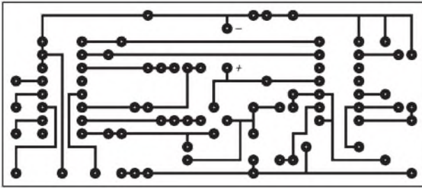
Bild 2: Platinenlayout
