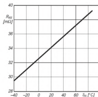
Bild 7: Der intere Fühlerwiderstand ist direkt proportional zur Umgebungstemperatur.
