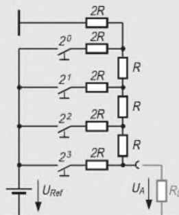
Bild 1: Prinzipschaltung eines 4-Bit-D/A-Wandlers
