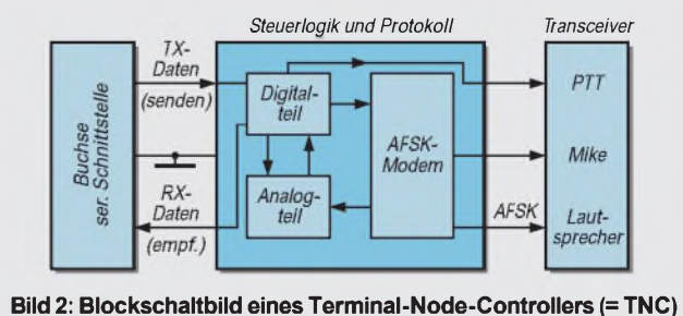
Bild 2: Blockschaubild eines Terminal-Node-Controllers (= TNC)
