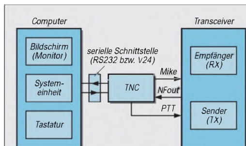
Bild 1: Zum Betrieb von Packet-Radio benutzt man ein TNC oder die im Text erwähnte „Softwarelösung“ (Minimodem, o.ä.), einen Computer und seinen Transceiver bzw. Sender und Empfänger.
