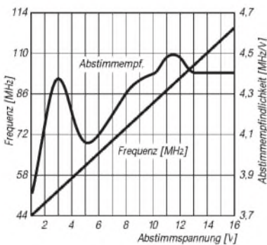
Bild 5: POS-100/JTOS-100-Abstimmcharakteristik; Ausgangsfrequenz und Abstimmungsempfindlichkeit in Abhängigkeit von der Abstimmungsspannung
