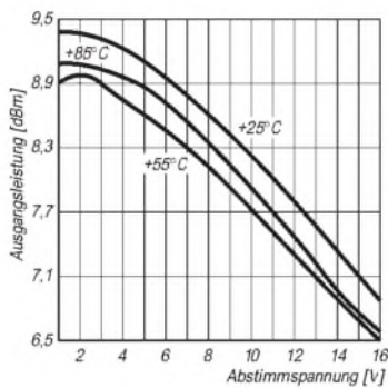
Bild 6: POS-100/JTOS-100-Ausgangsleistung in Abhängigkeit von Abstimmungsspannung und Temperatur
