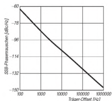
Bild 12: POS-300/JTOS-300-Phasenrauschen in Abhängigkeit vom Träger-Offset bei SSB
