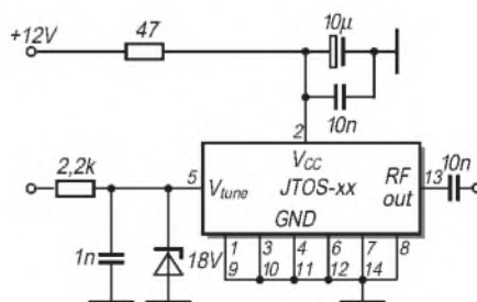
Bild 2: Empfohlene Grundbeschaltung der JTOS-Typen
