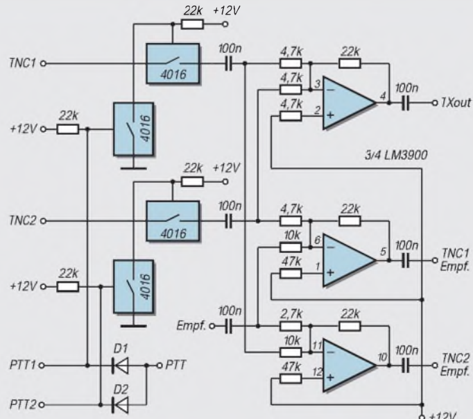
Bild 2: Stromlaufplan des TNC-Kopplers mit Hilfsschalter zur Unterdrückung eines TX-Dauertons
