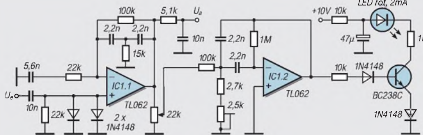
Bild 3: SSTV-Vorfilter mit zusätzlicher Anzeige der 1200-Hz-Synchronimpulse
