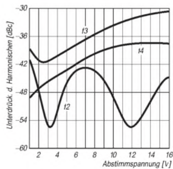
Bild 7: POS-100/JTOS-100-Unterdrückung der Harmonischen f2, f3 und f4 in Abhängigkeit von der Abstimmungsspannung
