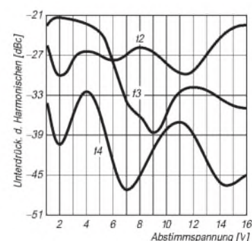
Bild 15: POS-1025/JTOS-1025-Unterdrückung der Harmonischen f2, f3 und f4 in Abhängigkeit von der Abstimmspannung
