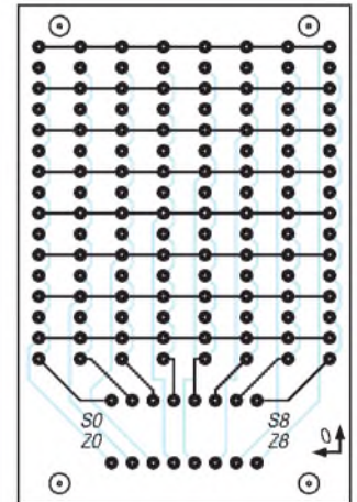
Bild 4: Leiterplatte ANB-5 (Bestückungsseite; für 5 mm LED)
