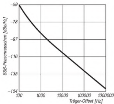
Bild 8: POS-100/JTOS-100-Phasenrauschen in Abhängigkeit vom Träger-Offset bei SSB
