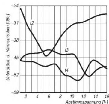
Bild 11: POS-300/JTOS-300-Unterdrückung der Harmonischen f2, f3 und f4 in Abhängigkeit von der Abstimmspannung
