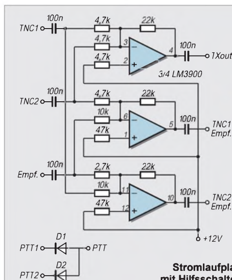
Bild 1: Stromlaufplan des TNC-Kopplers ohne Hilfsschalter
