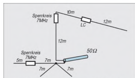
Bild 11: Antennenaufbau beim Verfasser
