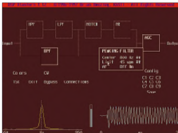
Bild 4: RTTY-Signal mit aktiviertem Bandpaßfilter und Geräuschreduktion
