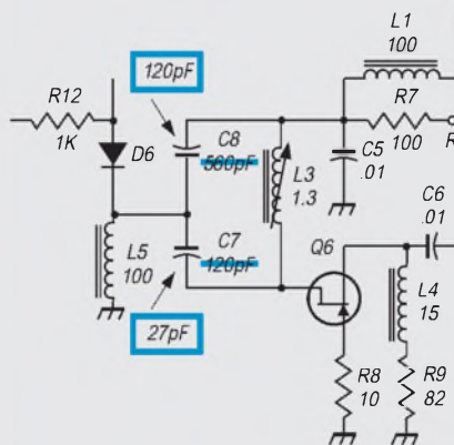
Bild 2: Auszug des Stromlaufplans des 14-MHz-Empfangsverstärkers. C 7 und C 8 sind zu ändern in C 7 = 27 pF, C 8 = 120 pF. L3 ist neu abzugleichen.
