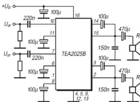
Bild 8: Stereoverstärker mit typisch 45 dB Spannungsverstärkung
