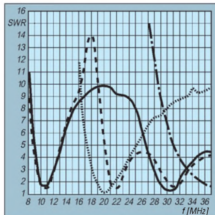
Bild 3: Stehwellenverhältnisse der einzelnen Monopole (Schiebemast, Strichlinie; Aluminiumrohre, Punkt- und Strichpunktlinie) und ihrer Parallelschaltung (ausgezogene Linie) als Funktion der Frequenz
