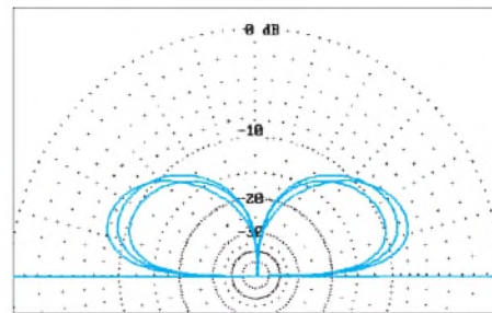
Bild 7: Strahlungsdiagramm der CSCR-Antenne bei 10,5 MHz, 20 MHz und 37 MHz bei schlechterer Bodenleitfähigkeit. Es weist wiederum eine nahezu frequenzunabhängige Kontur auf.
