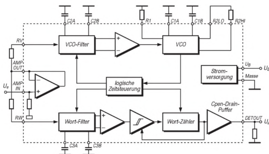
Bild 1: Blockaufbau des Tondekoder-Schaltkreises
