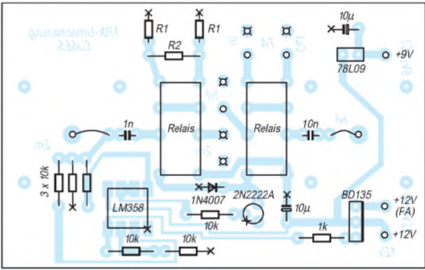
Bild 8: Leitungsführung der Platine für die Sende/Empfangs-Umschaltung
