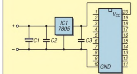
Bild 2: Anschluß der Betriebsspannung incl. Spannungsreglung
