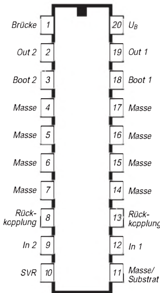
Bild 3: SO-Gehäuse (TEA 2025D)
