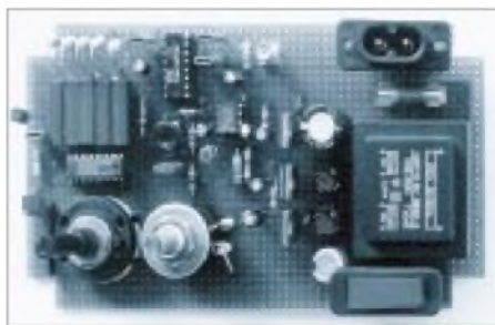
Bild 4: Musteraufbau
