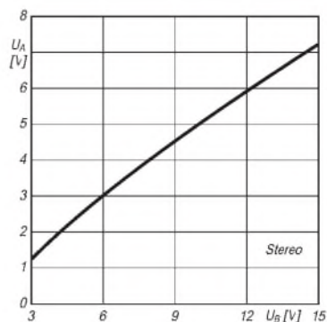
Bild 5: Ausgangsgleichspannung und Betriebsspannung
