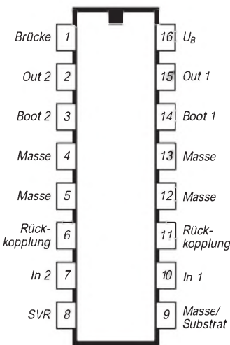
Bild 2: Power-DIP (TEA 2025B)
