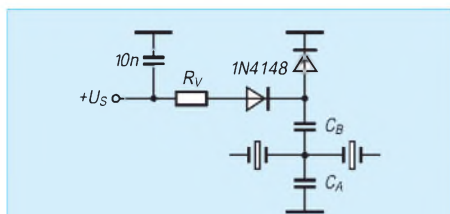
Bild 4: Prinzip einer Bandbreitenumschaltung mit Hilfe der Abzweigkondensatoren C1 bis C5. C A bestimmt die größere Bandbreite, C B wird zur Verringerung der Bandbreite parallelgeschaltet. Die Kapazitäten addieren sich dabei.
