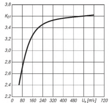
Bild 3: Der Abfallzeit proportionaler Faktor K_{OT} über der Eingangsamplitude mit Diode zwischen Pin 5 und 6
