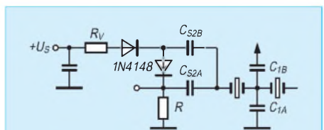
Bild 5: Prinzip einer Bandbreitenumschaltung mit Hilfe der Serienkondensatoren C s . C s2A wird C s2B parallelgeschaltet. R V und R ergeben eine Reihenschaltung, der Richtwert des Gesamtwiderstands ist bei U s = 12 V 3,3 kΩ. Bei der Umschaltung eines anderen Serienkondensators wird R durch eine Drossel ersetzt.
