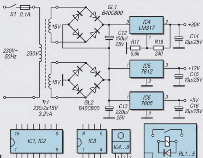
Bild 3: Stromversorgung
