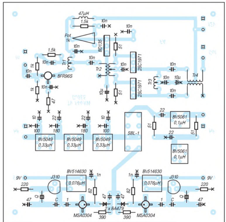
Bild 5: Bestückungs- plan der Leiterplatte für den Transverter mit Sende- endstufe. Alle per Kreuz markierten Anschlüsse werden einfach auf der Bestückungs- seite mit Masse verlötet.
