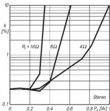
Bild 7: Klirrfaktor über der Ausgangsleistung
