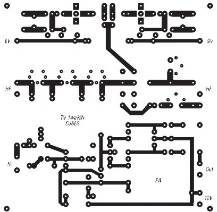
Bild 4: Leitungs- führung der Platine für den Trans- verter mit Sende- endstufe. Die Rückseite der Platine ist durchgehend kaschiert (Massefläche). Die Bohrungen sind frei- zusenken.
