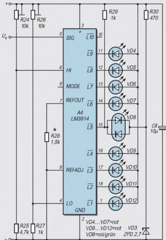
Bild 2: Stromlaufplan der LED-Skala (LM3914)
