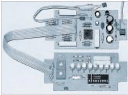
Bild 10: Musteraufbau der Schaltung mit LM3914
