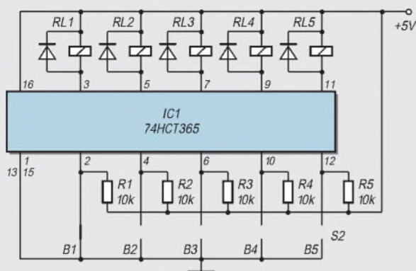
Bild 2: Die Bereichsumschaltung erfolgt über Relais.
