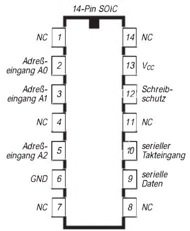
Bild 2: Anschlußbelegung
