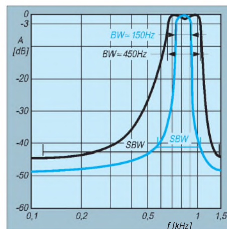
Bild 7: Filterkurven des CW-Filters bei den Programmierungen 150 Hz und 450 Hz, f_0 = 800 Hz
