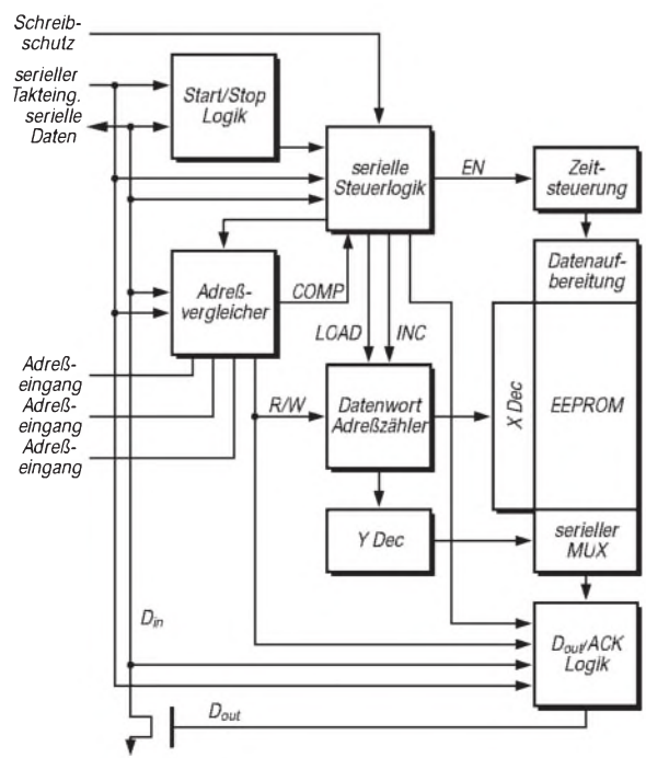
Bild 1: Blockschaltbild des EEPROMs
