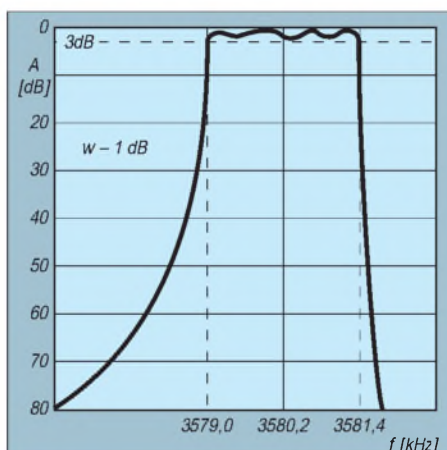
Bild 6: Ungefährer Verlauf der Durchlaßkurve mit 3579,545-kHz-Quarzen; n = 8 ; B \approx 2,4 kHz
