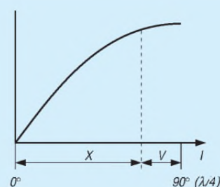
Bild 5: Um das Stück X verkürzt sich die kapazitiv belastete \lambda/4 -Leitung
