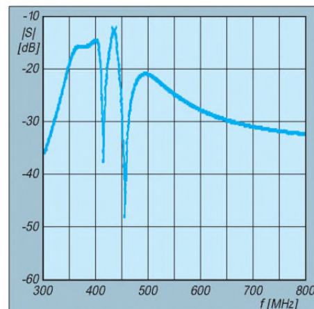
Bild 9: Berechnete Durchlaßkurve eines UHF-Eingangsteils mit vorgeschalteten Saugkreisen. Marke: 435 MHz, f_u = 415 MHz, f_o = 455 MHz
