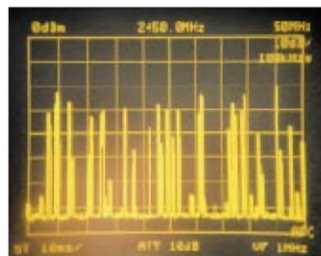
Bild 7: Spektrum eines Frequenzhopping-Signals
