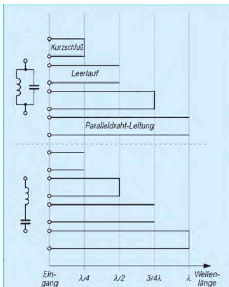
Bild 4: Skizze mehrerer (durch parallele Striche dargestellte) Paralleldrahtleitungen mit einer Länge einer Viertelwellenlänge sowie Leitungen, deren Länge ganze Vielfache einer Viertelwellenlänge lang sind. Die skizzierten Paralleldrahtleitungen sind abwechselnd an ihrem Leitungsende kurzgeschlossen oder leerlaufend. Sie weisen dementsprechend an ihrem Leitungseingang entweder Parallelresonanzverhalten oder Serienresonanzverhalten auf.
