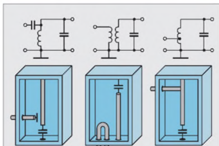
Bild 12: Die Ein- und Auskopplung der Hochfrequenz kann in Rohr- und Topfkreisen induktiv oder kapazitiv erfolgen. Das Bild zeigt Skizzen von Schnitten einiger typischer Anordnungen von Koppelschleifen, die in den Topf einzubauen sind. Die jeweils über die Anordnung gezeichnete Schaltung zeigt den Vergleich zu üblichen Schaltungen aus den Hochfrequenzbereichen.
