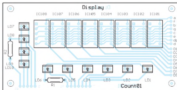
Bild 7: Bestückung der Platine „Display“
