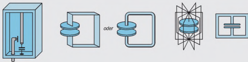
Bild 8: In der Anfangszeit der Fernsehuner wurden die Leitungskreise oft durch Drahtbügel in Abschirmkammern oder auf Leiterplatten realisiert und durch Plattendrehkondensatoren oder -trimmer an ihrem Eingang auf die gewünschte Resonanzfrequenz abgestimmt.
