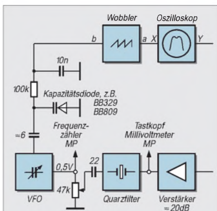
Bild 8: Prinzip der Wobbelung. Man beachte, daß das Quarzfilter dabei mit den richtigen Widerstandswerten abzuschließen ist.
