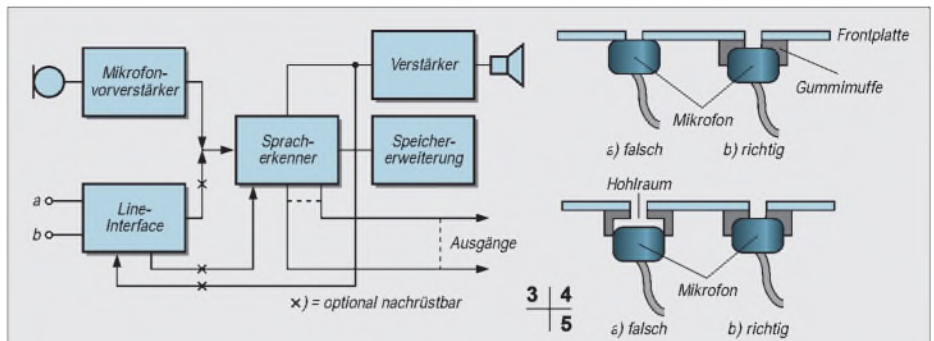
Bild 3: Das Blockschaltbild unserer Spracherkennerbaugruppe
