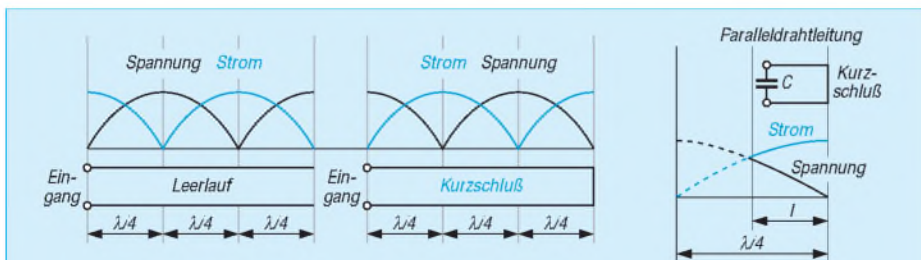
Bild 5: Einige der im Bild 4 gezeigten Paralleldrahtleitungen mit den zugehörigen Strom- und Spannungscurven: Am Kurzschluß tritt selbstverständlich immer ein Strommaximum auf, und die Spannung hat den Wert Null. Am Leerlauf dagegen herrscht ein Spannungsmaximum, und der Strom hat den Wert Null.
