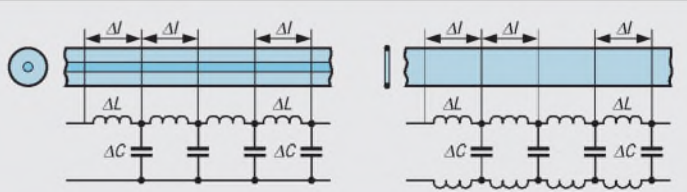
Bild 2: Skizze einer Koaxialdrahtleitung und einer Paralleldrahtleitung
