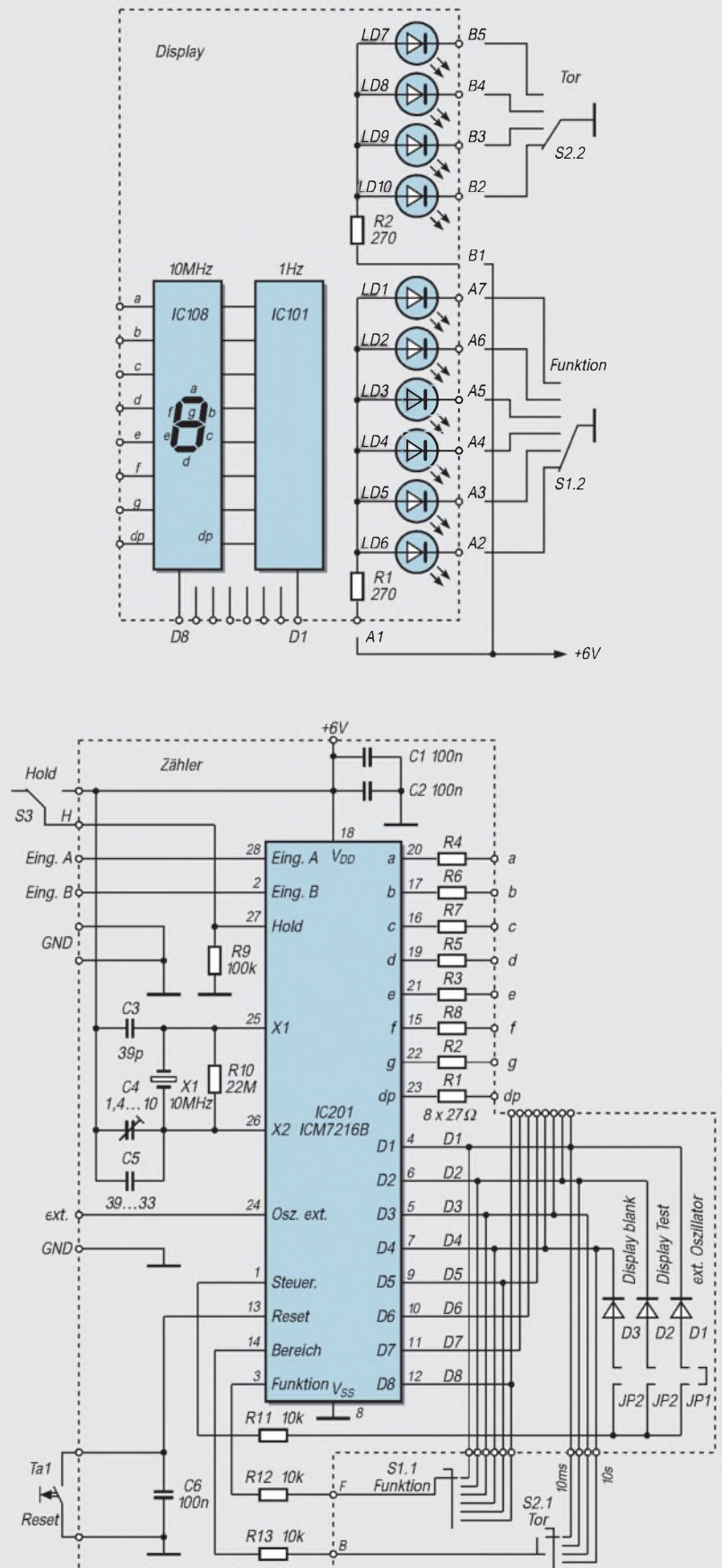
Bild 3: Grundbaustein des modularen Zählers
