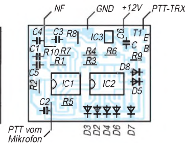
Bild 4: Leitungsführung der SMD-Platine für die Roger-K-Baugruppe zum Einbau in das Mikrofon des IC-820H
