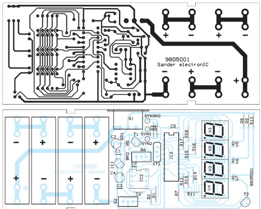
Bild 2: Die Platine besitzt zwei Einkerbungen für das Gehäuse.
