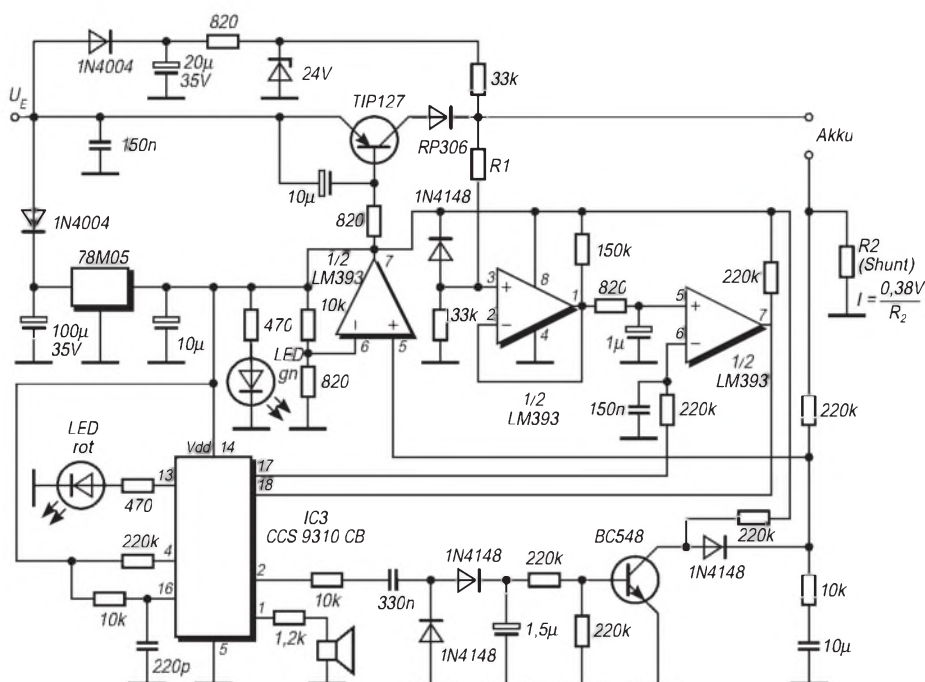
Bild 3: Anwendungsschaltung des Herstellers. Die Schaltung muß über einen Vollweggleichrichter ohne Glättungskondensator versorgt werden; U_E ist somit eine 100-Hz-Sinushalbwellen-Spannung. Der Ladestrom I sollte C/h betragen, bei einem 600-mAh-Akku also 600 mA. Er ergibt sich aus R_2 und der Referenzspannung 0,38 V nach der angegebenen Formel.
