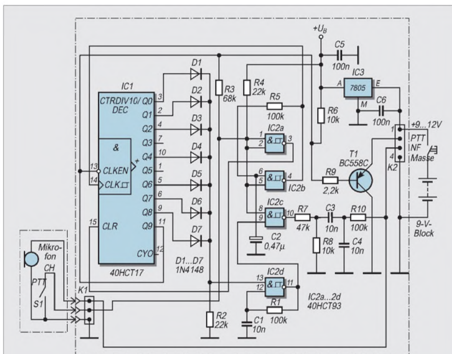
Bild 1: Stromlaufplan der Roger-K-Baugruppe
