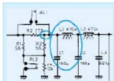
Bild 5: Überbrückung des Preselektors
