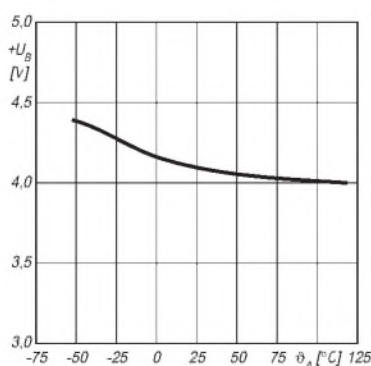
Bild 3: Minimale Betriebsspannung
