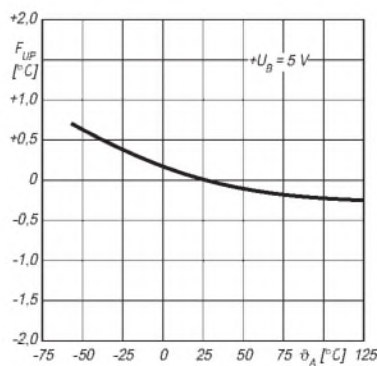
Bild 4: Typischer Linearitätsfehler
