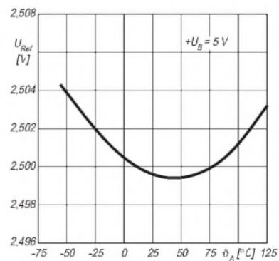
Bild 5: Referenzspannungsverlauf
