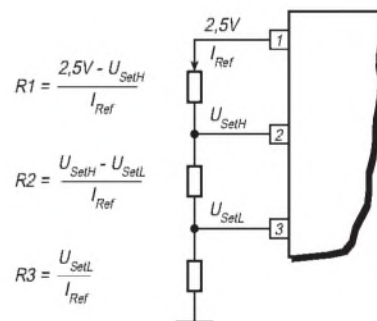
Bild 2: Schaltschwellenfestlegung
