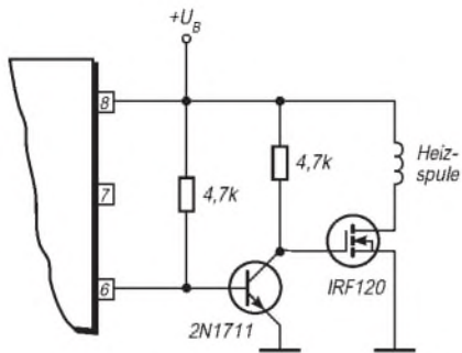
Bild 6: Bipolartransistor und Power-MOSFET für hohen Laststrom
