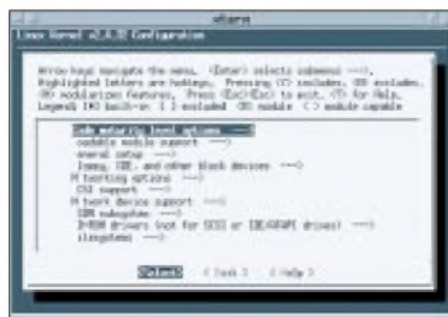
Bild 9: Menüauswahl der Kernelkonfiguration
