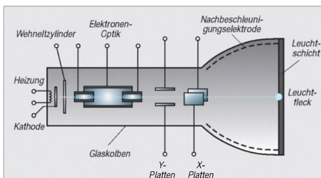
Bild 1: Schematische Darstellung der Elektronenstrahlröhre eines Oszilloskops.
