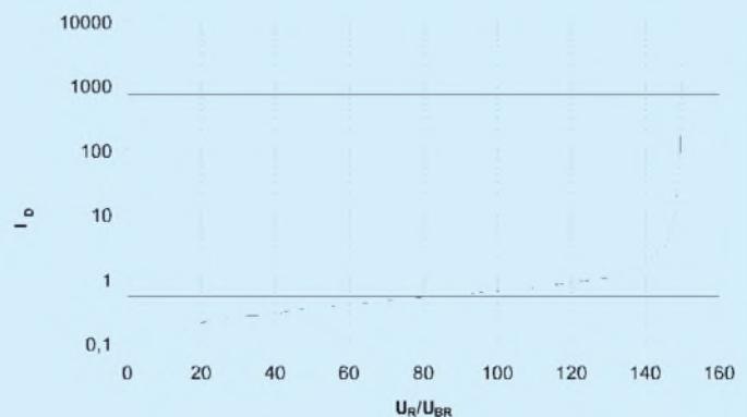
Bild 5: Der Dunkelstrom steigt mit zunehmender Sperrspannung.
