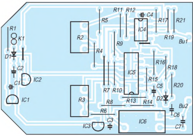
Bild 4: Bestückungsplan
