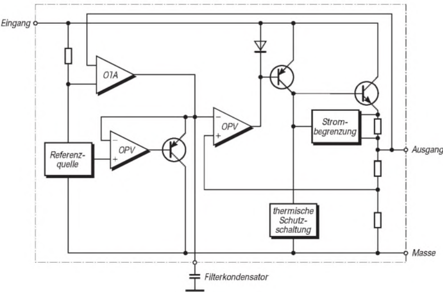
Bild 2: Innenaufbau (Filterkondensator 10...47 µF)
