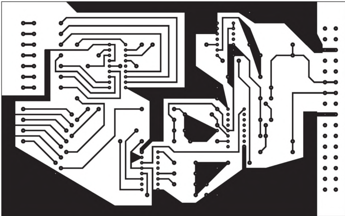
Bild 4: Platinenlayout
