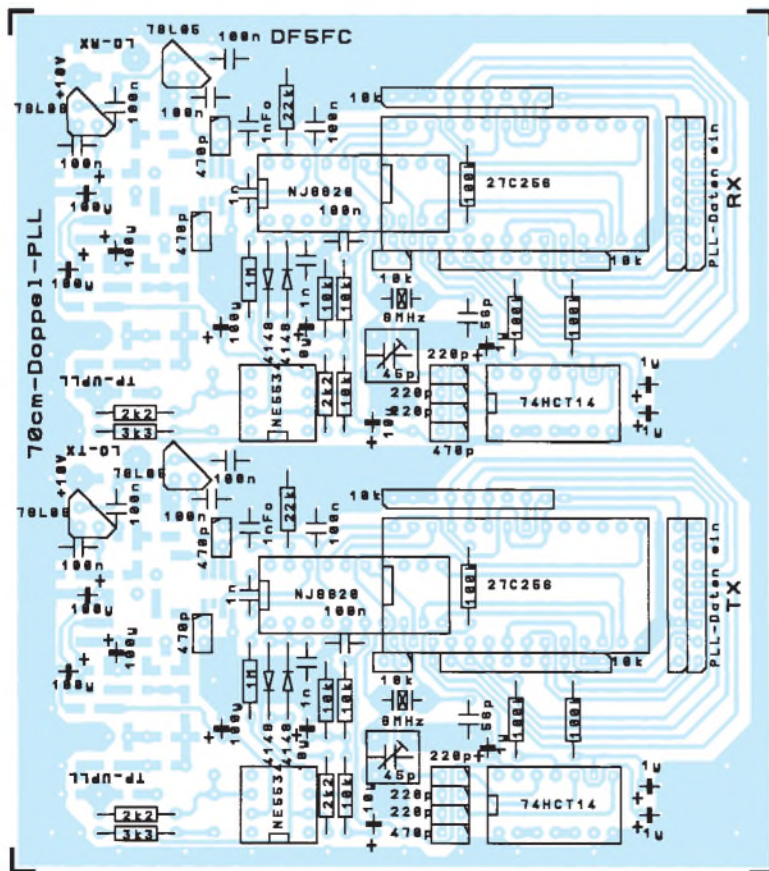
Bild 12: Bestückungsplan der Leiterplatte für die beiden PLLs (Sender und Empfänger)
