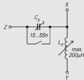
Bild 3: Variables Anpassglied für T-Antennen
