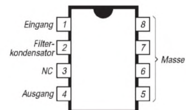
Bild 1: Pinbelegung
