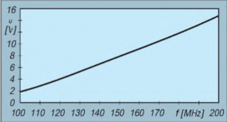
Bild 2: Frequenz/Eingangsspannungskennlinie des eingesetzten VCOs
