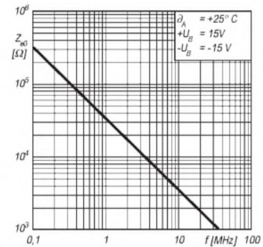
Bild 8: Eingangsimpedanz als Funktion der Frequenz
