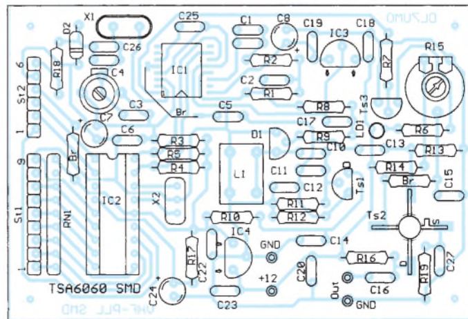
Bild 6: Bestückungsplan der PLL-Leiterplatte (SMD-IC-Variante)
