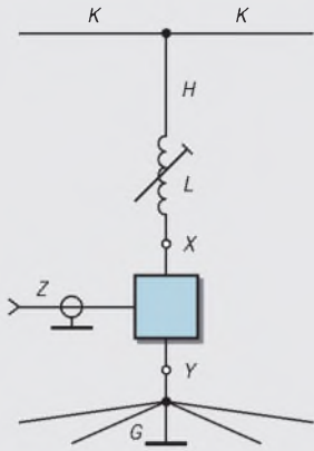
Bild 2: Grund- sätzlicher Aufbau einer T-Antenne
