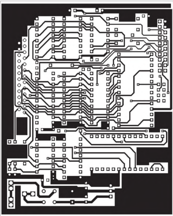
Bild 4 a: Lötseite
