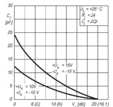
Bild 11: Dimensionierungsempfehlung für den Kompensationskondensator
