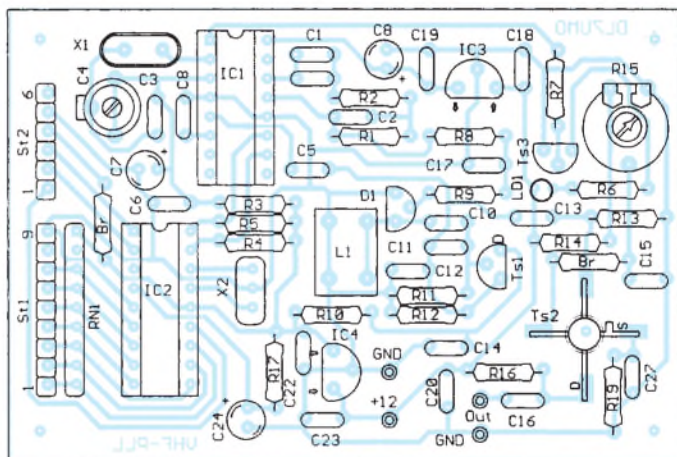
Bild 4: Bestückungsplan der PLL-Leiterplatte (DIL-IC-Variante)
