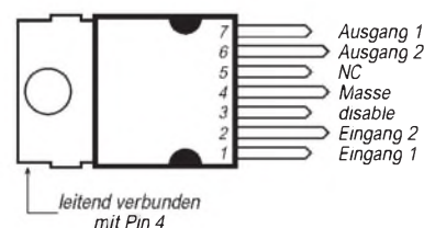
Bild 2: Pinbelegung des siebenpoligen Gehäuses mit Kühlfahne
