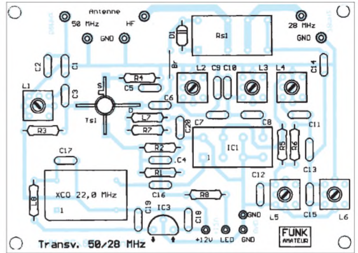
Bild 3: Leitungsführung der Leiterplatte für den Empfangskonverter. Der BF 981 ist hier auf der Oberseite sichtbar, wird aber auf der Unterseite in das Loch eingesetzt und flach auf die quadratischen Lötäugen gelötet.
