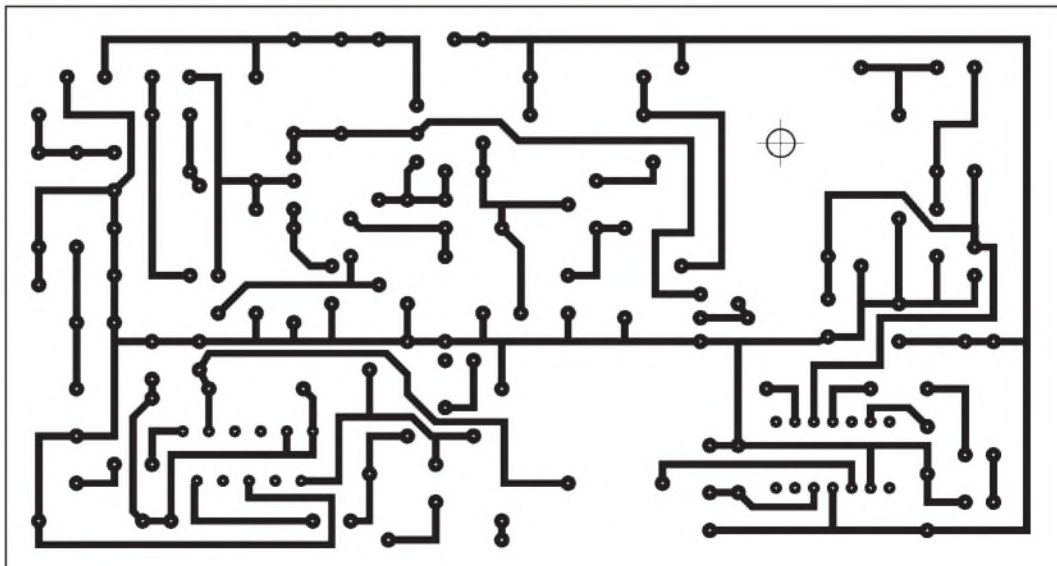
Bild 2: Platinenlayout
