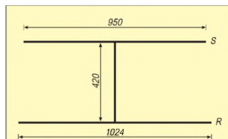
Bild 3: Abmessungen der 2-Element-Yagi (eine Ebene)
