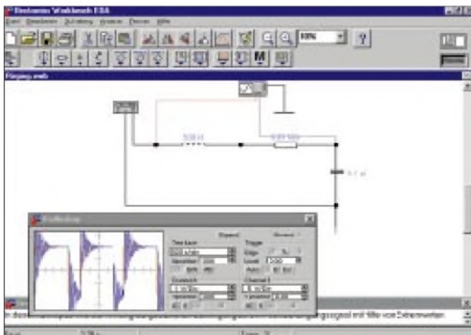
Bild 1: Mit EWB hat man ein komplettes Elektroniklabor auf dem PC, mit dem sich z.B. die elektrischen Schwingungsvorgänge bei Beaufschlagung eines Bandpasses (Extremwerte!!) mit einem Rechtecksignal untersuchen lassen.
