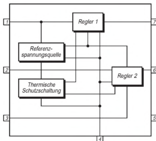
Bild 1: Da die Referenzspannungsquelle über Pin 1 versorgt wird, kann Regler 2 nicht arbeiten, wenn dort keine ausreichende Spannung anliegt.
