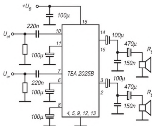
Bild 9: Stereoschaltung; auch hier kann die Verstärkung jedes Kanals mit einem Widerstand zwischen Pin 6 bzw. 11 und dem Kondensator verringert bzw. korrigiert werden.
