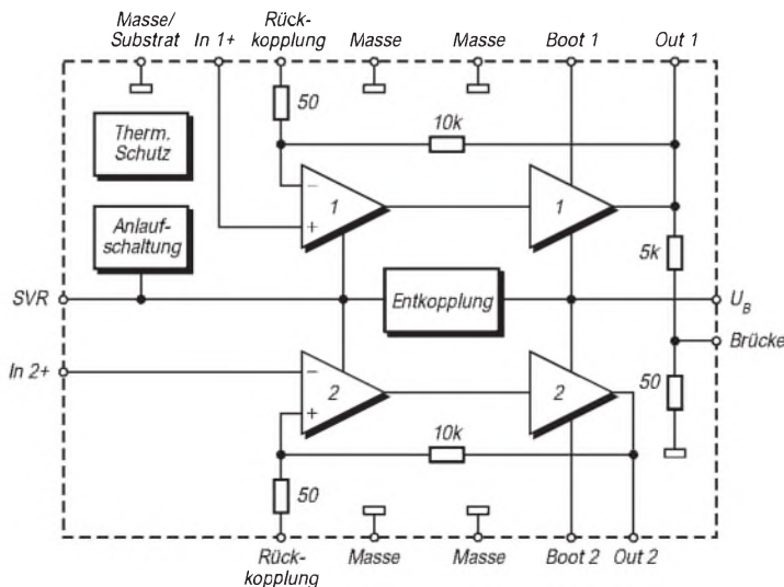
Bild 1: Die internen Funktionsgruppen
