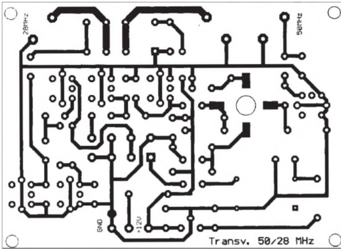
Bild 2: Leitungsführung der Platine für den Empfangskonverter. Die Bestückungsseite ist eine durchgehende Kupferfläche, auf der die Bohrungen für nicht mit Masse verbundene Bauelemente anzusenken sind. Die Bohrlöcher der Lötäugen wurden generell einheitlich angelegt.
