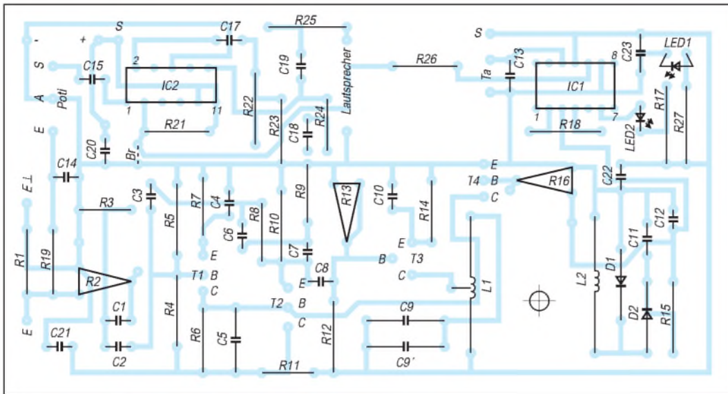
Bild 3: Bestückungsplan
