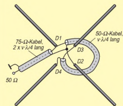
Bild 4: Schema der Zusammenschaltung von Phasen- und Anpaßleitung bei der 2-Element-Yagi
