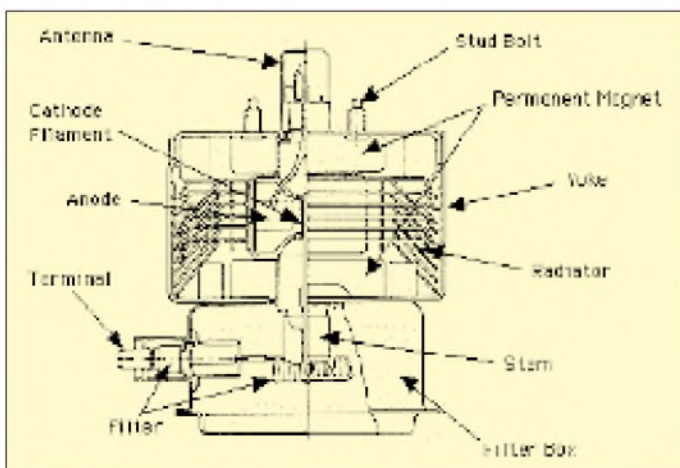
Bild 1: Das Magnetron ist das Herzstück von Mikrowellenherden.
