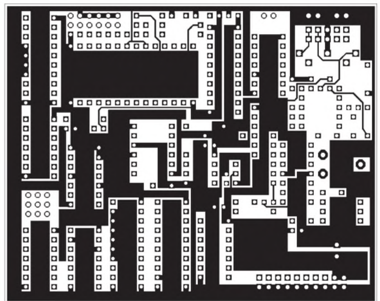
Bilder 5 bis 7: Leitungsführung der Platine (Leitungsseite, oben, und Bestückungsseite) sowie Bestückungsplan der Leiterplatte des DF91C-Modems
