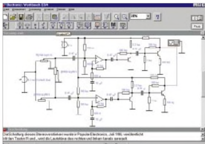
Bild 4: Die Simulation umfangreicher Schaltungen, wie z.B. eines Stereoverstärkers, erfordert für schnelle Ergebnisse oder bei Änderung der Parameter während der Simulation einen schnellen Rechner der Pentium-Klasse.
