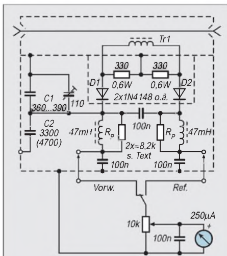
Stromlaufplan des LW-Stehwellenmessers. Für C1 ist ein Styroflex- oder Glimmerkondensator für 400/630 V ~ empfehlenswert, für C2 ein Wima FKC2 für 63 V. Für D1 und D2 eignen sich 1 N 4148, HPA 2800, AA 117, AA 118 o.ä. Für Tr1 wurde ein Ringkern Amidon FT 50B-77 mit 60 Wdg. CuL eingesetzt.
