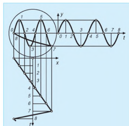
Bild 2: Zeichnerische Konstruktion der auf dem Bildschirm entstehenden Abbildung für die im Bild 1 an den Verstärkern des Oszilloskops anliegenden Spannungen. Die dünnen Konstruktionshilfslinien zeigen, für gleich weite Zeitspannen numeriert, die Lage des Leuchtflecks zu diesen Zeiten auf dem Bildschirm.
