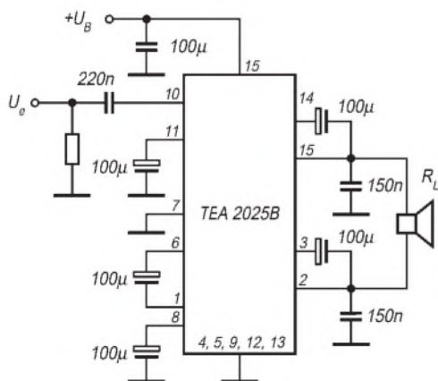
Bild 8: Brückenschaltung; über zusätzliche niederohmige Einstellwiderstände zwischen Pin 6 bzw. 11 und dem Kondensator kann man die internen Verstärkungen für geringsten Klirrfaktor angleichen.
