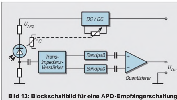
Bild 13: Blockschaltbild für eine APD-Empfängerschaltung
