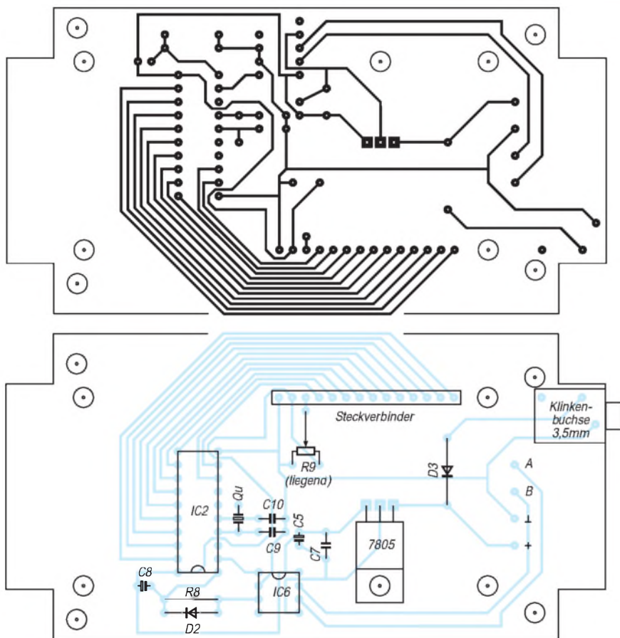
Bild 5: Platinenlayout des Empfangsteils
