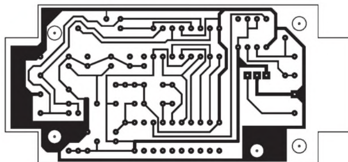
Bild 2: Platinenlayout des Sendeteils
