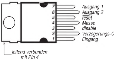
Bild 2: Pinbelegung des siebenpoligen Gehäuses mit Kühlfahne
