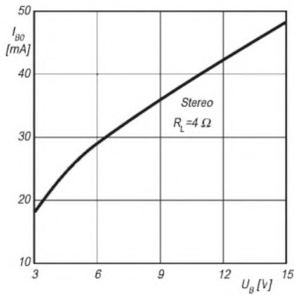
Bild 4: Der Ruhestrom hat bei jeder Betriebsspannung einen verhältnismäßig hohen Wert.
