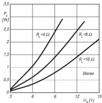
Bild 6: Die Ausgangsleistung bei 10 % Klirrfaktor und 1 kHz als Funktion der Betriebsspannung
