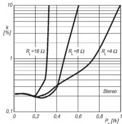
Bild 7: Verlauf des Klirrfaktors über der Ausgangsleistung bei 6 V Betriebsspannung und 1 kHz
