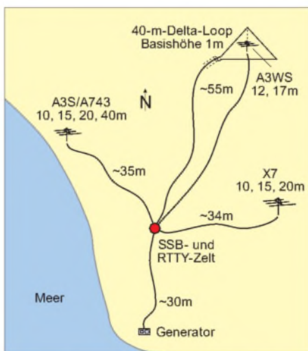
Antennenkarte des SSB-Stationsaufbaus
