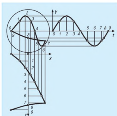
Bild 4: Das Bild zeigt, wie wichtig der – im Beitrag immer wieder angesprochene – zeitlineare Verlauf der Ablenkspannung auf der X-Seite ist. Die hier nicht linear ansteigende Ablenkspannung verzerrt die Darstellung der Meßkurve auf dem Bildschirm extrem stark. Um das hervorzuheben, wurde hier mit einer (statt zwei wie im Bild 2) Periode der Meßspannung gearbeitet.
