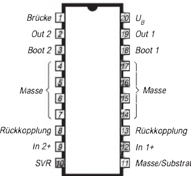
Bild 3: Anschlußbelegung des SMD-Gehäuses SO 20
