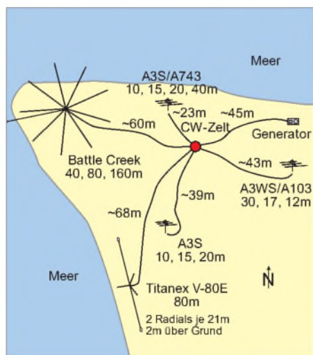
Antennenkarte des CW-Stationsaufbaus
