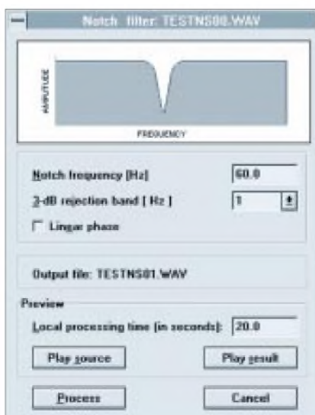
Bild 6: Einzelfilter-Funktion
