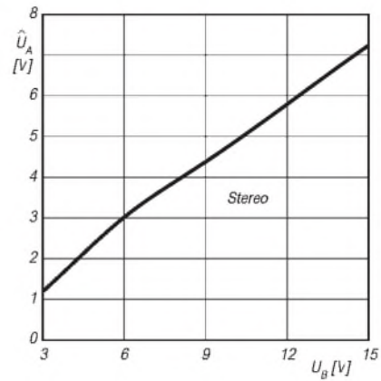
Bild 5: Im Betriebsspannungsbereich 6 ... 9 V kann der Schaltkreis am besten angesteuert werden.
