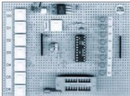
Bild 1: Taster und LEDs/Nachbau des Originals
