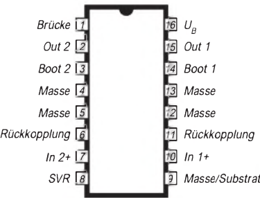
Bild 2: Anschlußbelegung des Powerdip-Gehäuses
