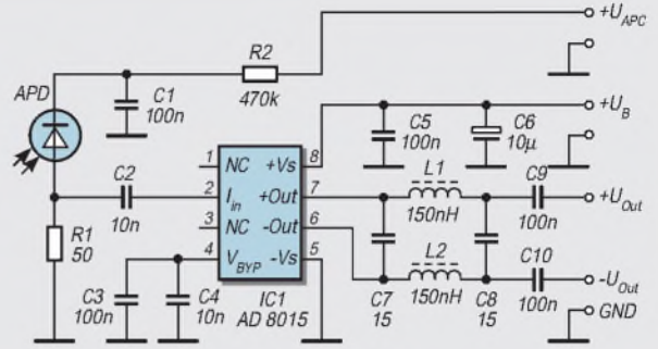
Bild 14: Zur Verstärkung des ADP- Signals wird der AD- Schaltkreis AD8015 verwendet.
